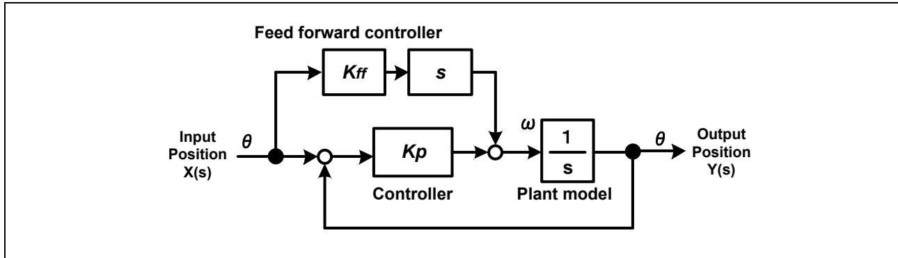
図 6-6 位置制御系のモデル
