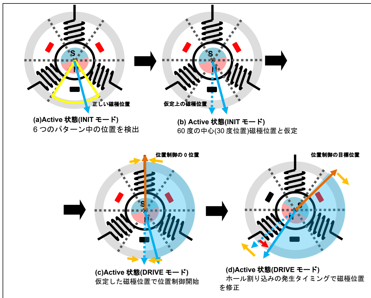
図 5-17 永久磁石の磁極位置の決定手順
