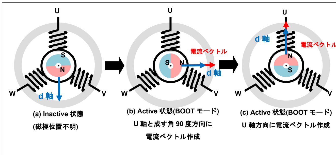
図 5-15 永久磁石位置の決定
