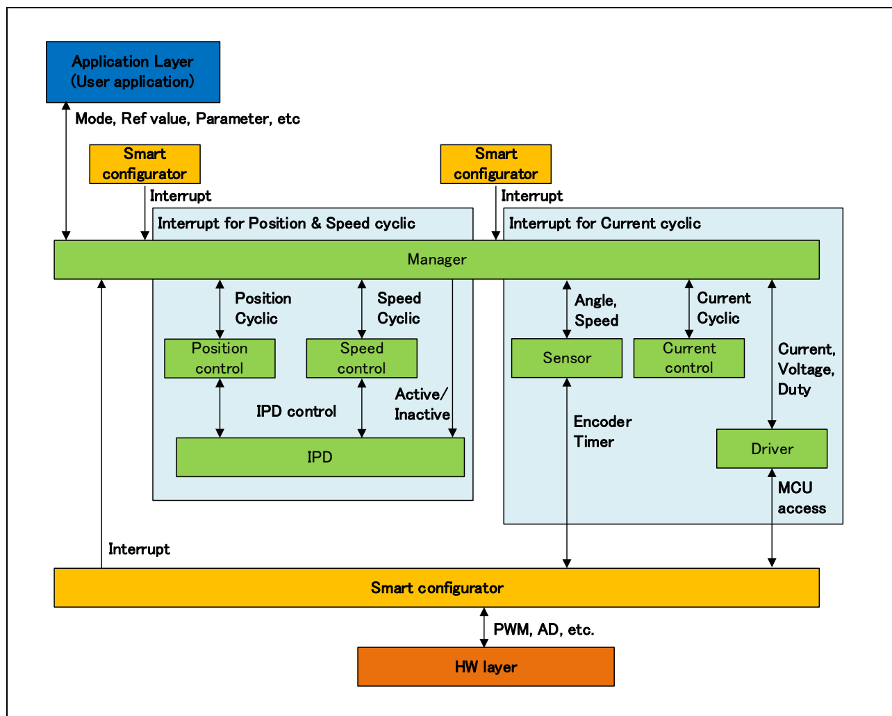
図 4-2 モータモジュールの構成
