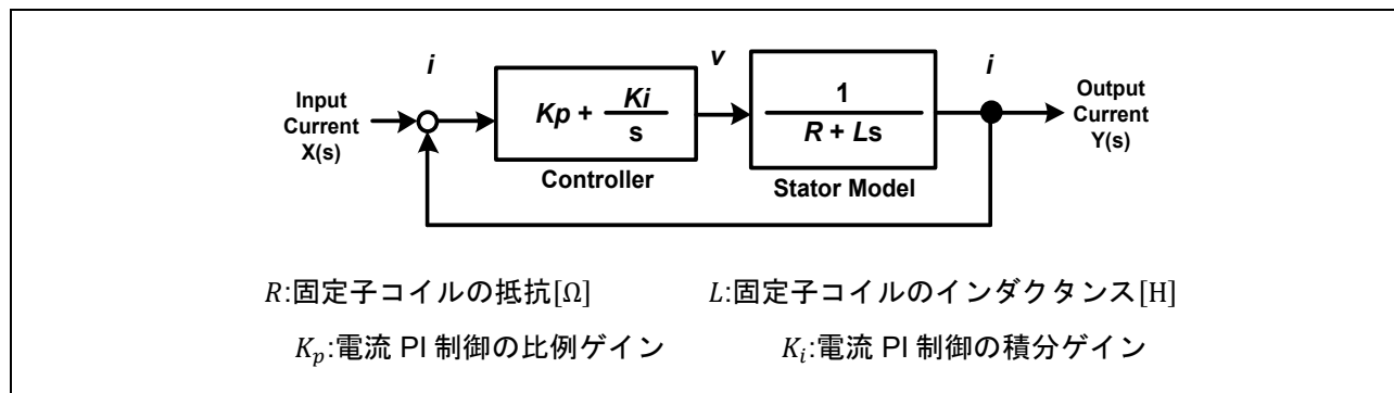
図 6-4 電流制御系のモデル
