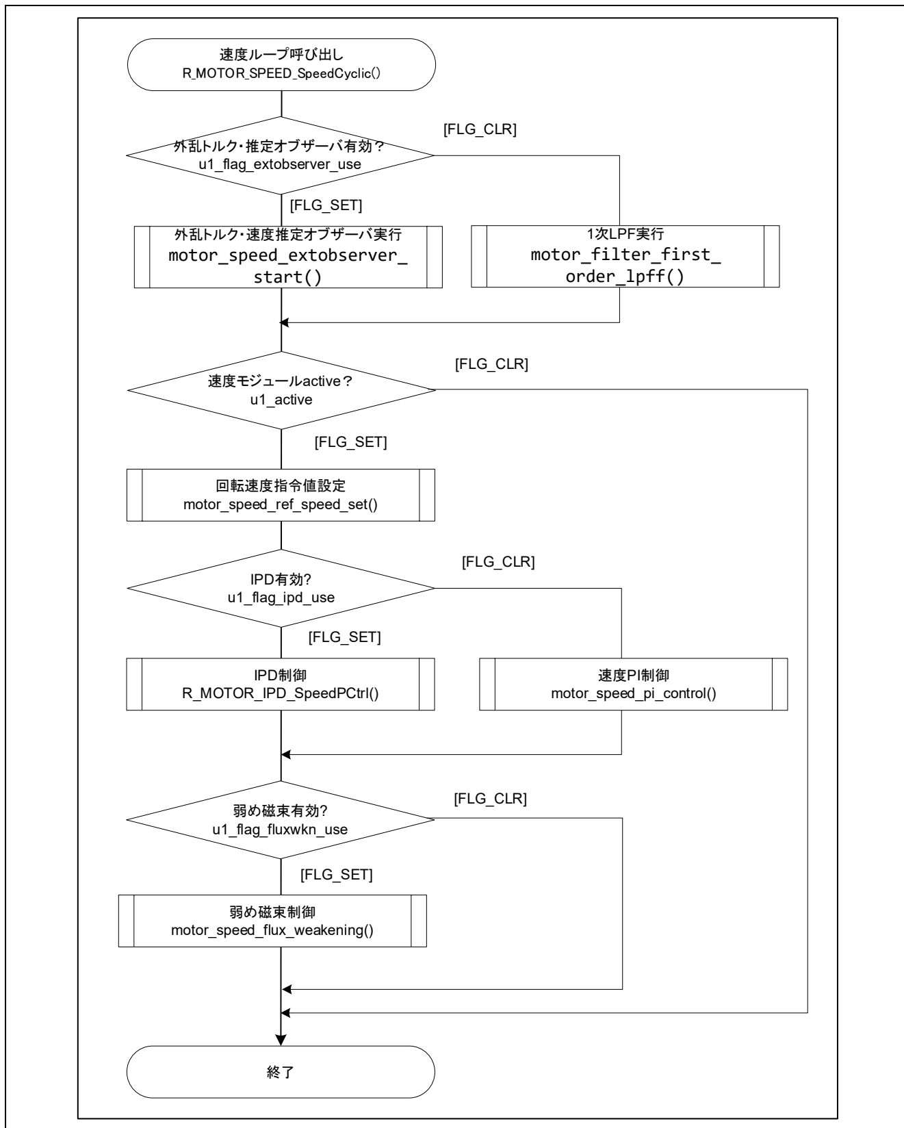
図 5-23 速度制御フローチャート
