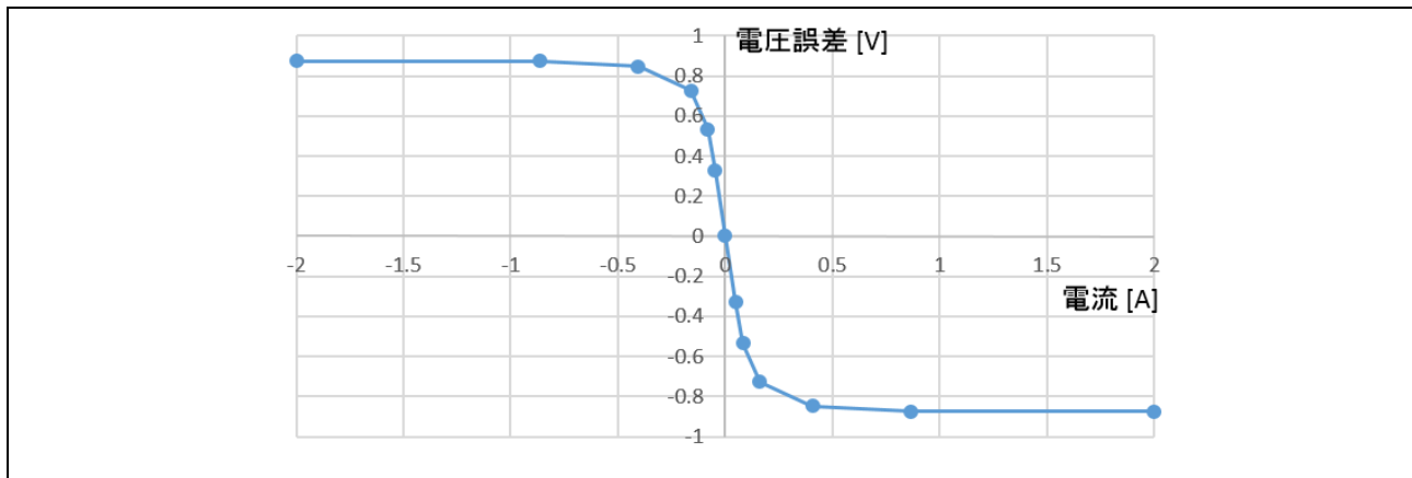
図 5-21 電圧誤差の電流依存性(一例)
