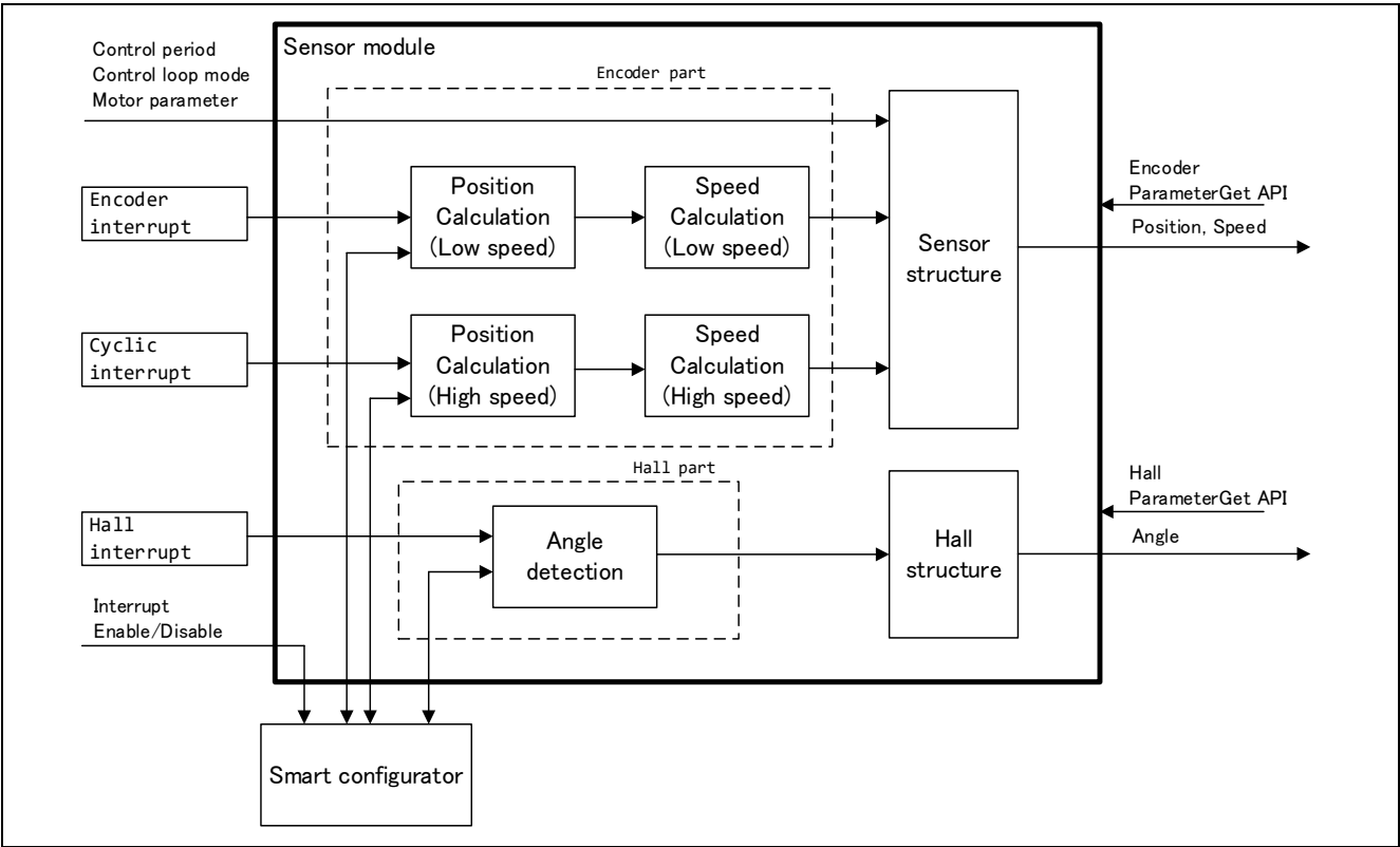
図 5-32 センサモジュール構成図
