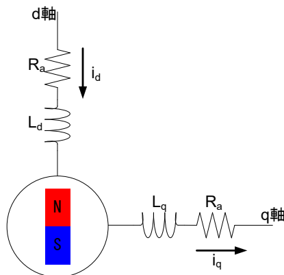
図 6-2 2 相直流モータの概念図
