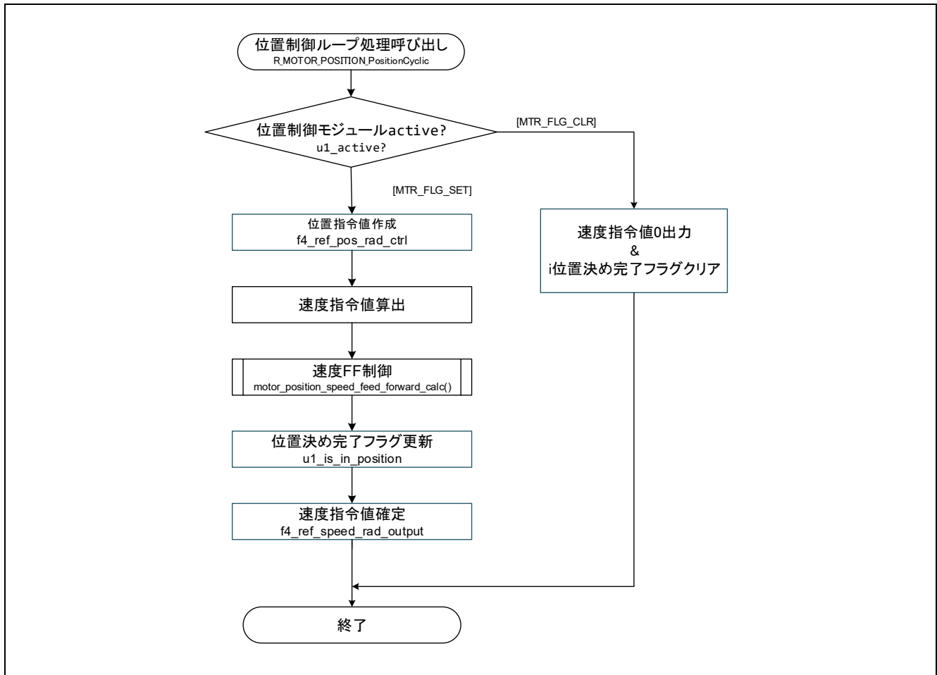
図 5-27 位置制御ループ処理フローチャート
