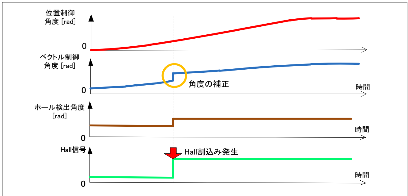
図 5-18 ホール使用初期位置検出における始動シーケンス
