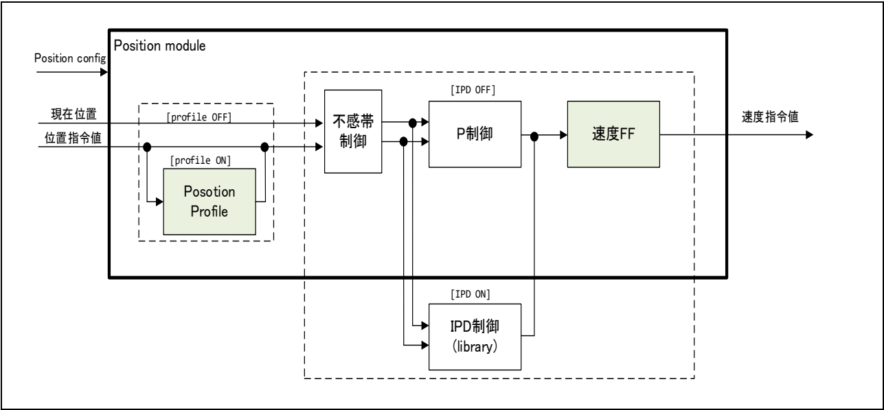
図 5-26 位置制御モジュール構成図
