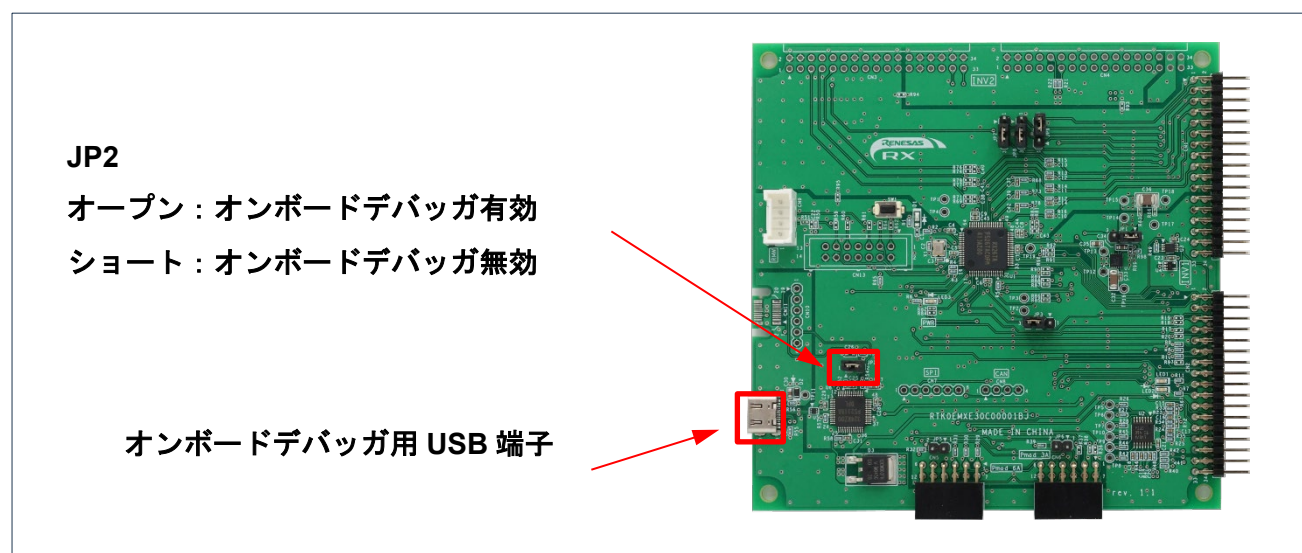
図 2-6 オンボードデバッグ(RX26T RAM48KB バージョン)
