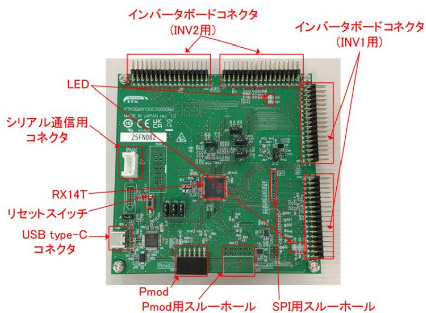
図 2-4 RX14T CPU ボードとインタフェース
