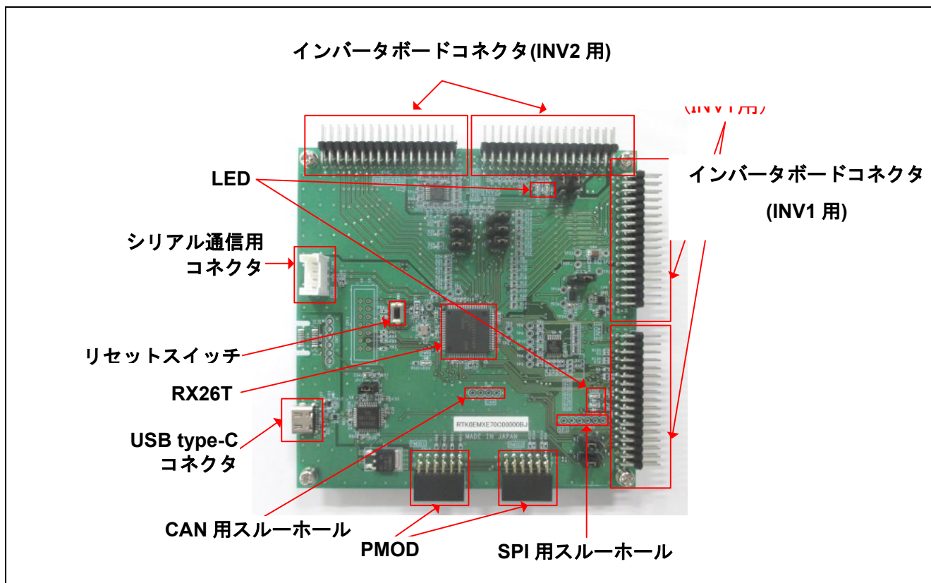
図 2-2 RX26T RAM64KB バージョン CPU ボードとインタフェース
