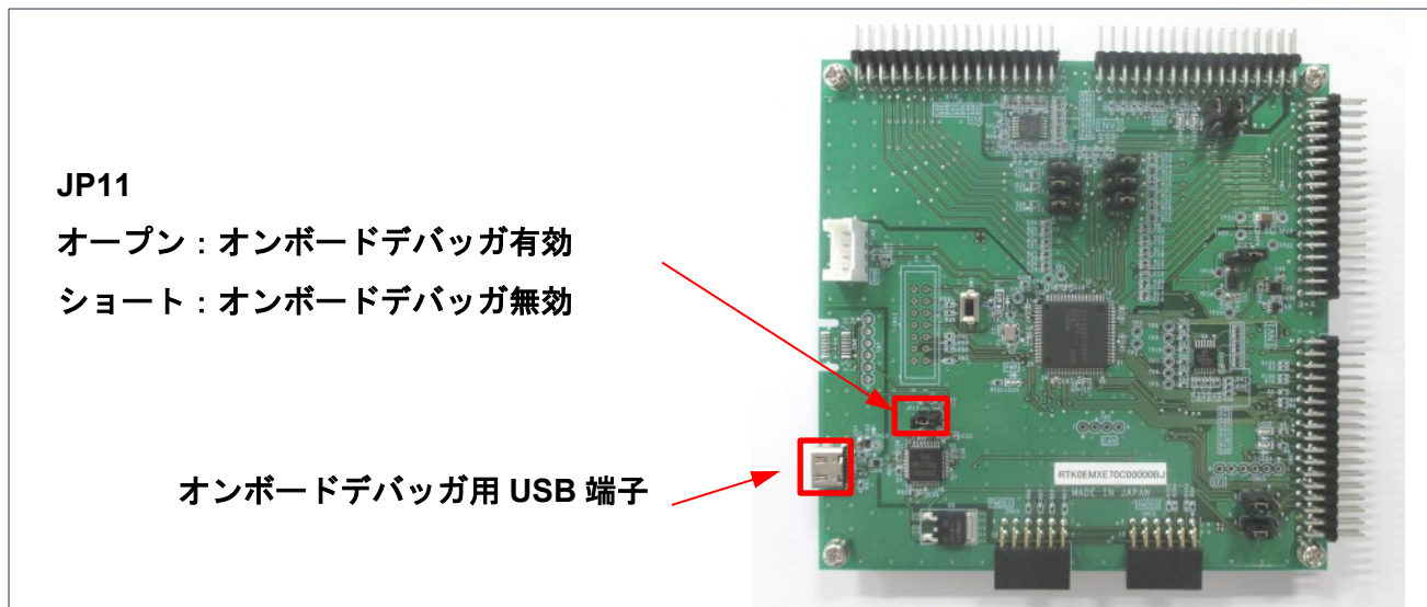
図 2-5 オンボードデバッグ(RX26T RAM64KB バージョン)
