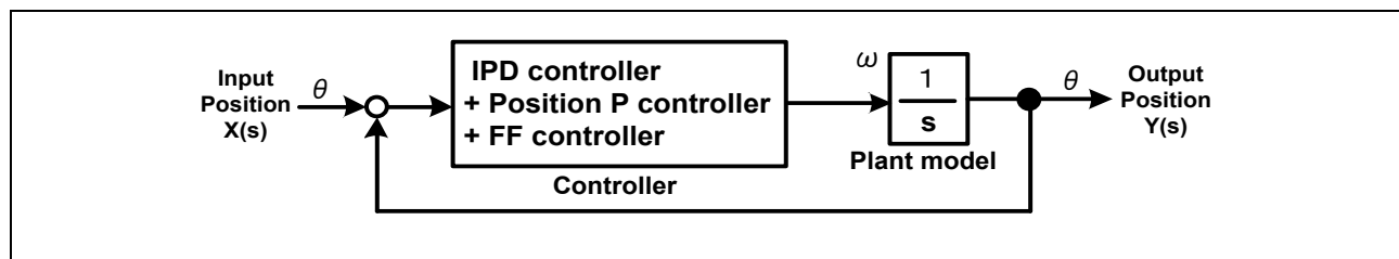
図 5-31 IPD 制御のモデル(位置)
