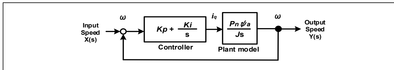
図 6-5 速度制御系のモデル
