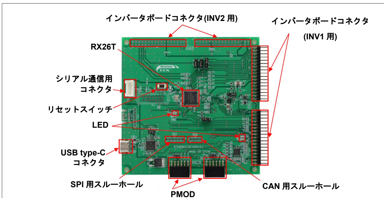
図 2-3 RX26T RAM48KB バージョン CPU ボードとインタフェース
