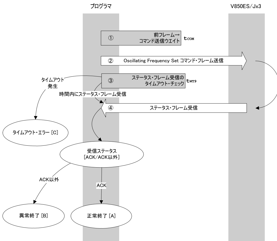
Oscillating Frequency Setコマンド処理手順
