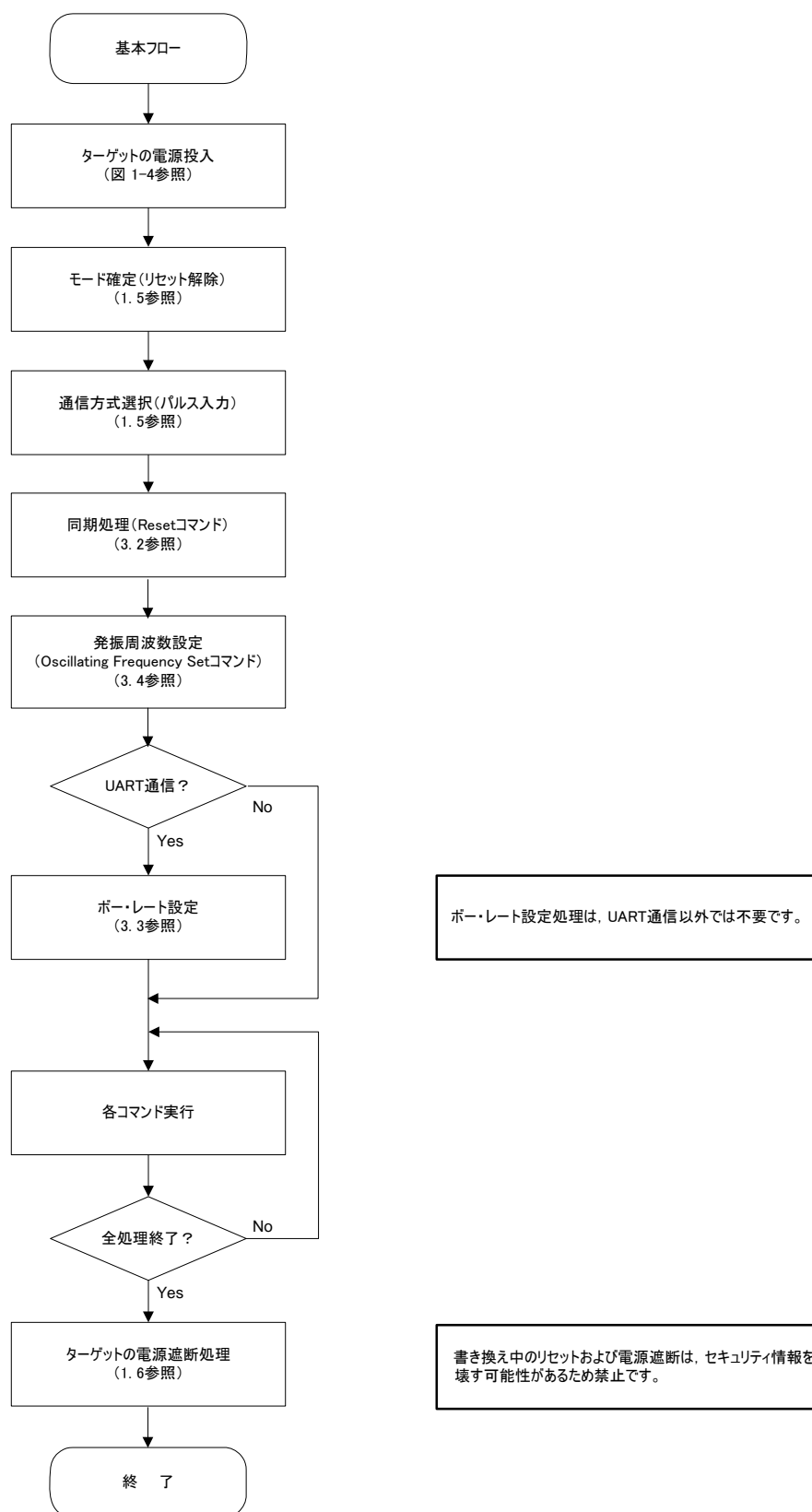
図1-7 フラッシュ処理の基本フロー・チャート
