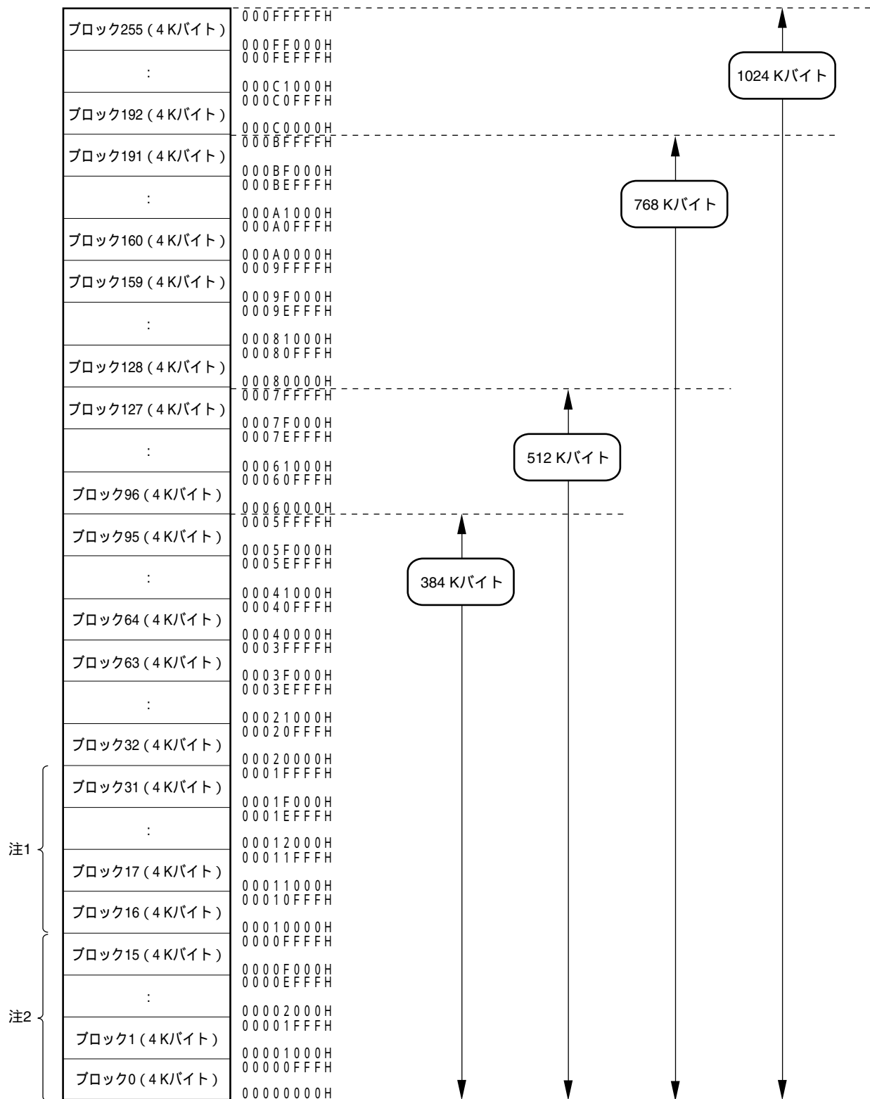
図1-3 フラッシュ・メモリ構成
