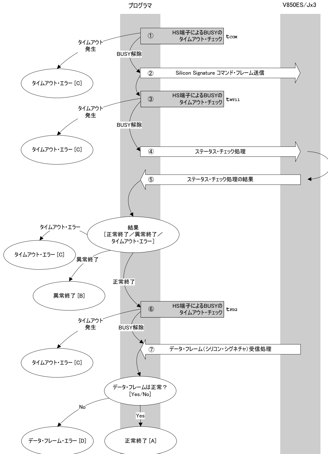
Silicon Signatureコマンド処理手順
