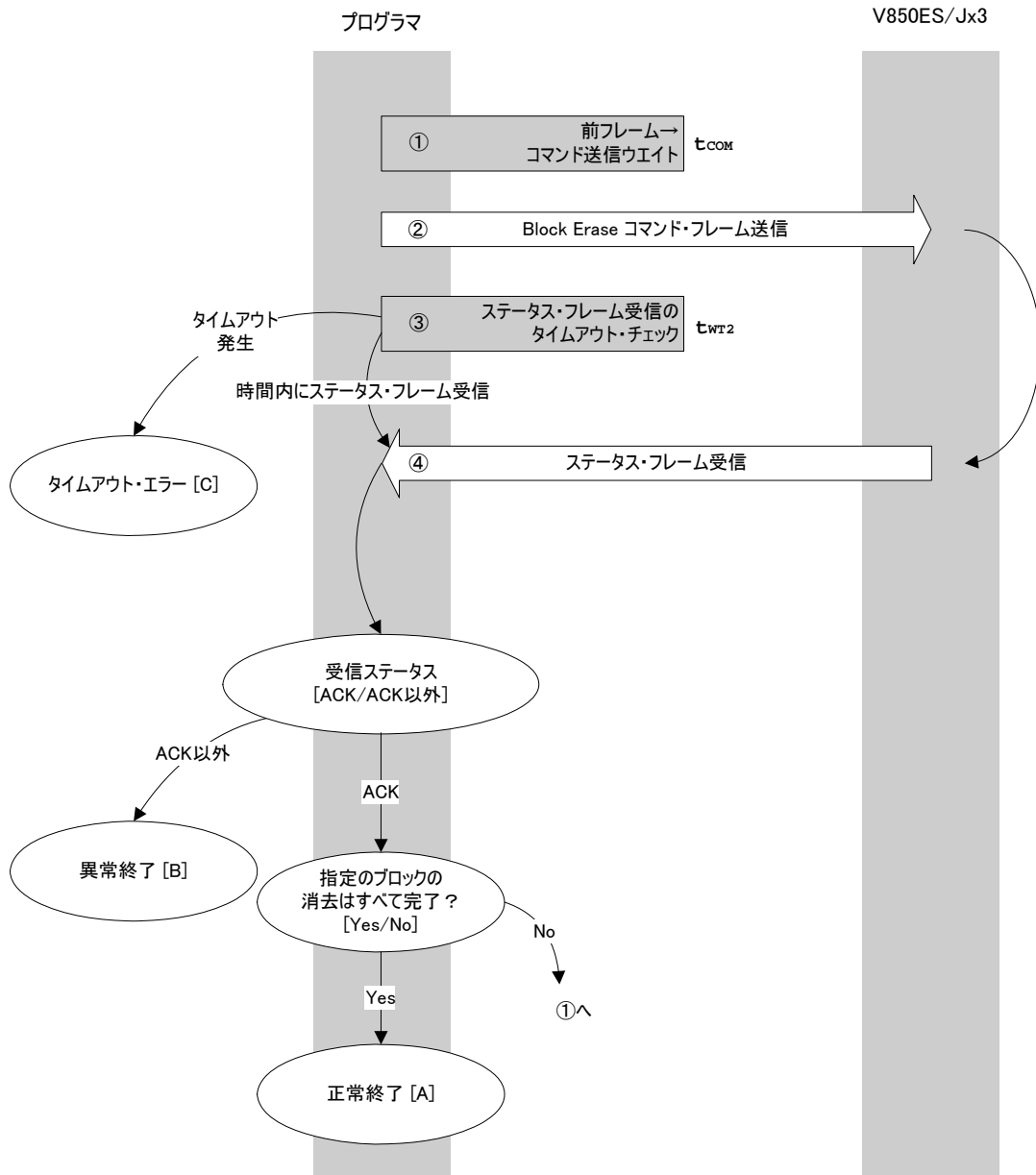
Block Eraseコマンド処理手順
