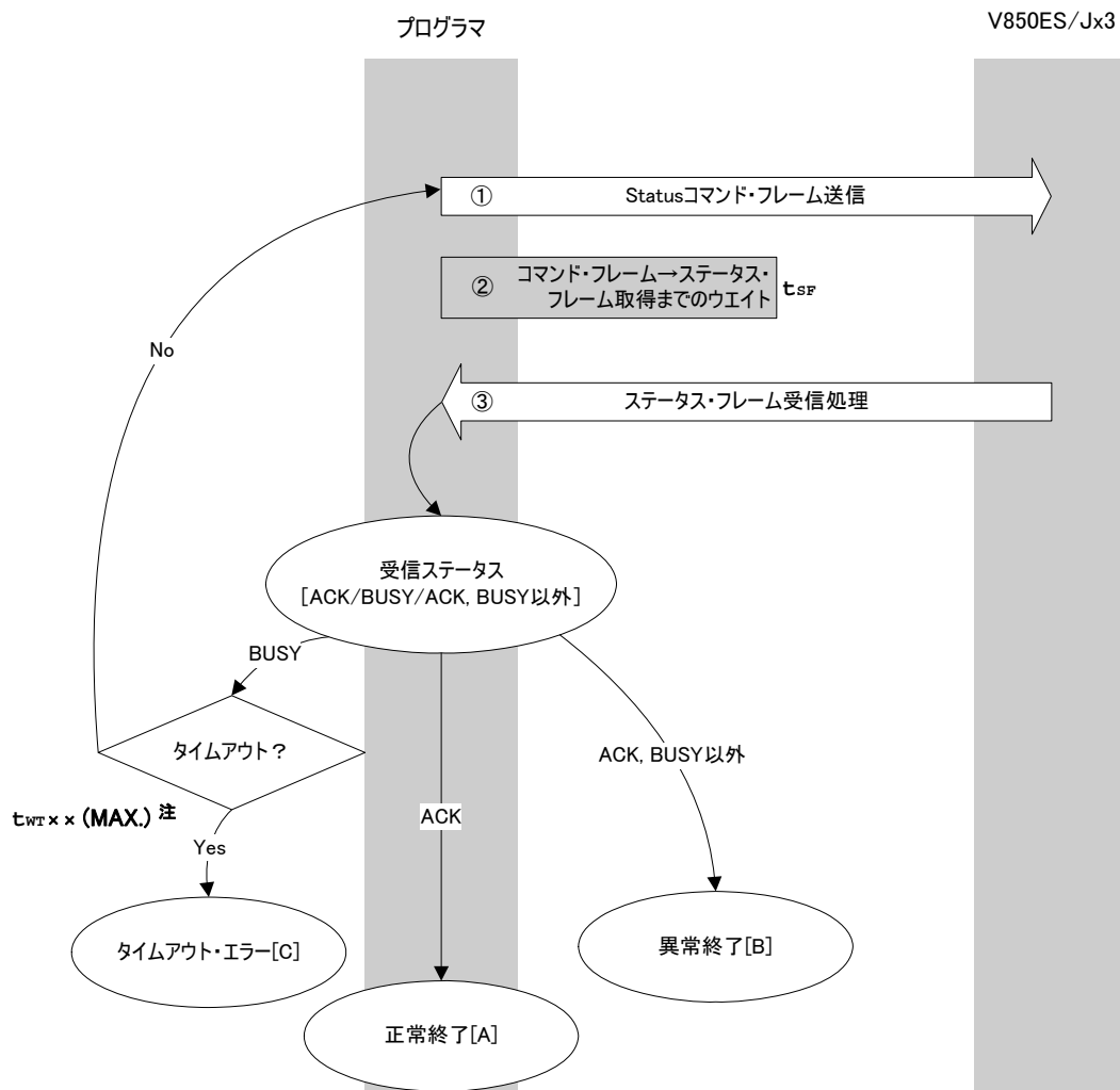
Statusコマンド処理手順
