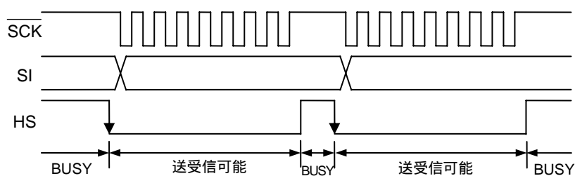
図1 - 5 CSI+HS通信のタイミング・チャート
