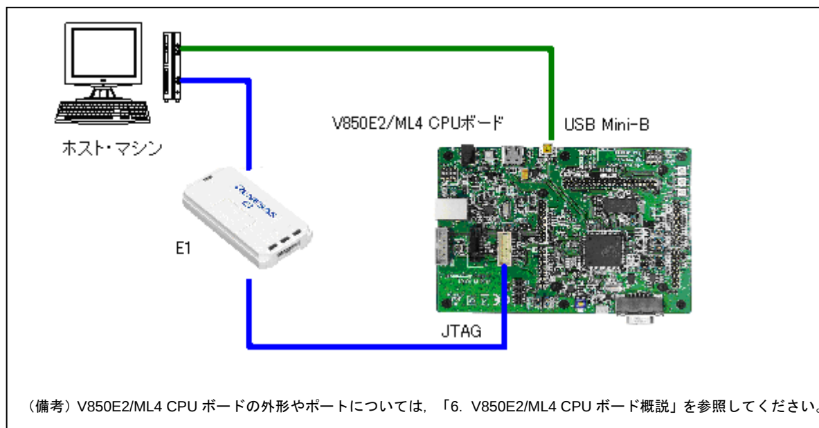
図 5-1 開発環境のシステム構成
