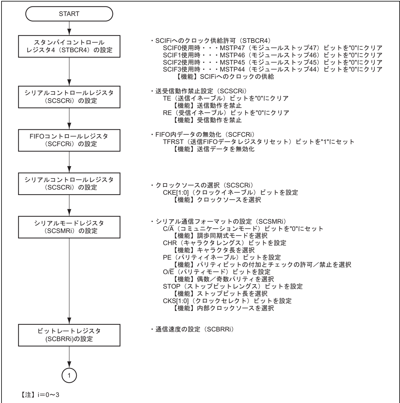
図2 UARTモード送信初期設定フロー例 (1)
