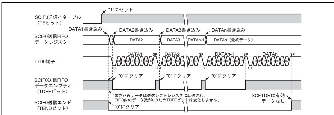
図 5 参考プログラムの動作タイミング
