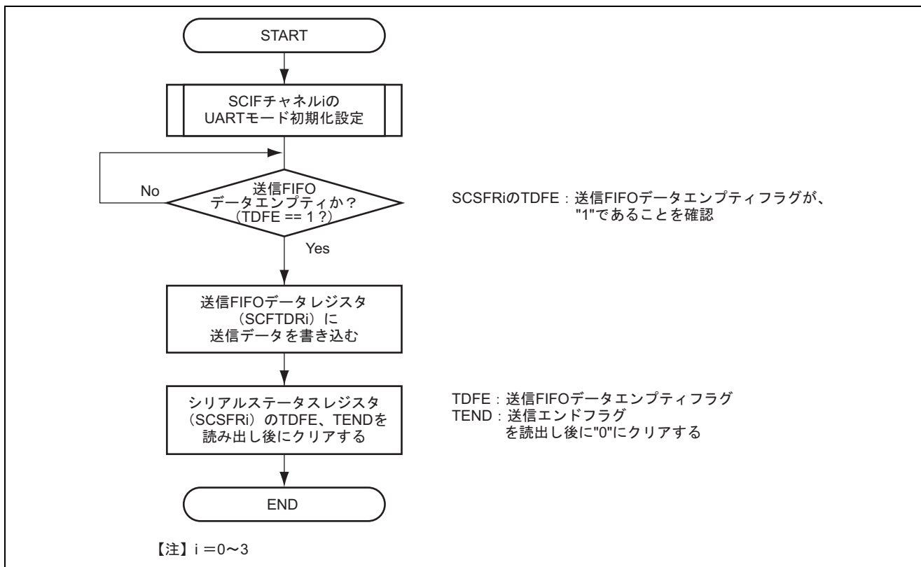
図 4 UART モード送信処理フロー例
