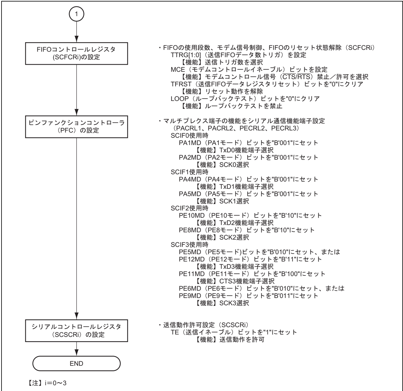
図 3 UART モード送信初期設定フロー例 (2)
