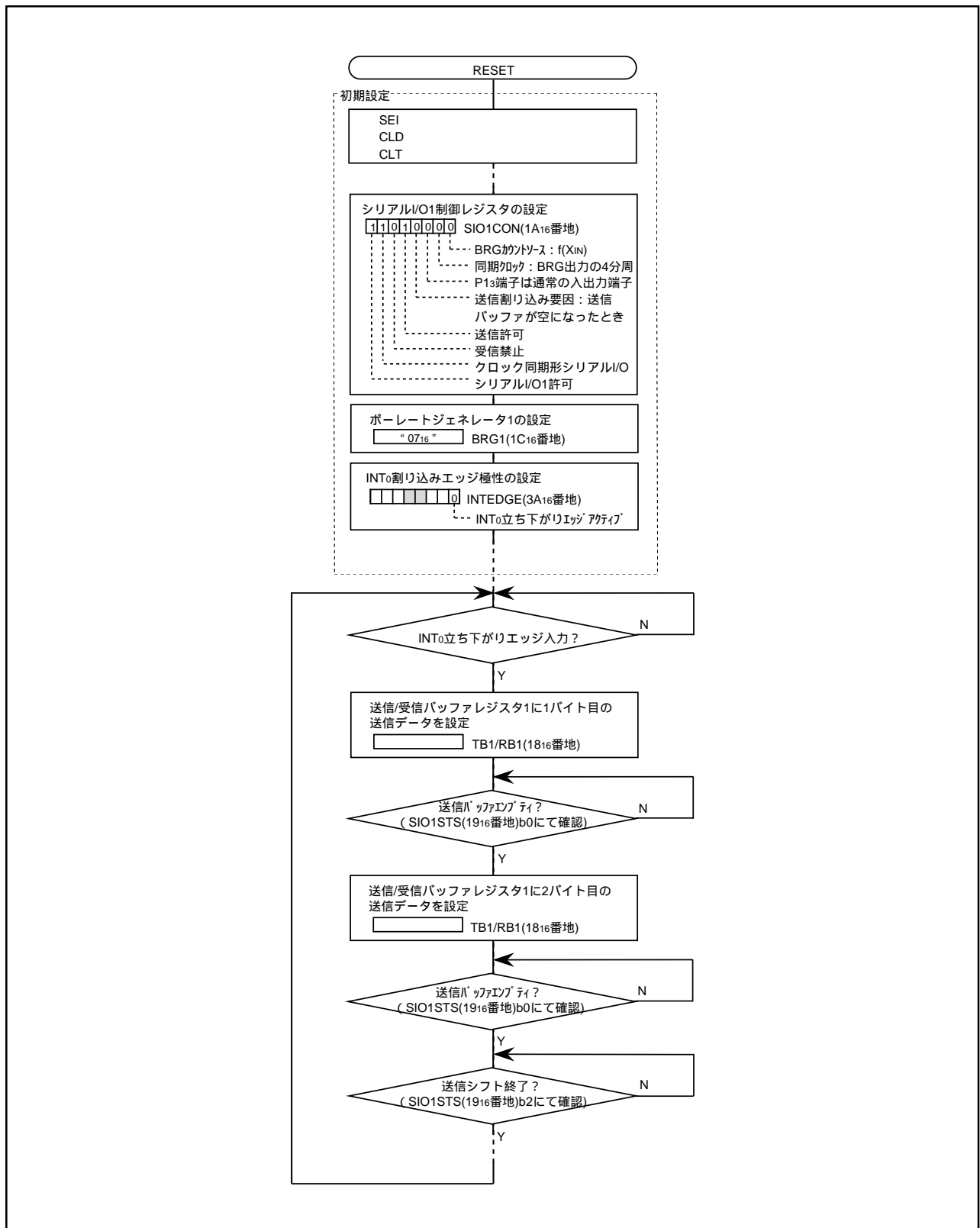
図5 . 送信側の制御手順例
