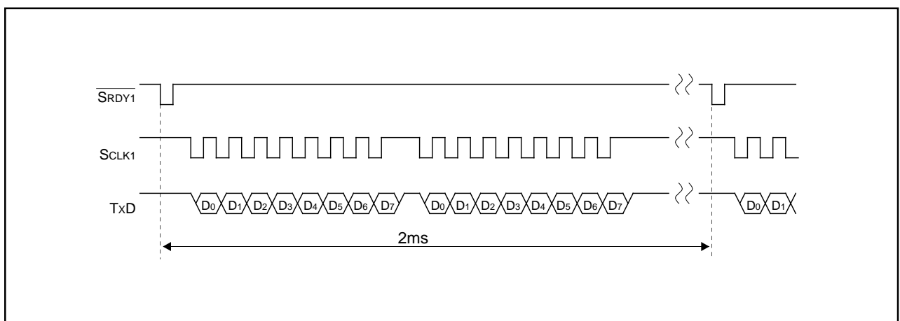
図4 . タイミング図
