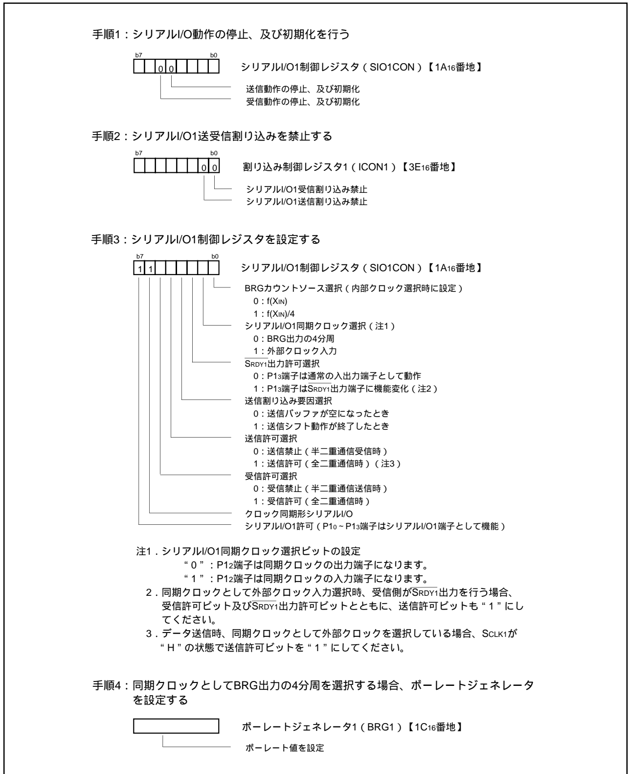
図1 . シリアルI/O1のクロック同期形設定方法(1)
