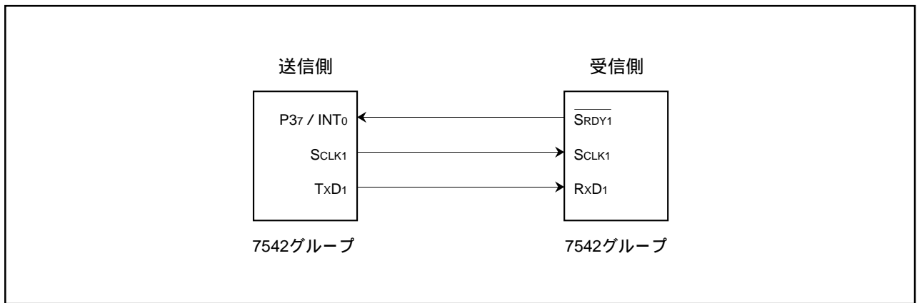
図3 . 接続図
