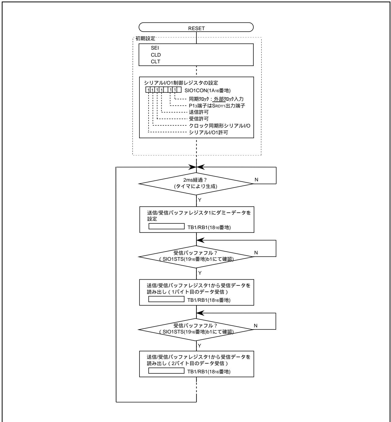
図6 . 受信側の制御手順例
