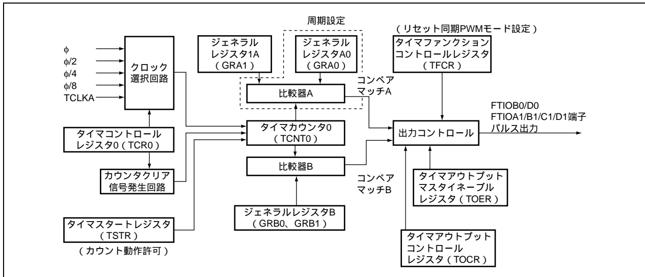
図 2.1 TimerZ CH0、CH1 ブロック図
