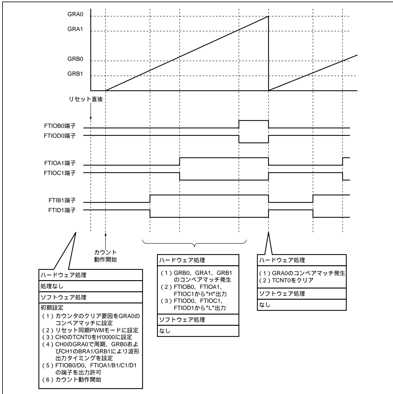
図 3.1 3相 PWM 出力動作原理
