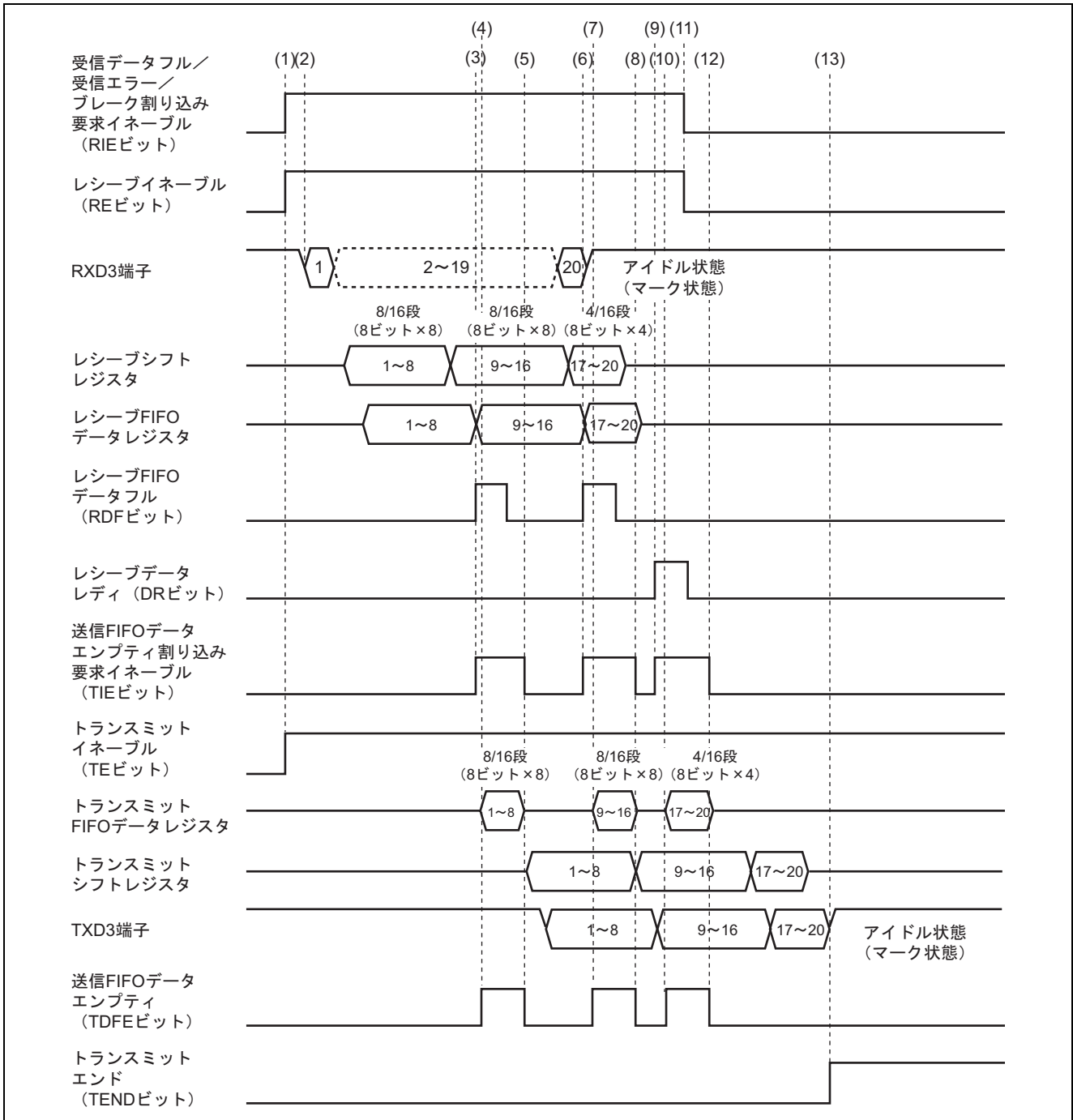
図3 動作説明
