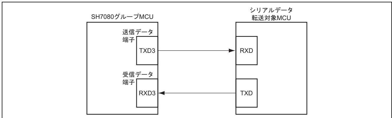
図 1 FIFO 付き調歩同期式シリアルデータ送受信動作概要
