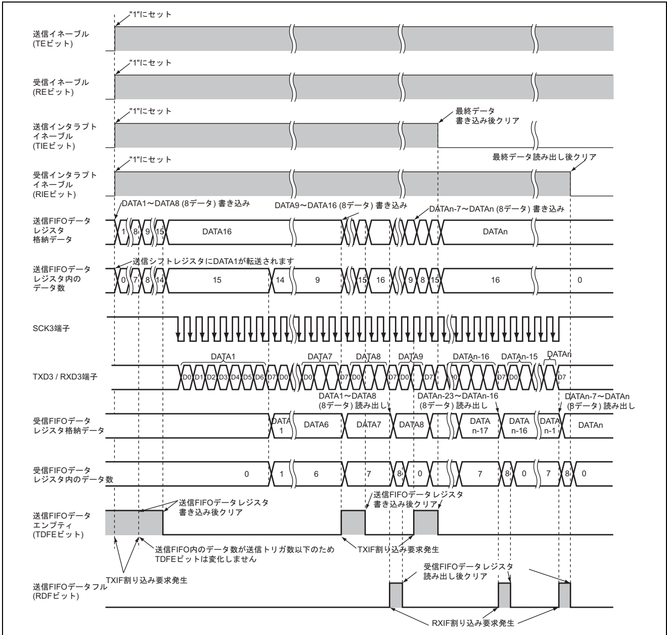
図3 動作説明
