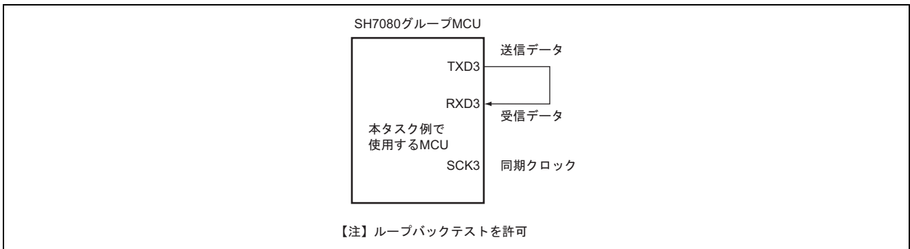
図 1 SCIF クロック同期式シリアルデータ送受信
