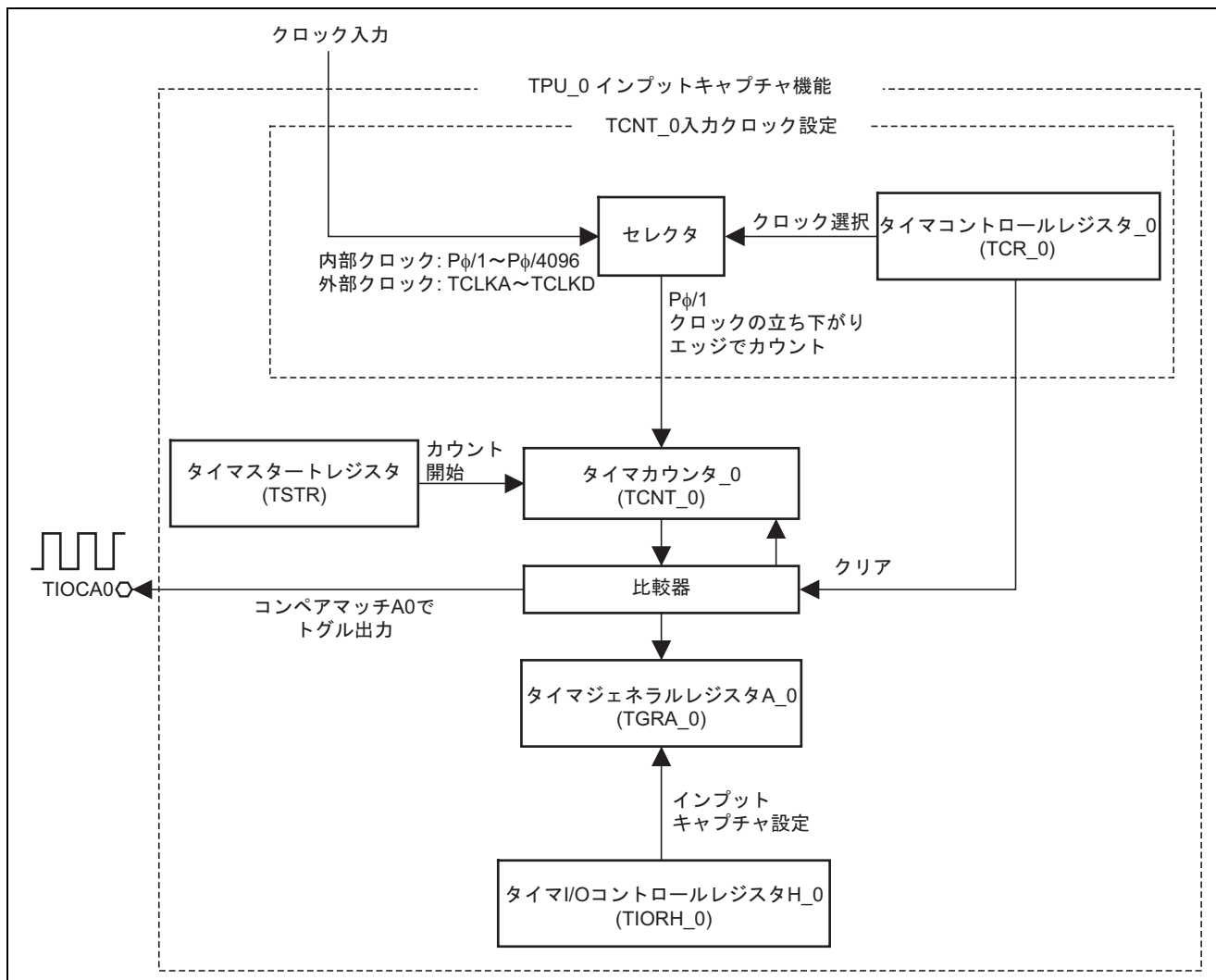
図 2 TPU チャンネル 0 (TPU_0) のブロック図
