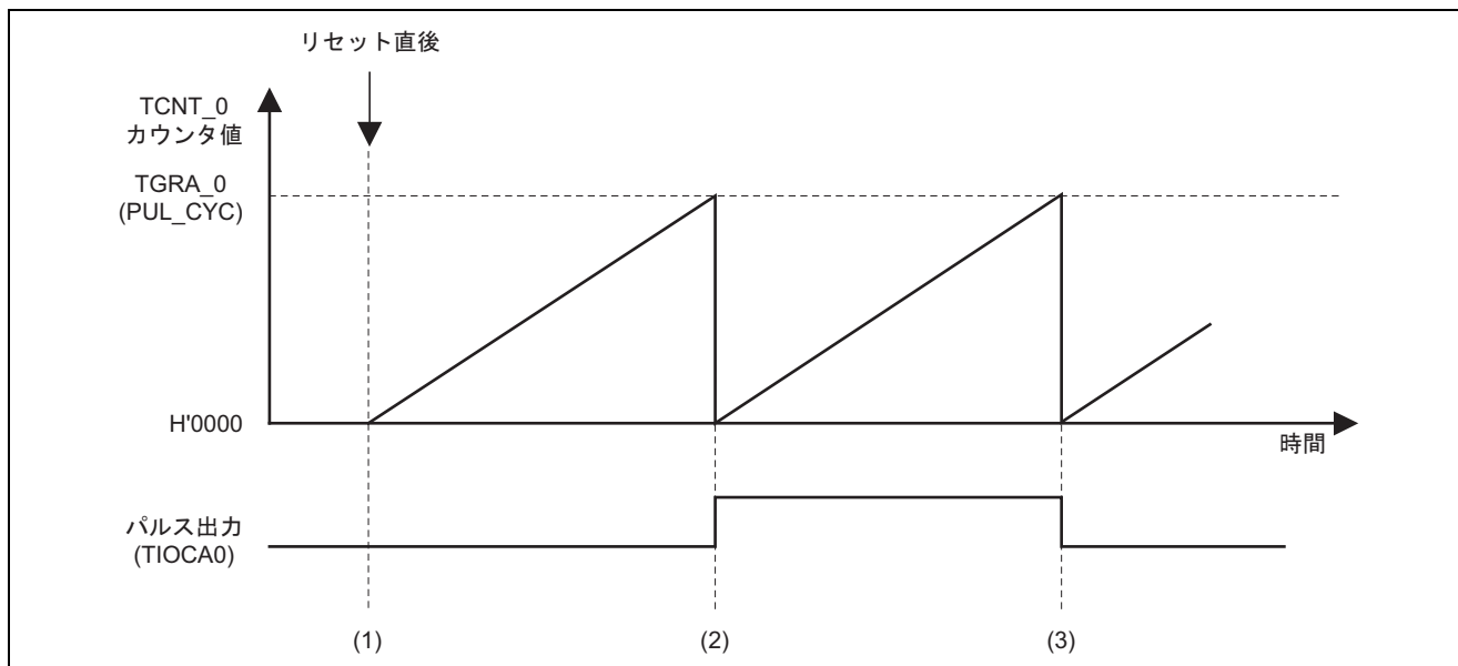
図3 パルス出力動作説明
