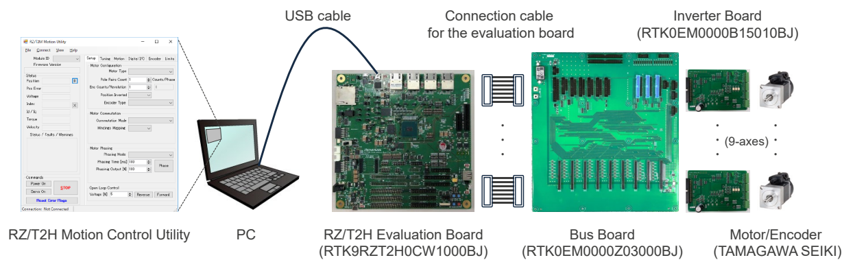
図 2-1 ハードウェア構成(接続構成)
