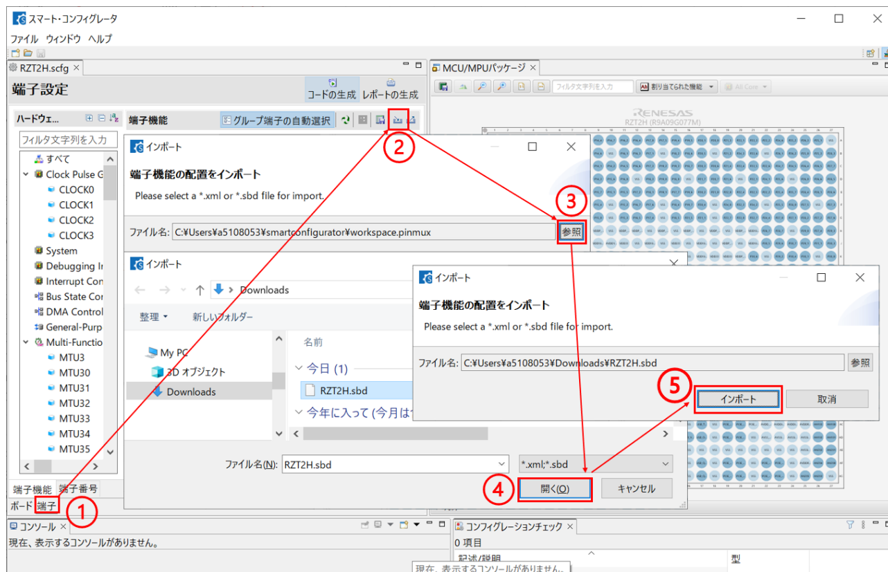
図 3 RZ スマート・コンフィグレータに Smart bundle ファイルをインポート
