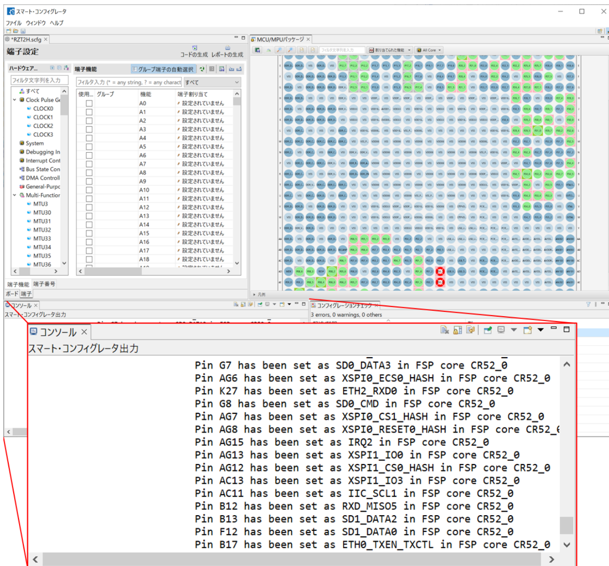
図 5 端子設定の競合を確認：「コンソール」ビュー
