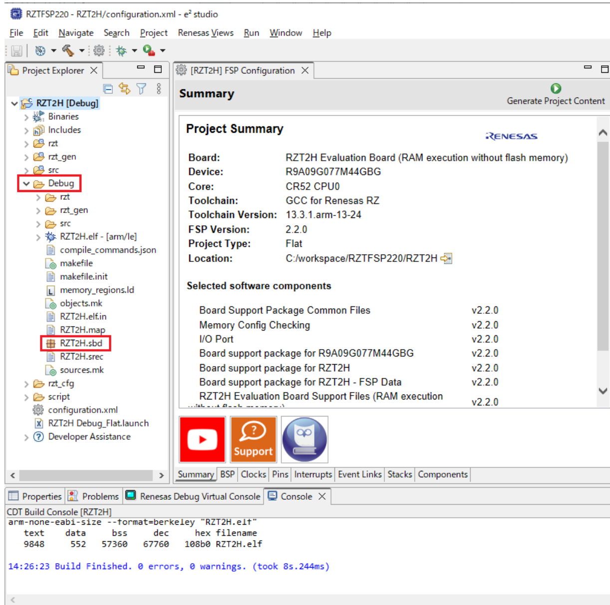
図 2 Smart bundle ファイルの生成確認
