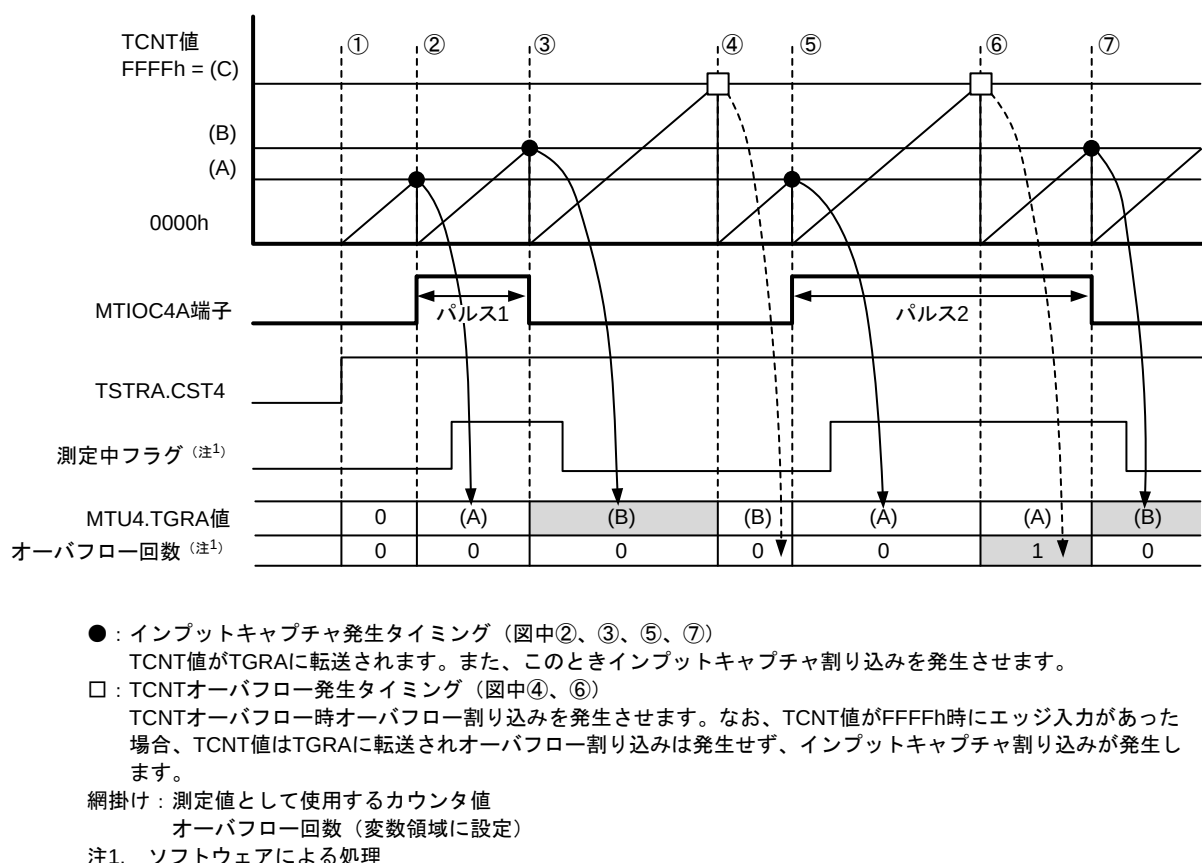
図2.21 MTU インพุットキャプチャ動作説明
