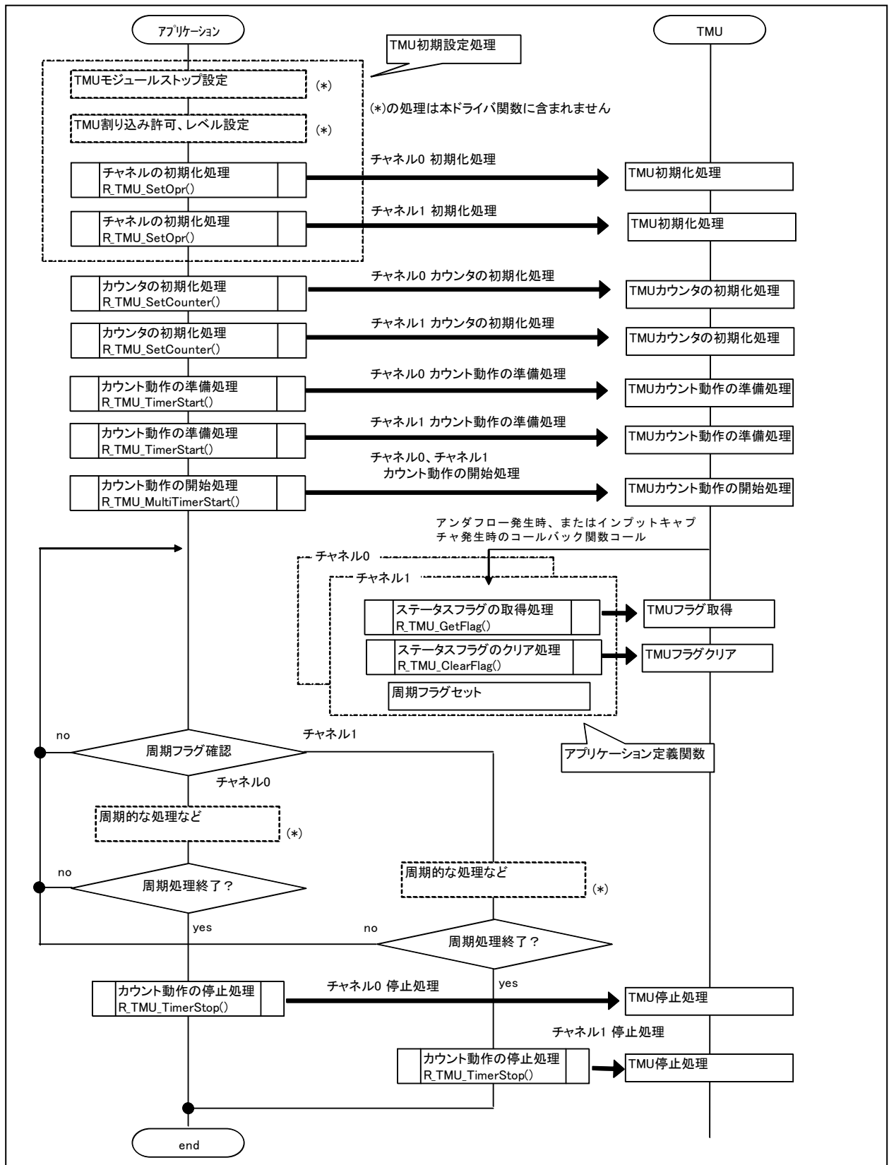
図 2. TMU 周期割り込みプログラム例(マルチスタート)
