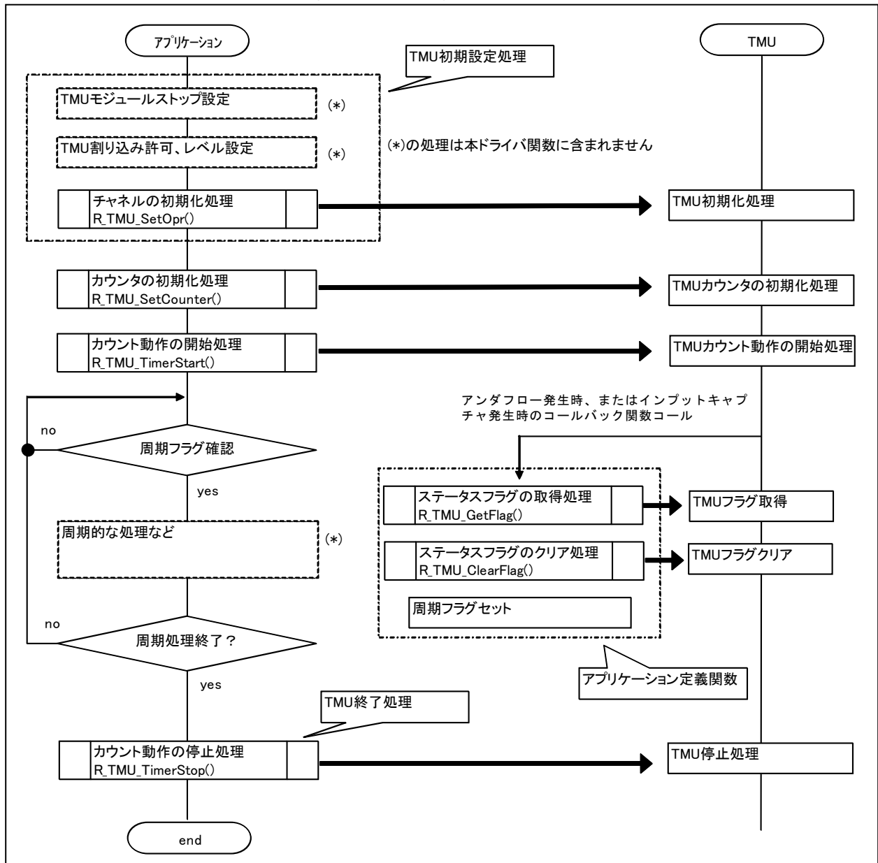
図 1. TMU 周期割り込みプログラム例(単一チャンネル)
