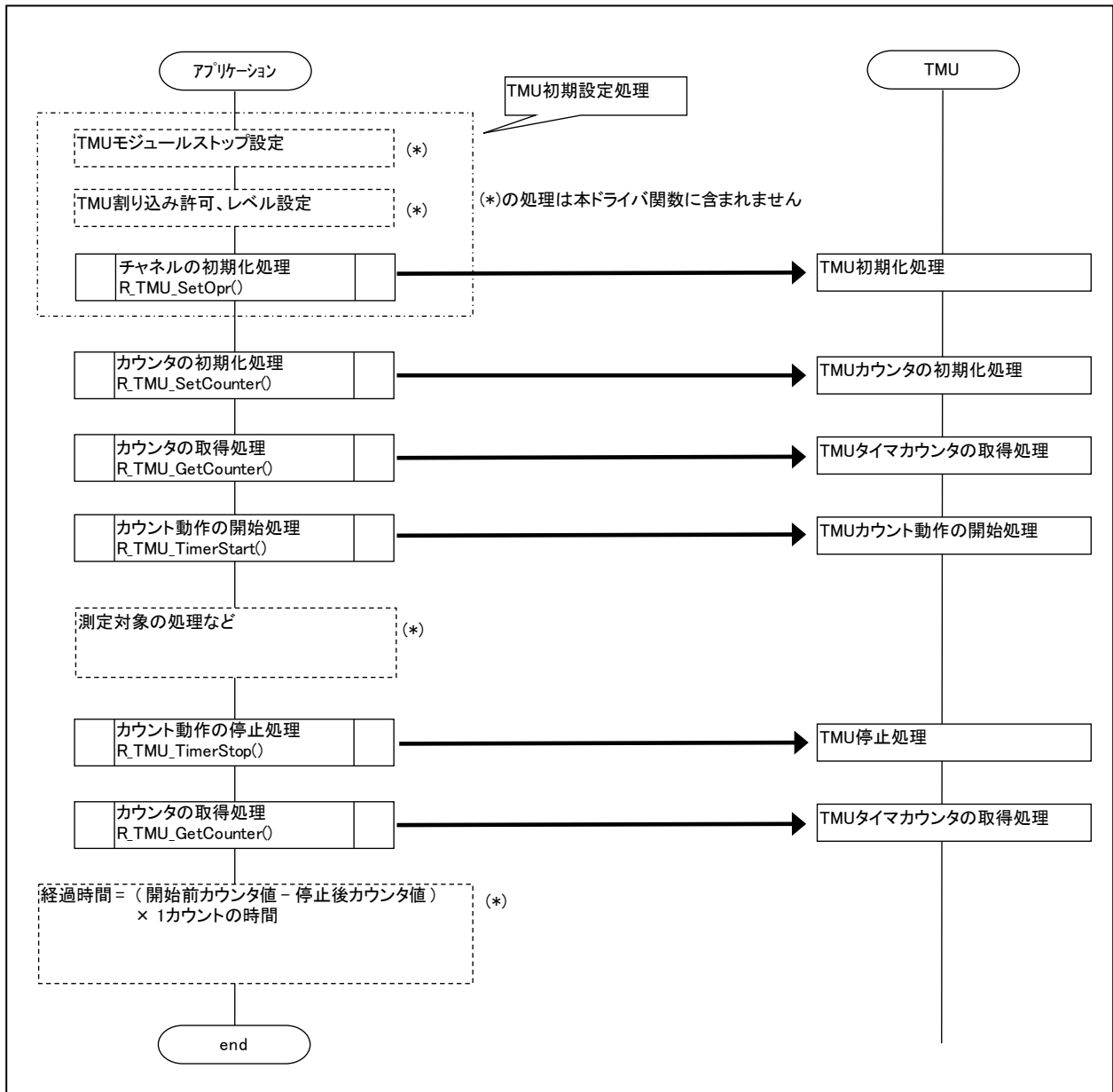
図 3. TMU 経過時間測定プログラム例
