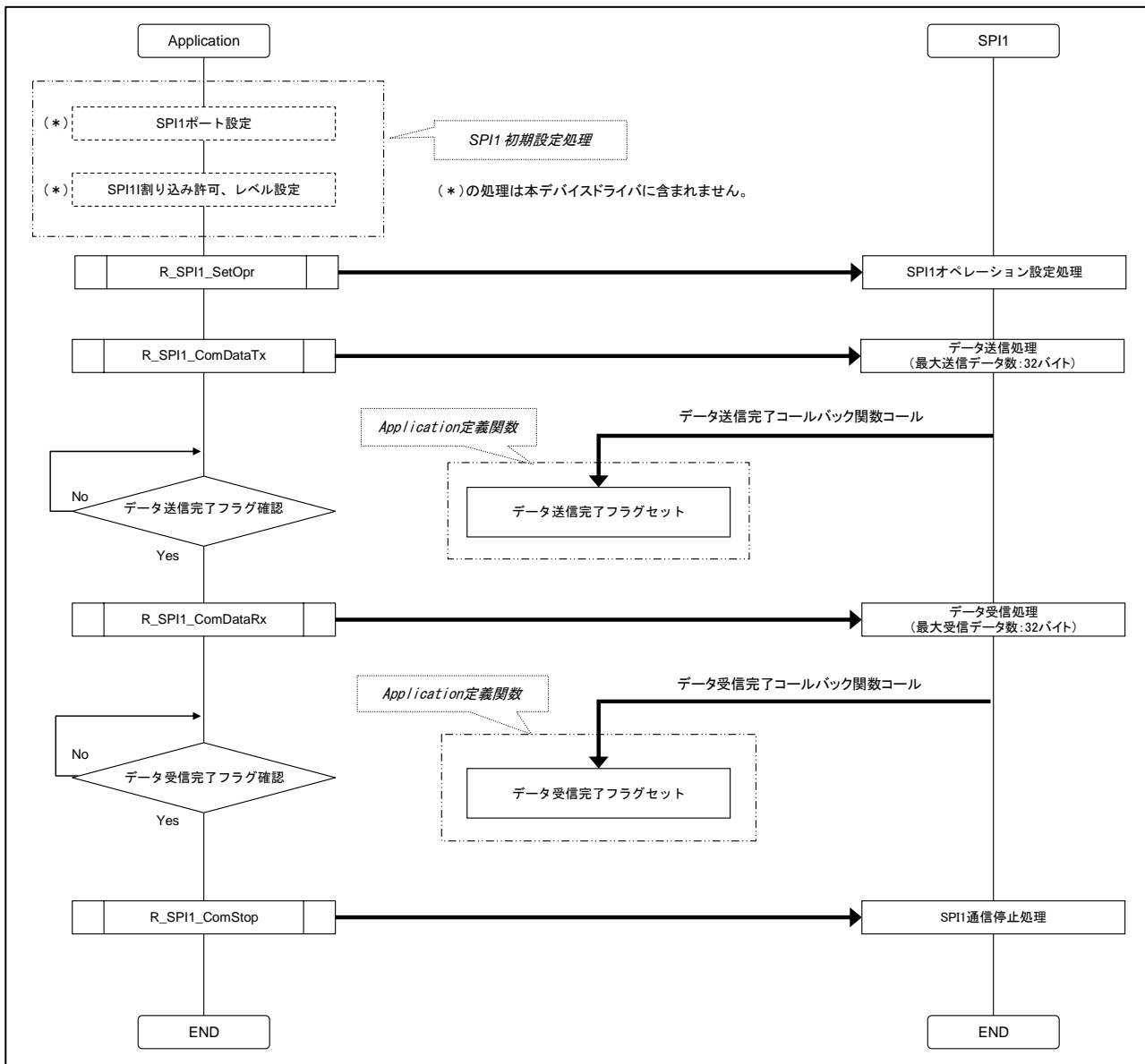
図 5. SPI デバイスデータ送受信アクセス時の使用例
