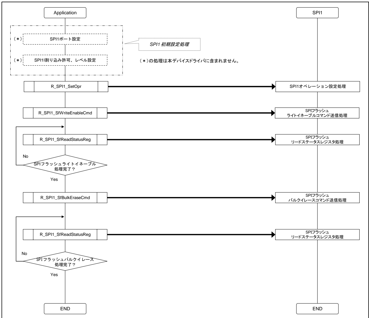
図 4. SPI フラッシュバルクイレースアクセスの処理例
