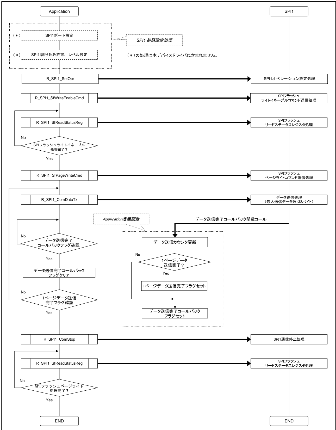
図 2. SPI フラッシュページライトアクセスの処理例
