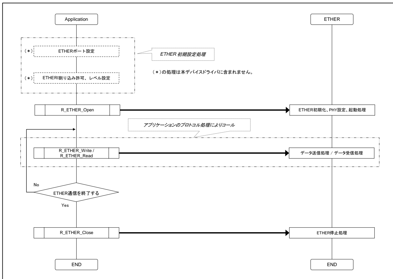
図 1. ETHERドライバの使用例
