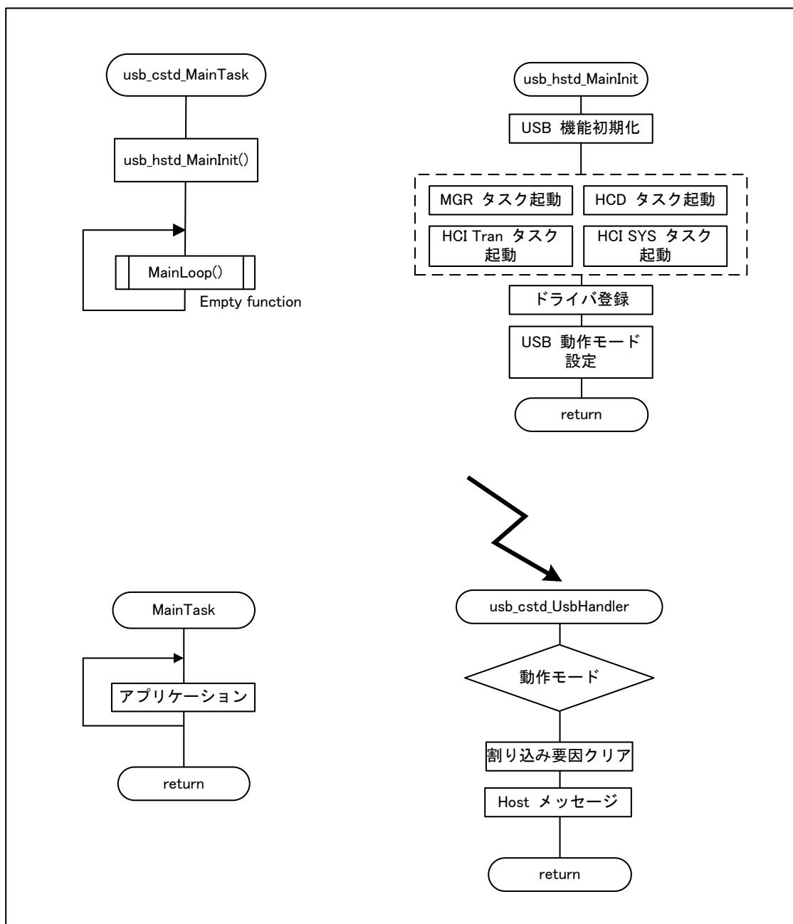
図2.2 概略フロー
