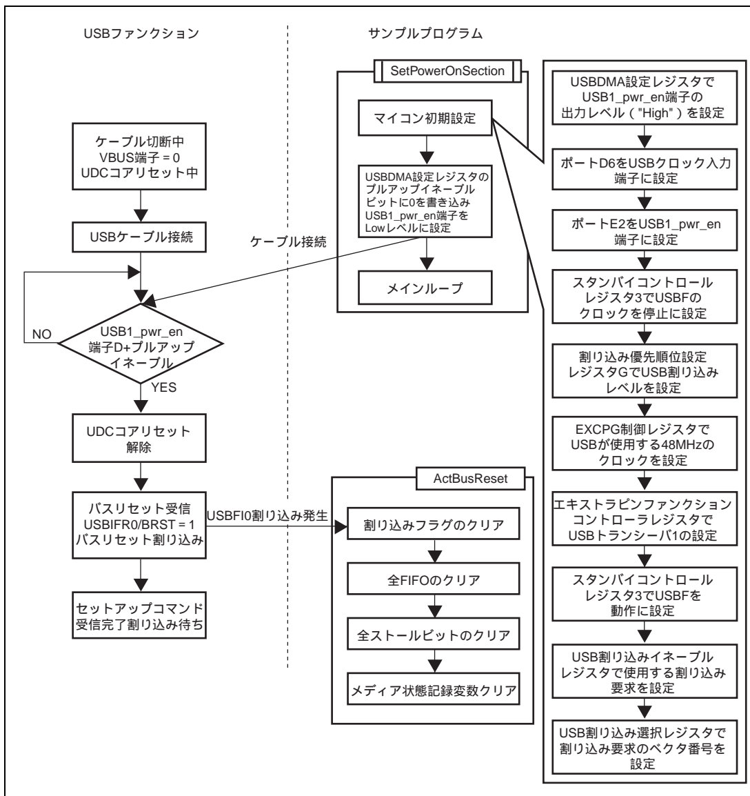
図 5.3 ケーブル接続時割り込み
