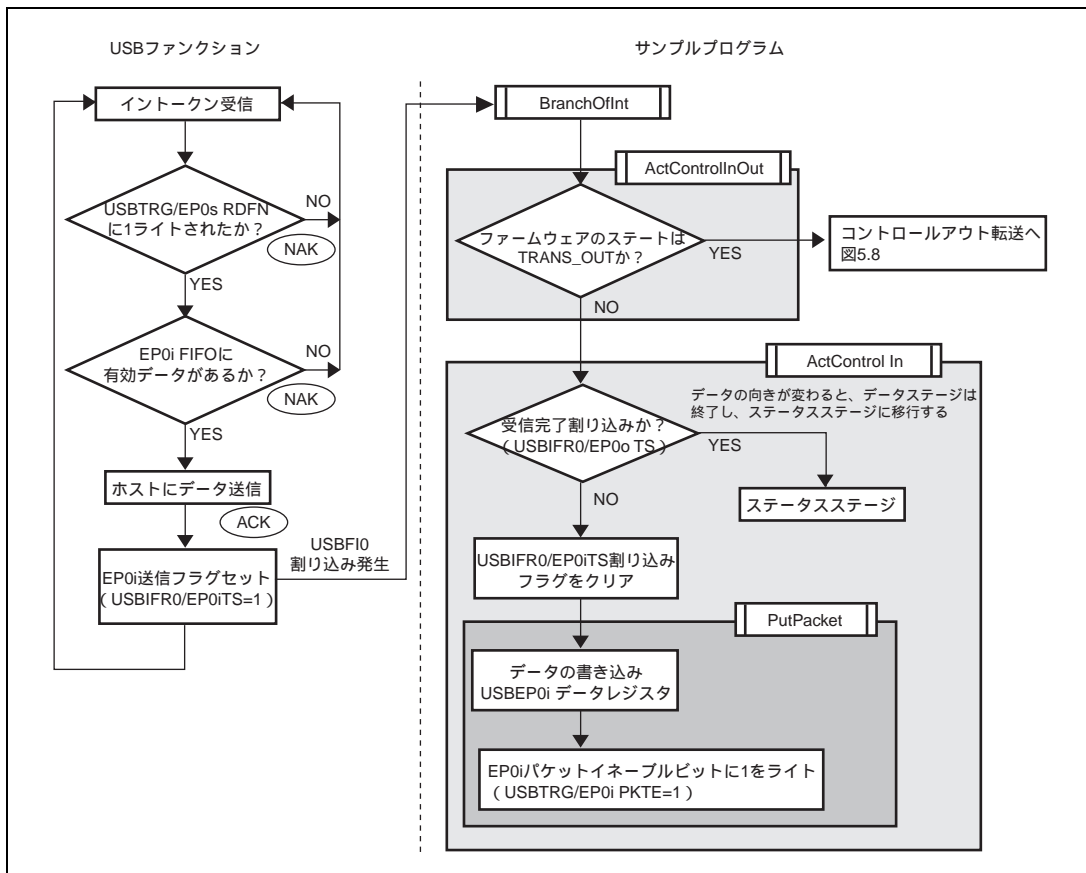
図 5.7 データステージ (コントロールイン転送)
