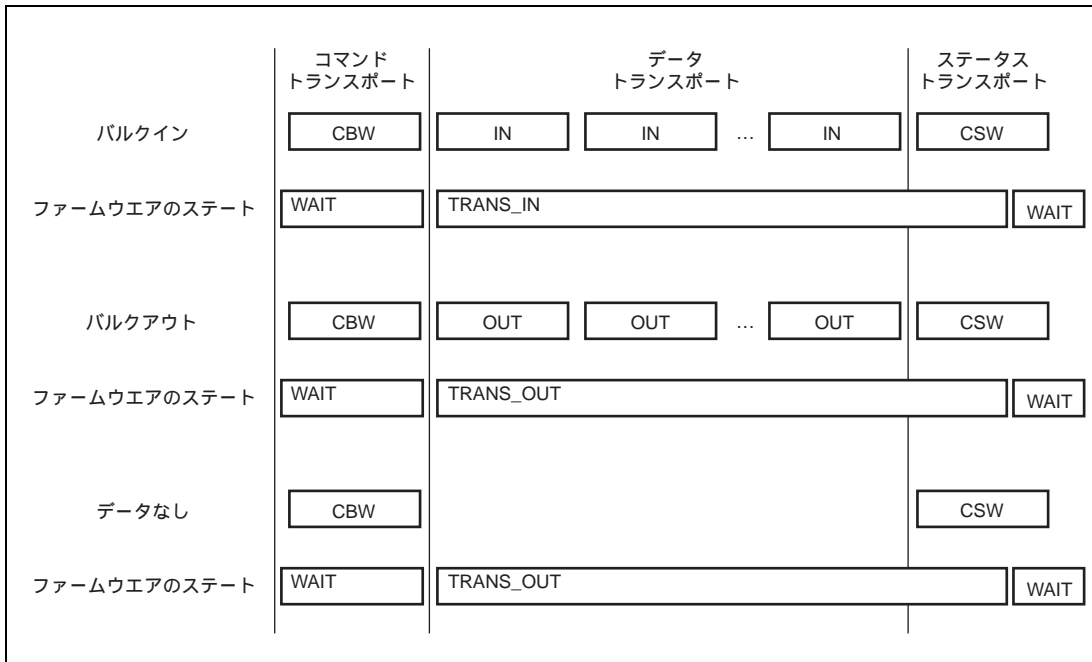
図 5.12 Bulk-Only Transport における各ステージ
