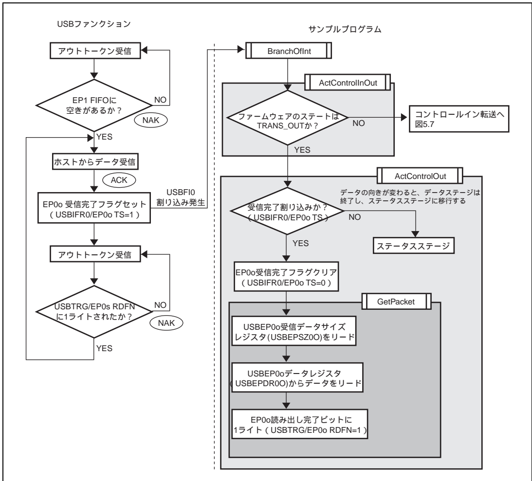
図5.8 データステージ (コントロールアウト転送)
