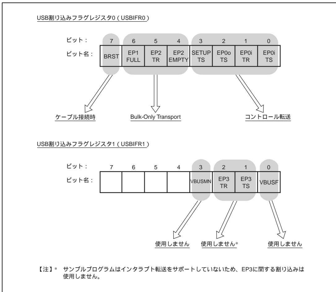
図 5.2 割り込みフラグの種類
