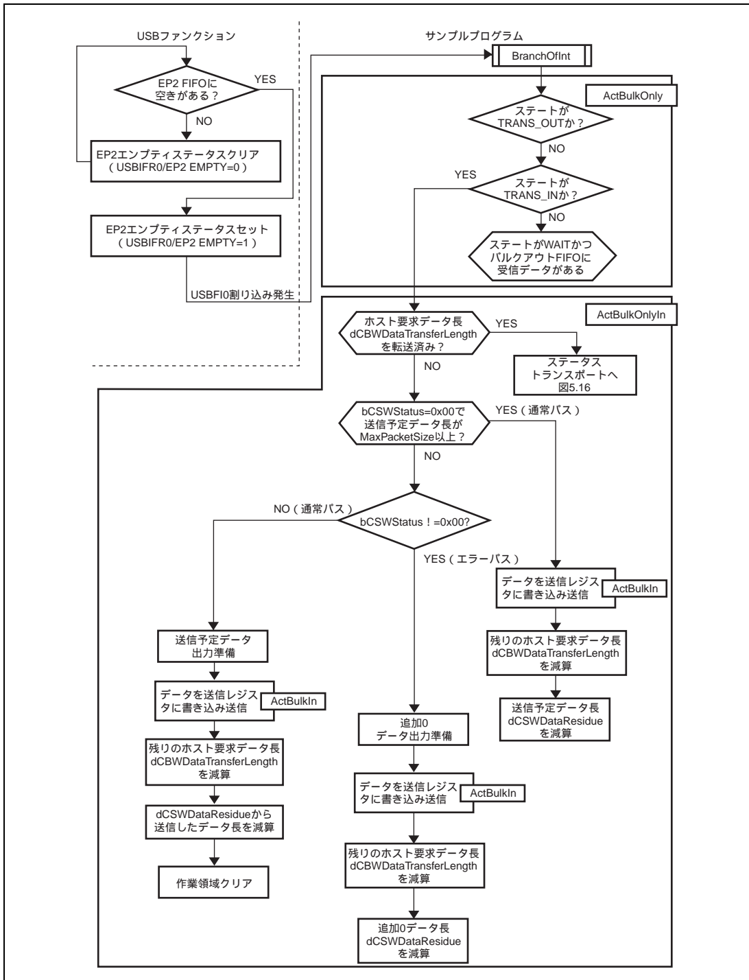
図 5.14 データトランスポート (バルクイン転送)
