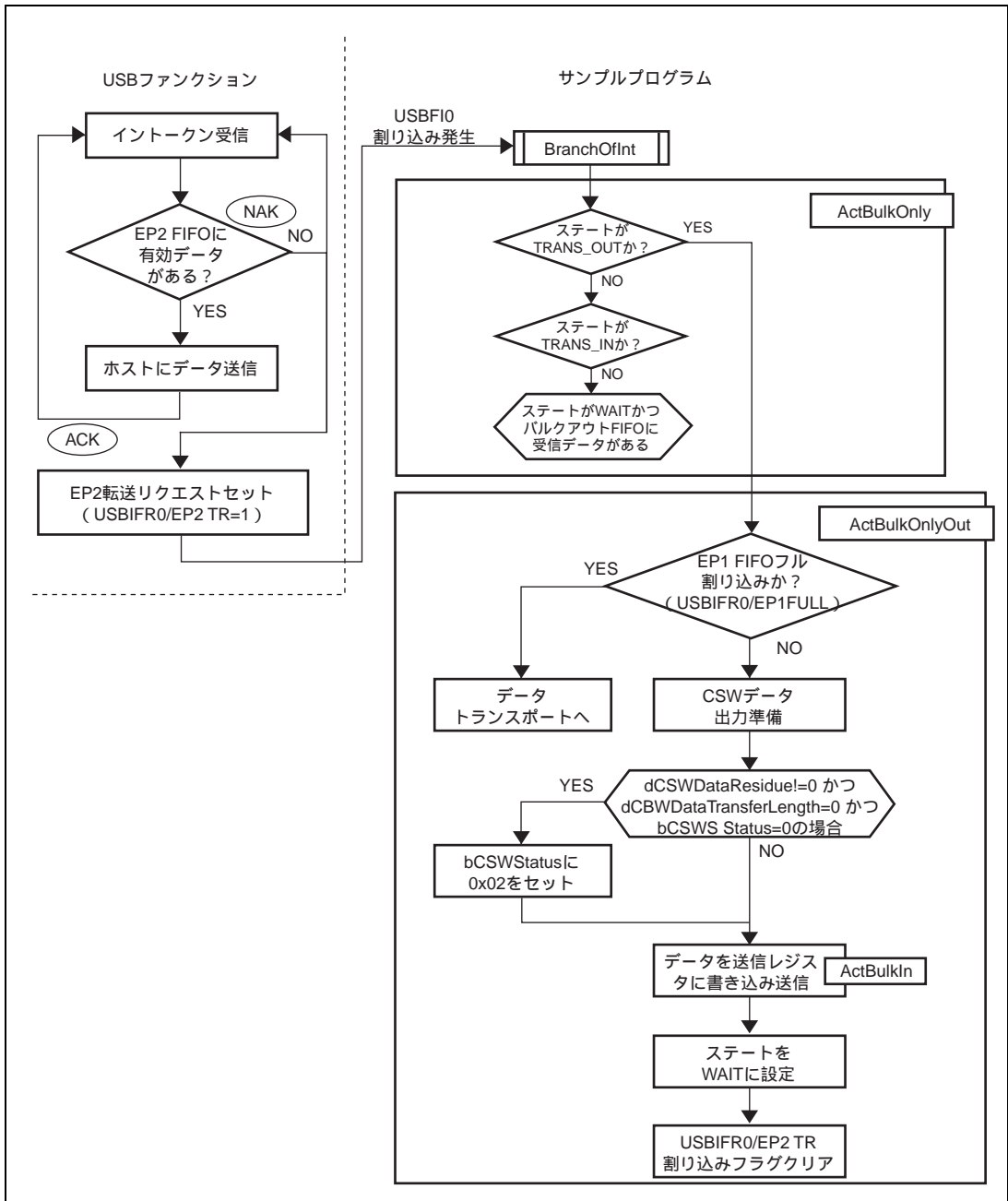
図 5.17 ステータス転送 (データ転送バルクアウト転送)
