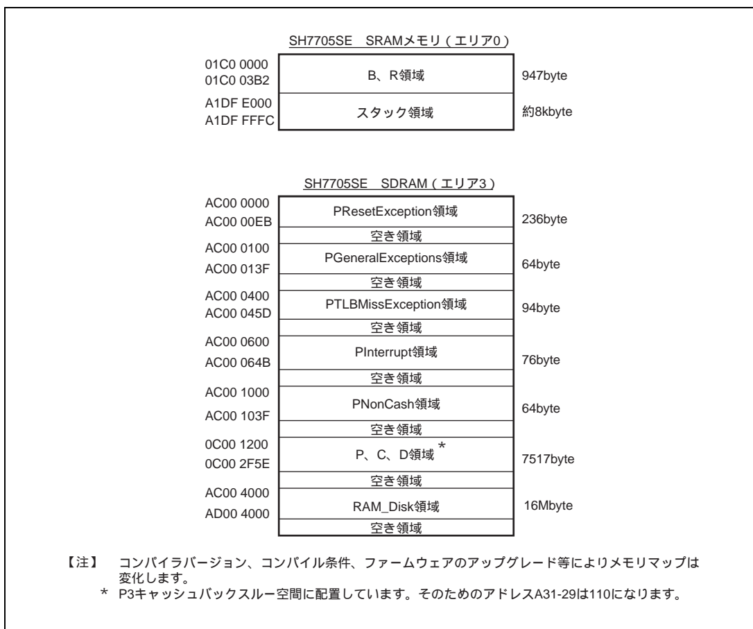
図 3.5 メモリマップ
