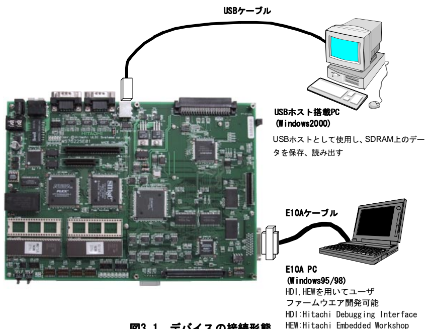
図3.1 デバイスの接続形態
