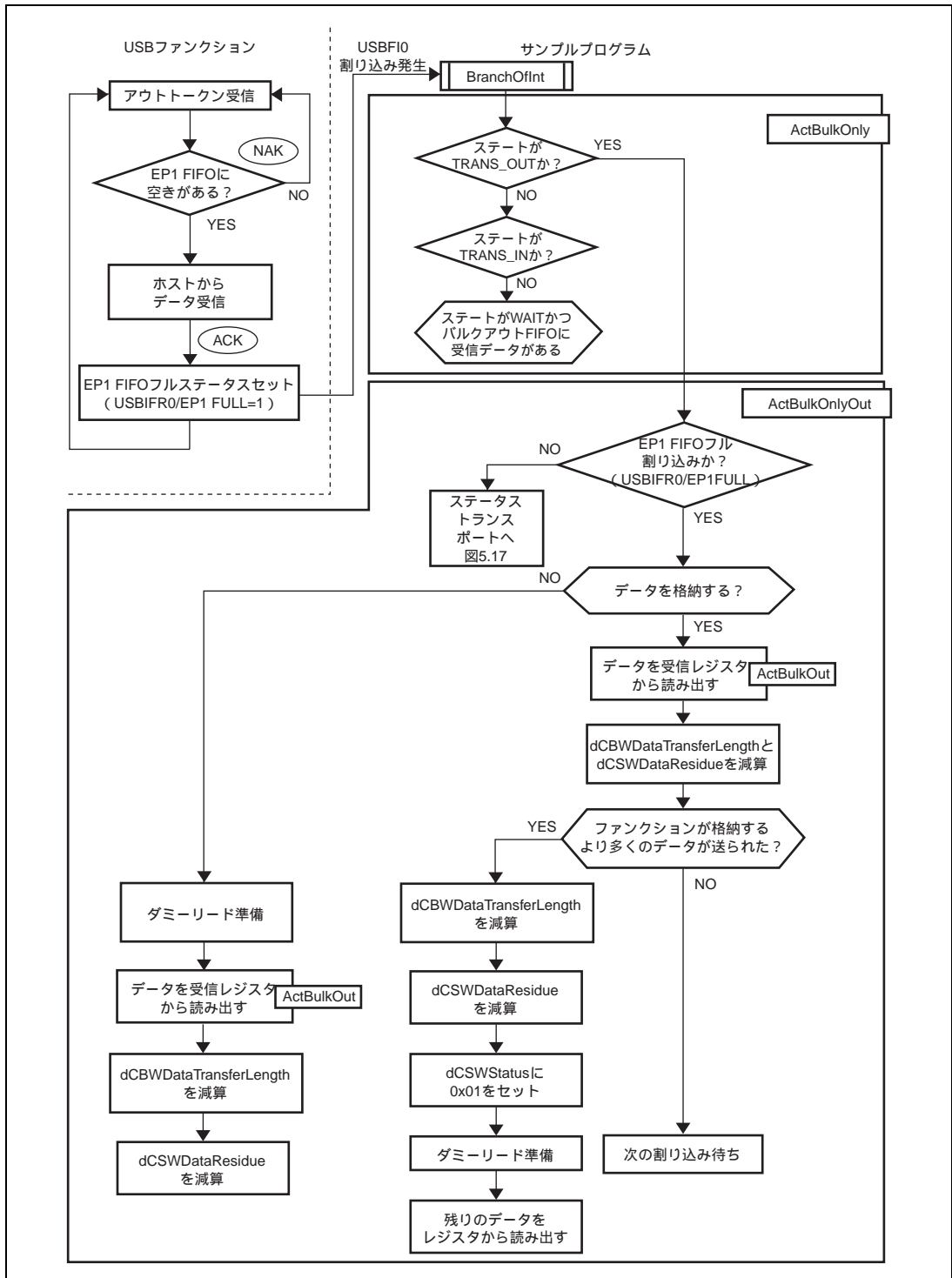
図 5.15 データトランスポート (バルクアウト転送)
