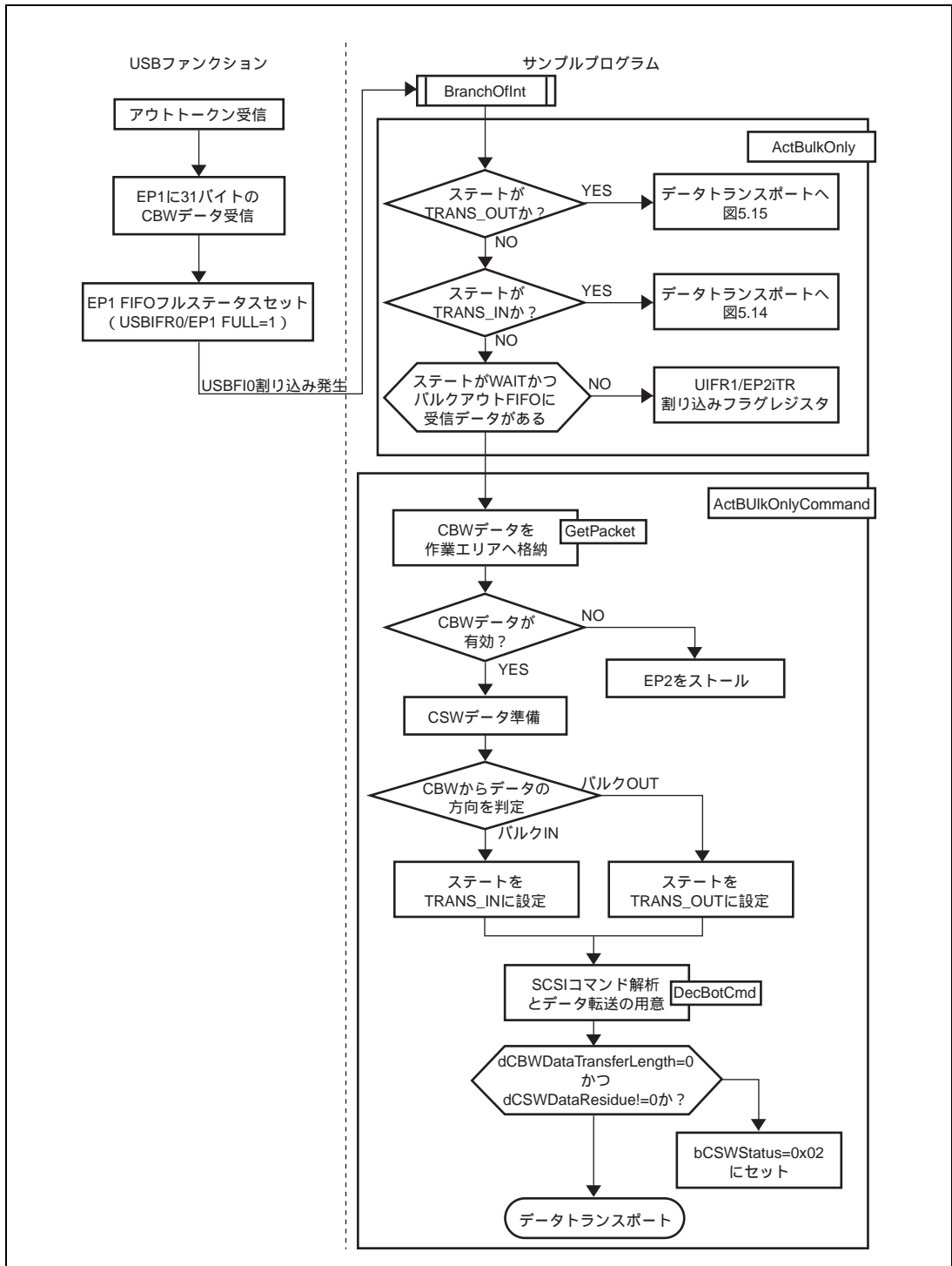
図 5.13 コマンドトランスポート
