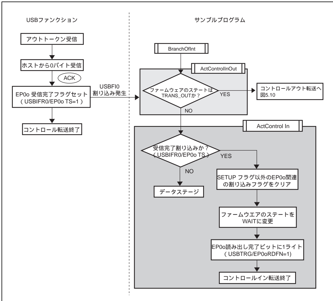
図 5.9 ステータスステージ (コントロールイン転送)
