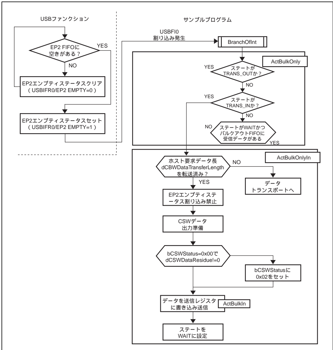
図 5.16 ステータストランスポート (データトランスポートバルクイン転送)
