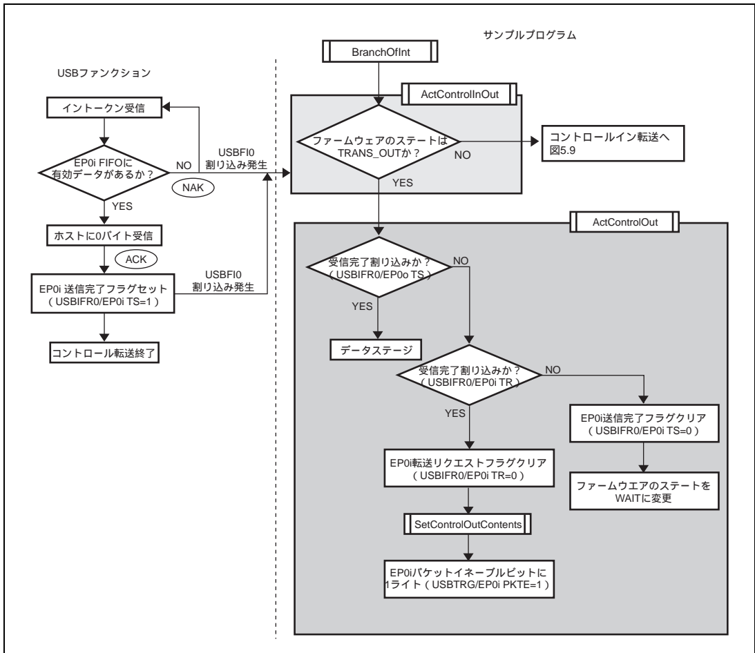
図 5.10 ステータスステージ (コントロールアウト転送)
