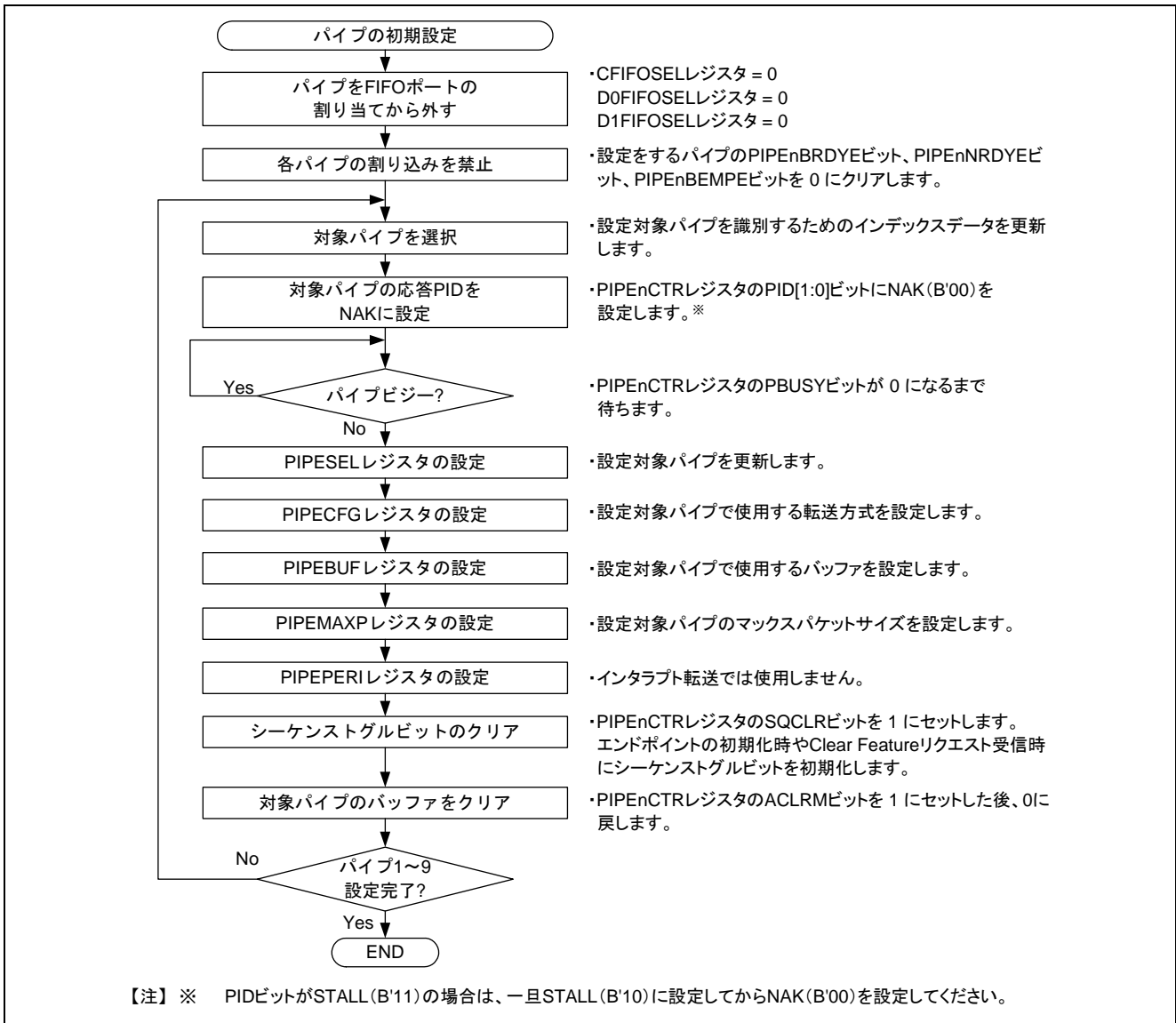
図6 パイプの初期化手順
