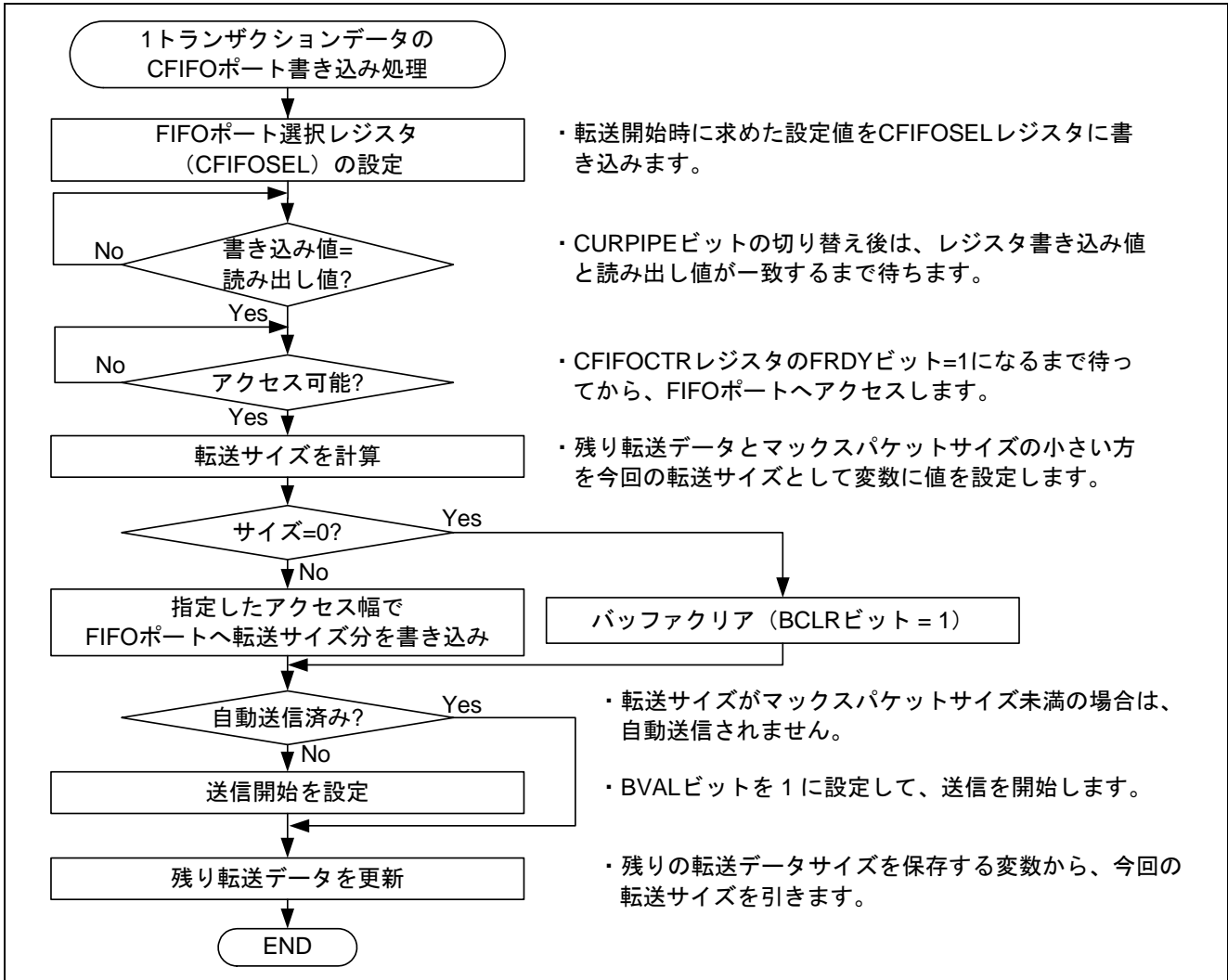
図16 1トランザクションデータのCFIFOポート書き込み処理例
