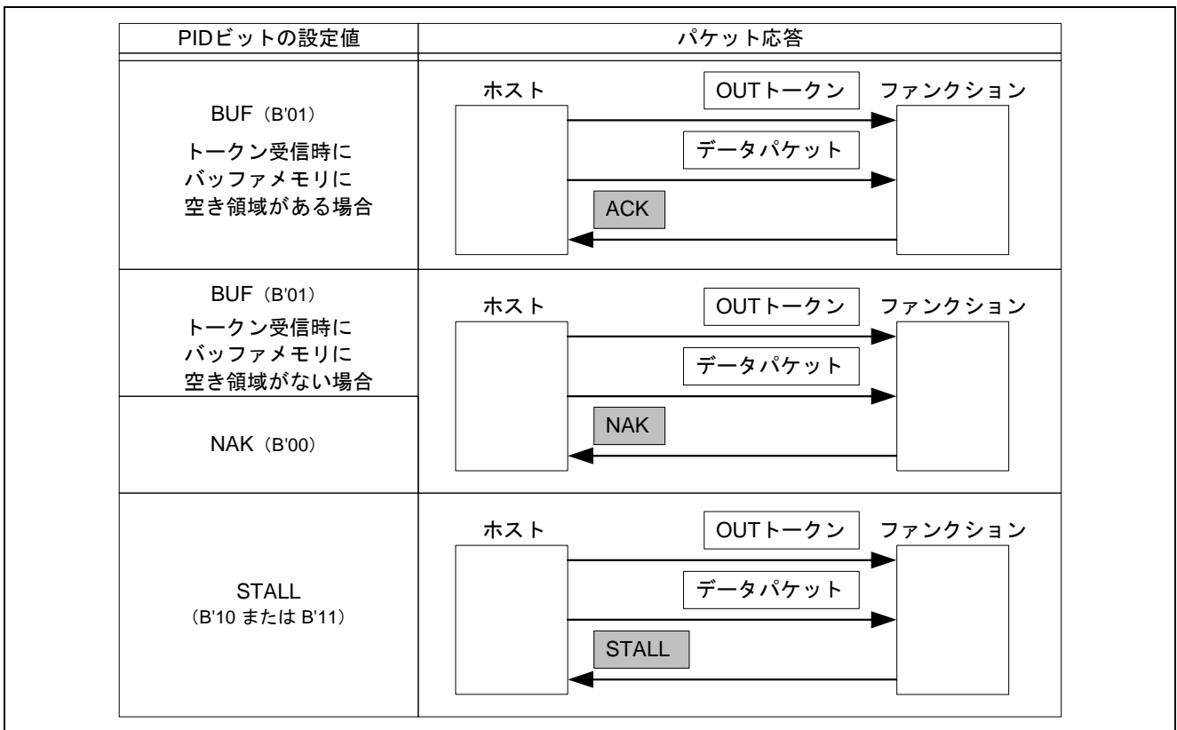
図3 インタラプト OUT 転送時のパケット応答パターン
