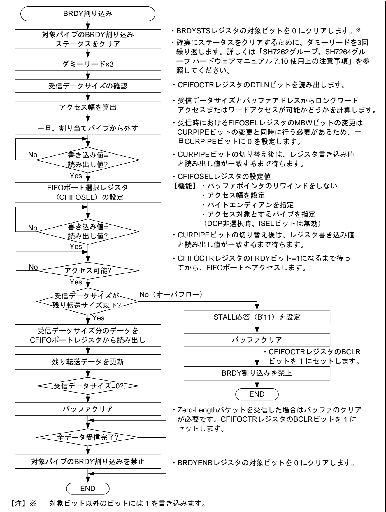
図19 BRDY 割り込み処理例
