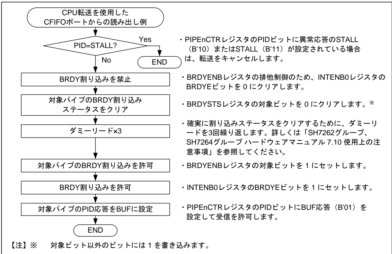
図18 FIFO ポートからの読み出し例
