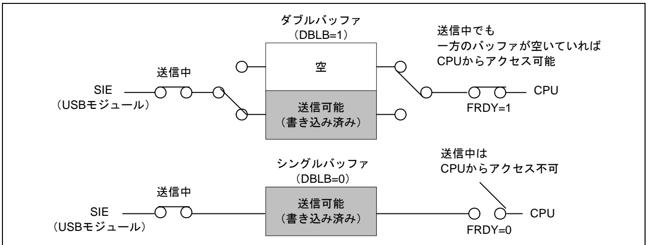
図8 ダブルバッファ
