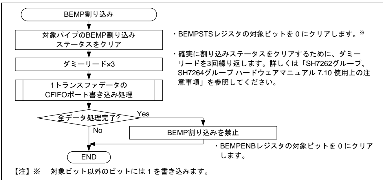
図17 BEMP 割り込み例
