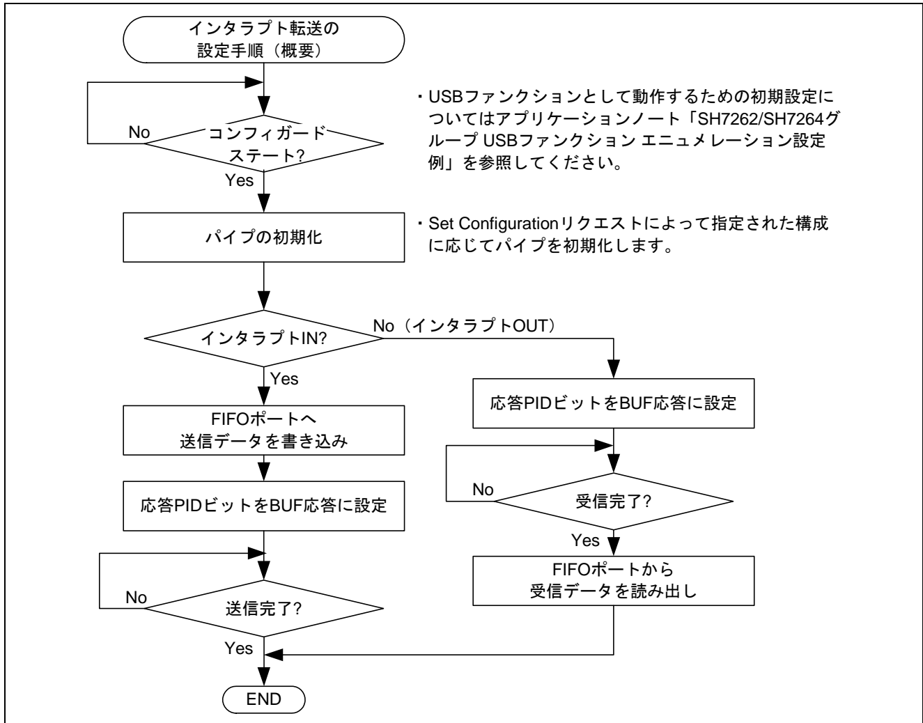
図4 インタラプト転送の設定手順（概要）
