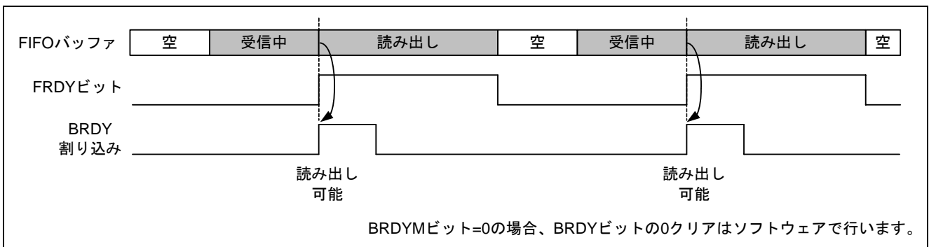
図13 受信動作の割り込み発生タイミング
