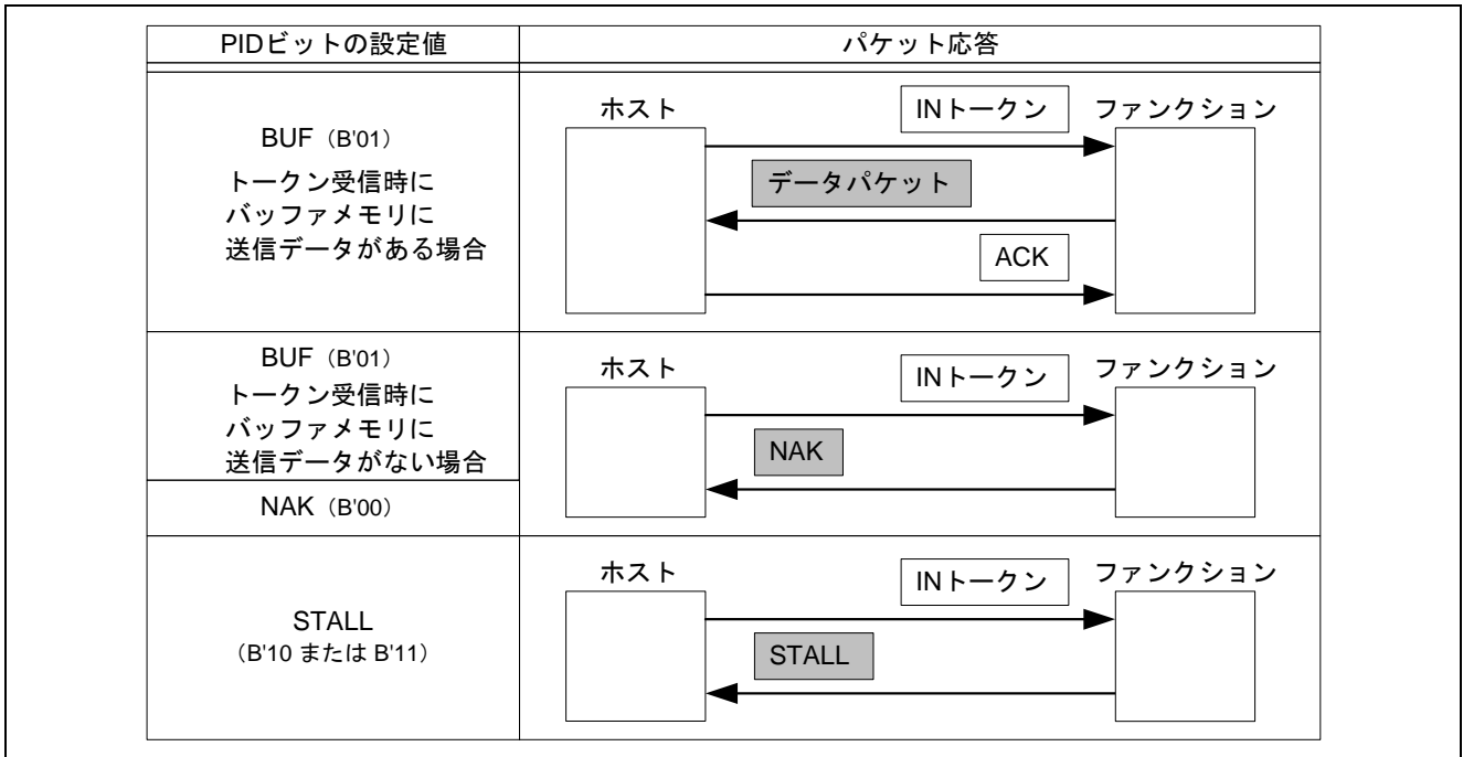
図2 インタラプト IN 転送時のパケット応答パターン
