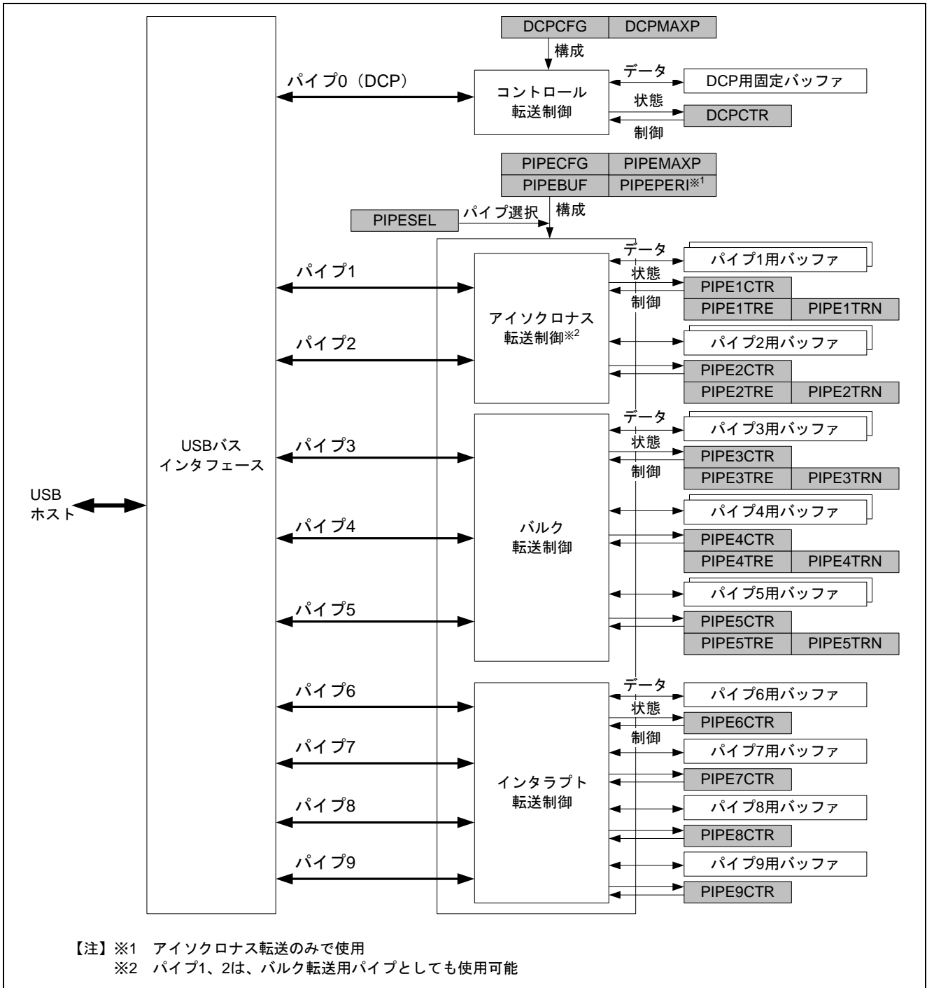
図5 パイプの概要
