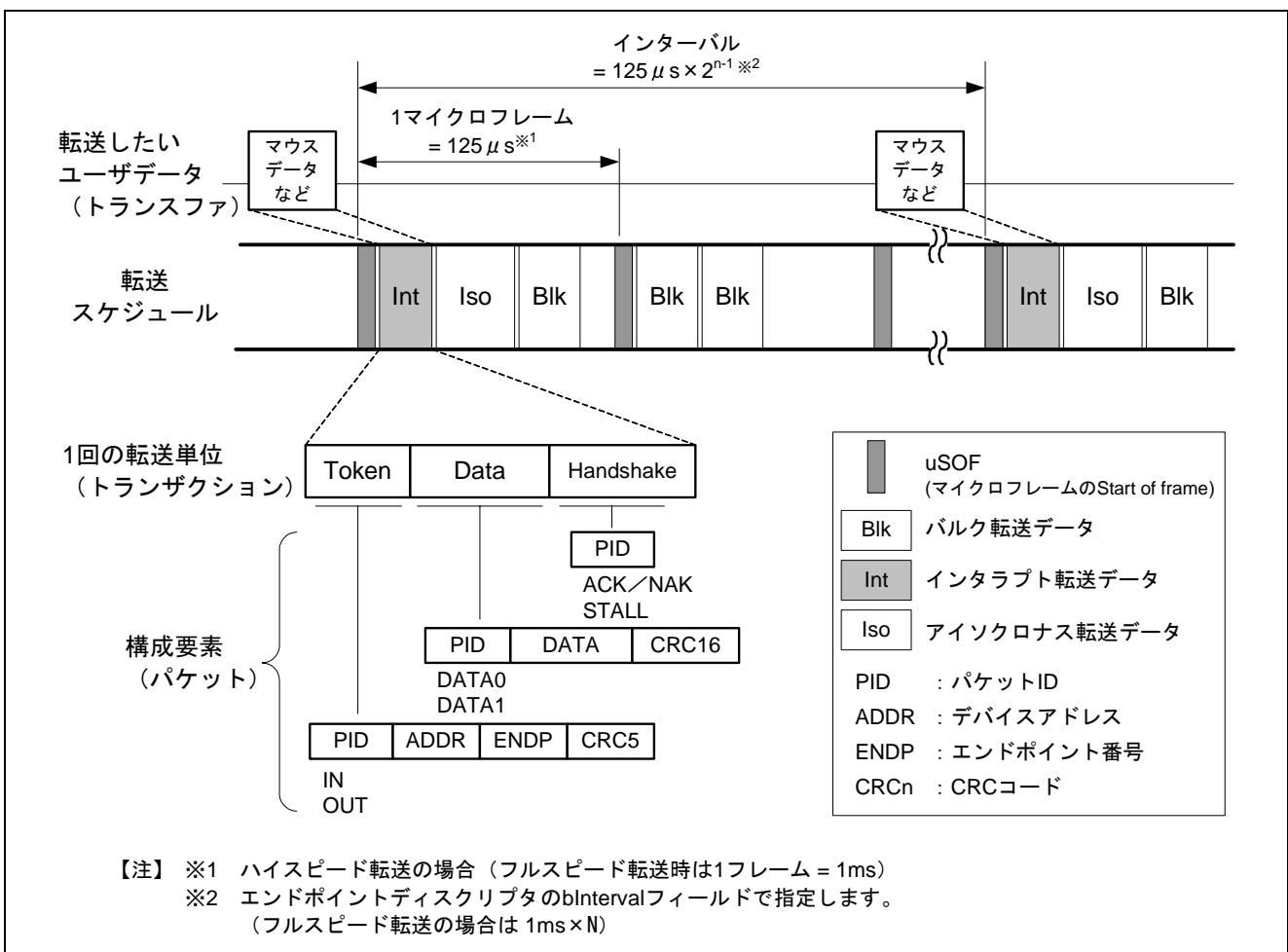
図 1 インタラプト転送の転送イメージ図
