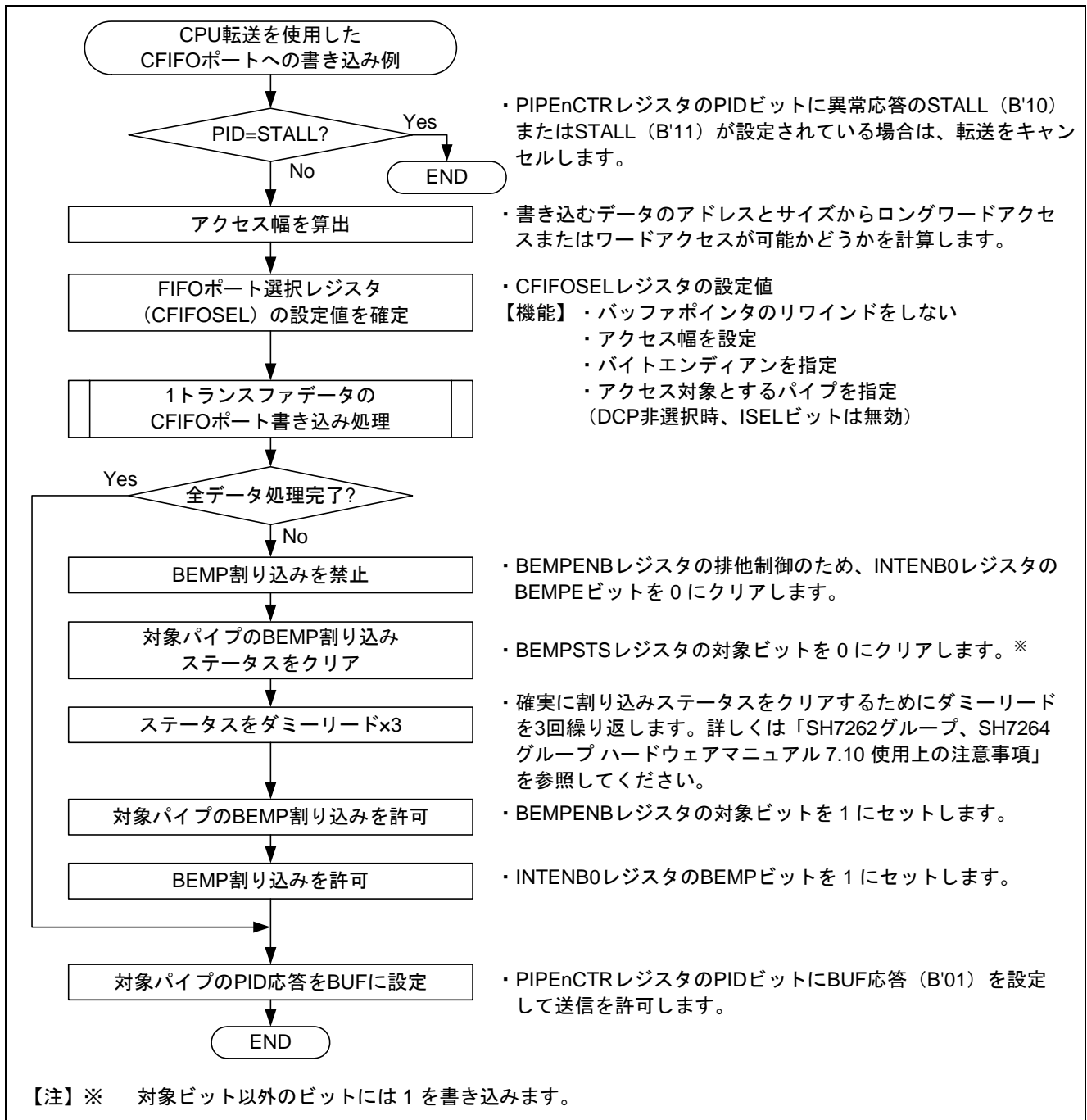
図15 FIFOポートへの書き込み例
