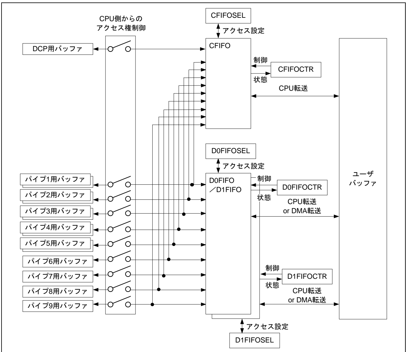
図14 FIFO ポートの概要
