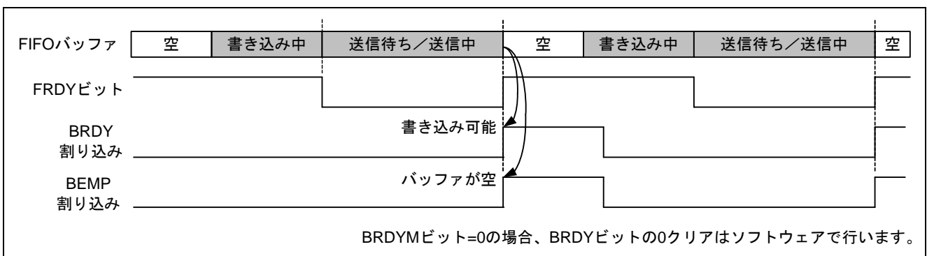
図11 送信動作の割り込み発生タイミング
