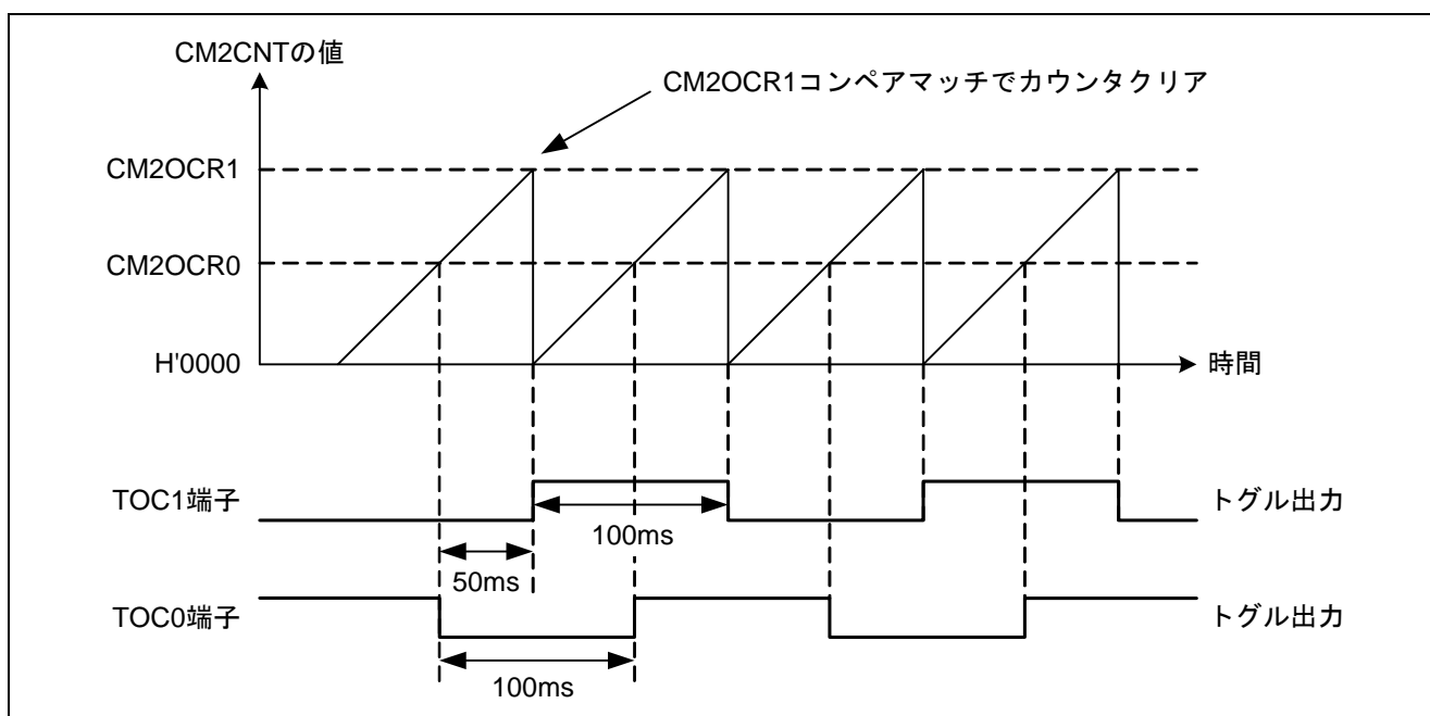
図 6.1 CMT2 アウトプットコンペア機能による矩形波出力例
