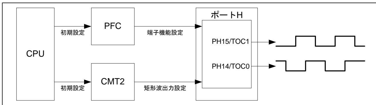
図 1.1 使用する周辺機能のブロック図
