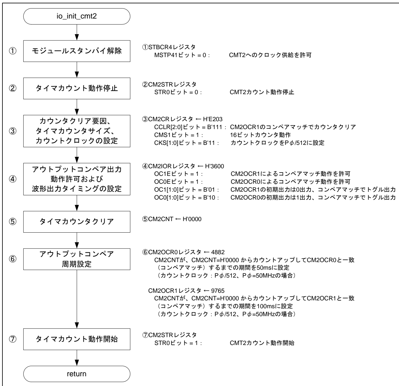
図 6.3 CMT2 設定処理 (io_init_cmt2 関数) フロー例
