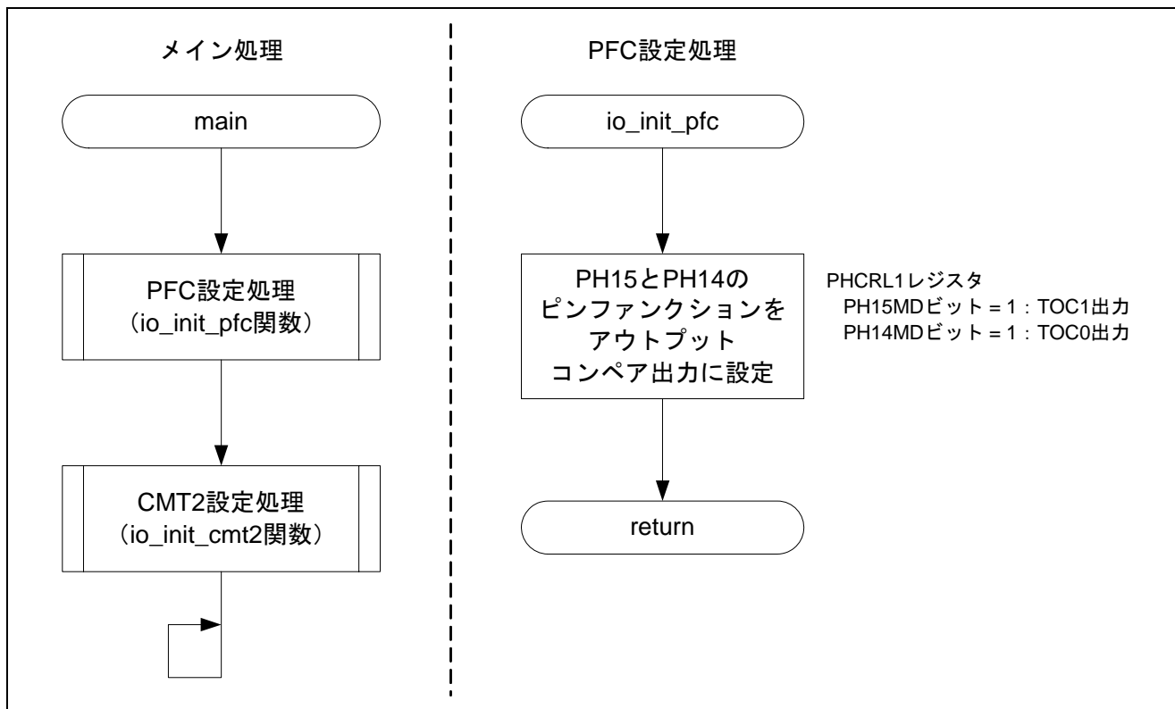
図 6.2 メイン処理 (main 関数) および PFC 設定処理 (io_init_pfc 関数) フロー例
