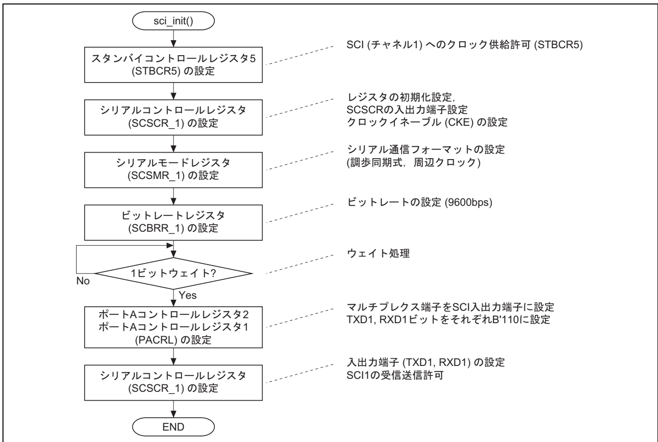
図 4 調歩同期式モード送信初期設定フロー
