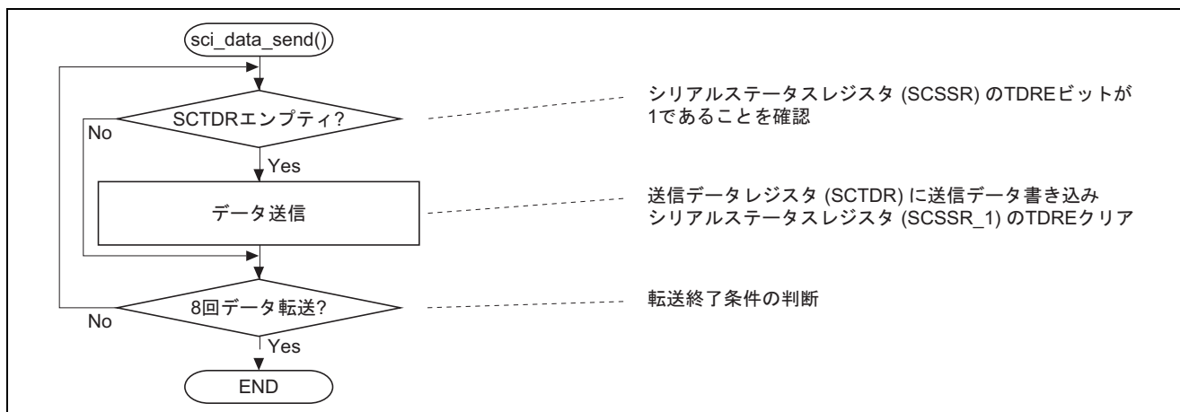
図 5 調歩同期式モード送信処理フロー
