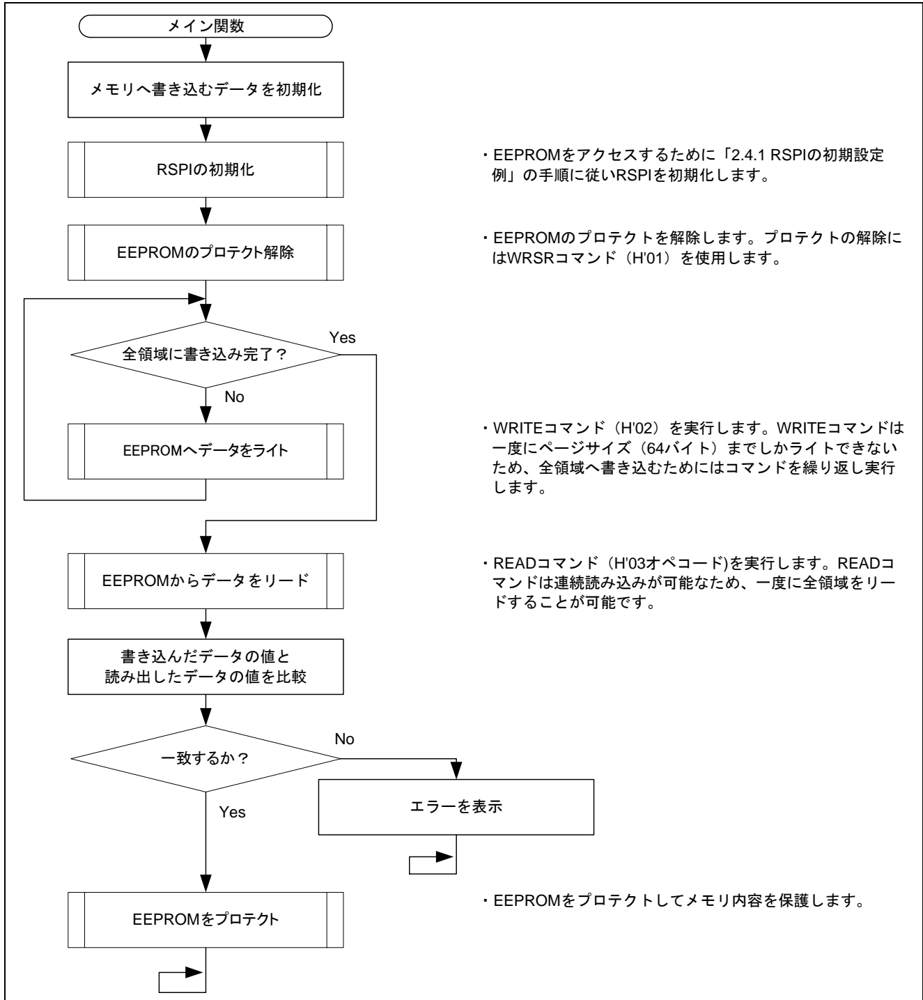
図8 参考プログラムのメイン関数フロー
