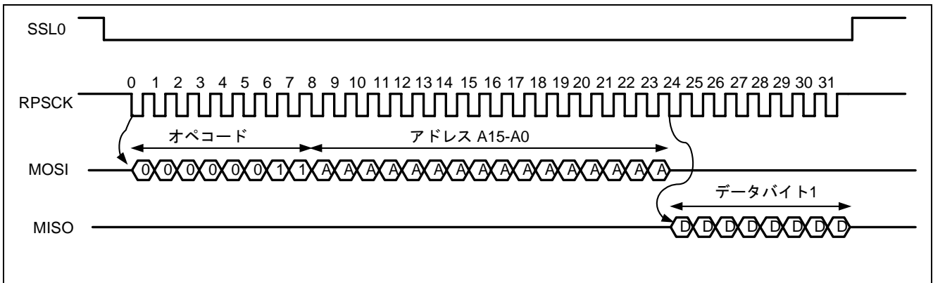
図5 リードコマンドシーケンス (H'03 オペコード)
