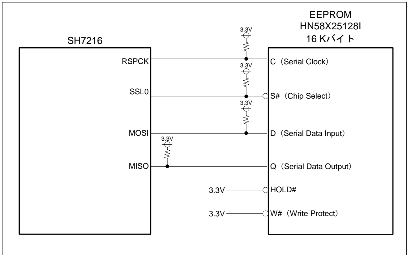
図1 EEPROM 接続回路例
