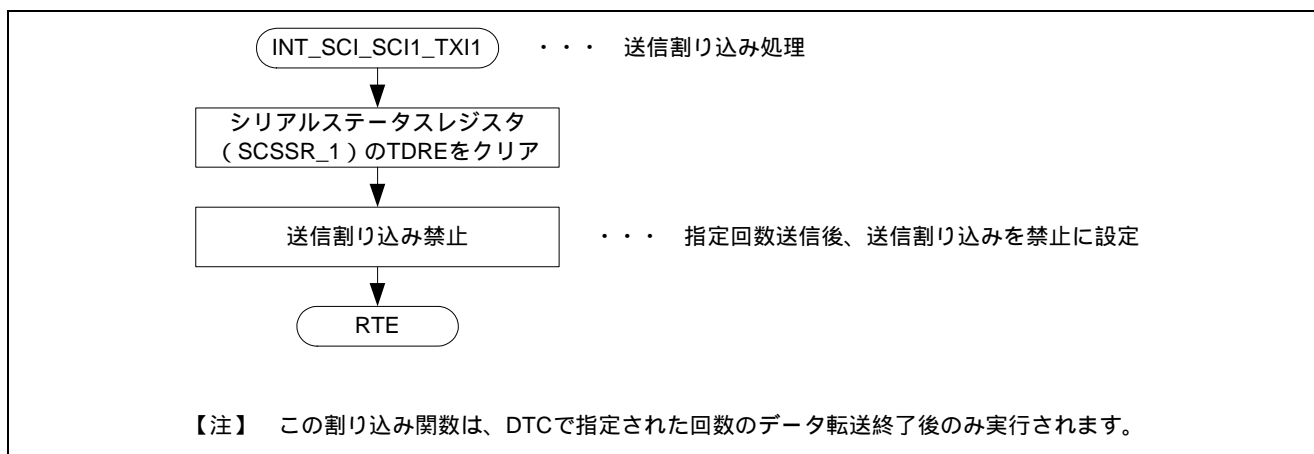
図 13 クロック同期式モード送信割り込み処理フロー
