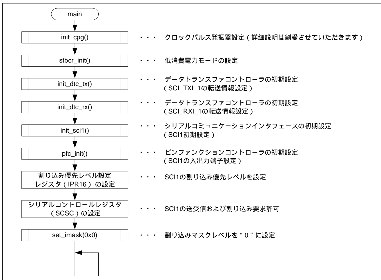
図 7 参考プログラム処理フロー
