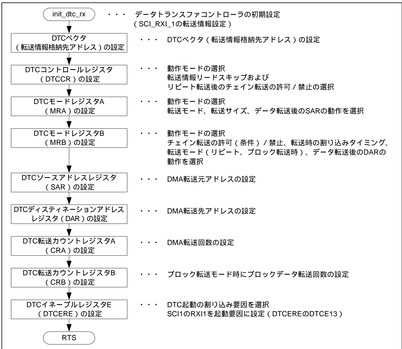
図 11 DTC の初期化フロー2
