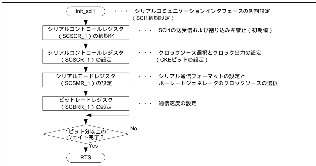
図 12 クロック同期式モード送受信初期設定フロー
