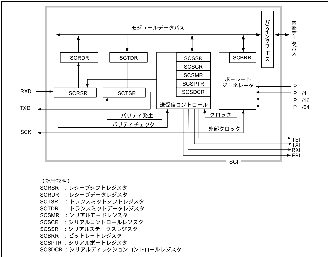
図 1 SCIF のブロック図
