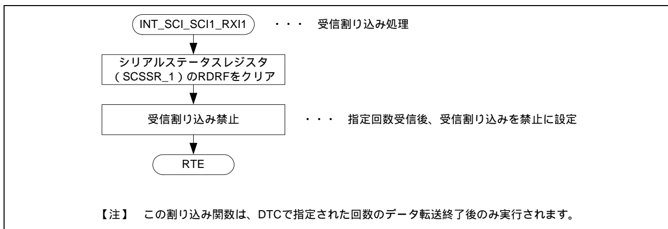
図 14 クロック同期式モード受信割り込み処理フロー
