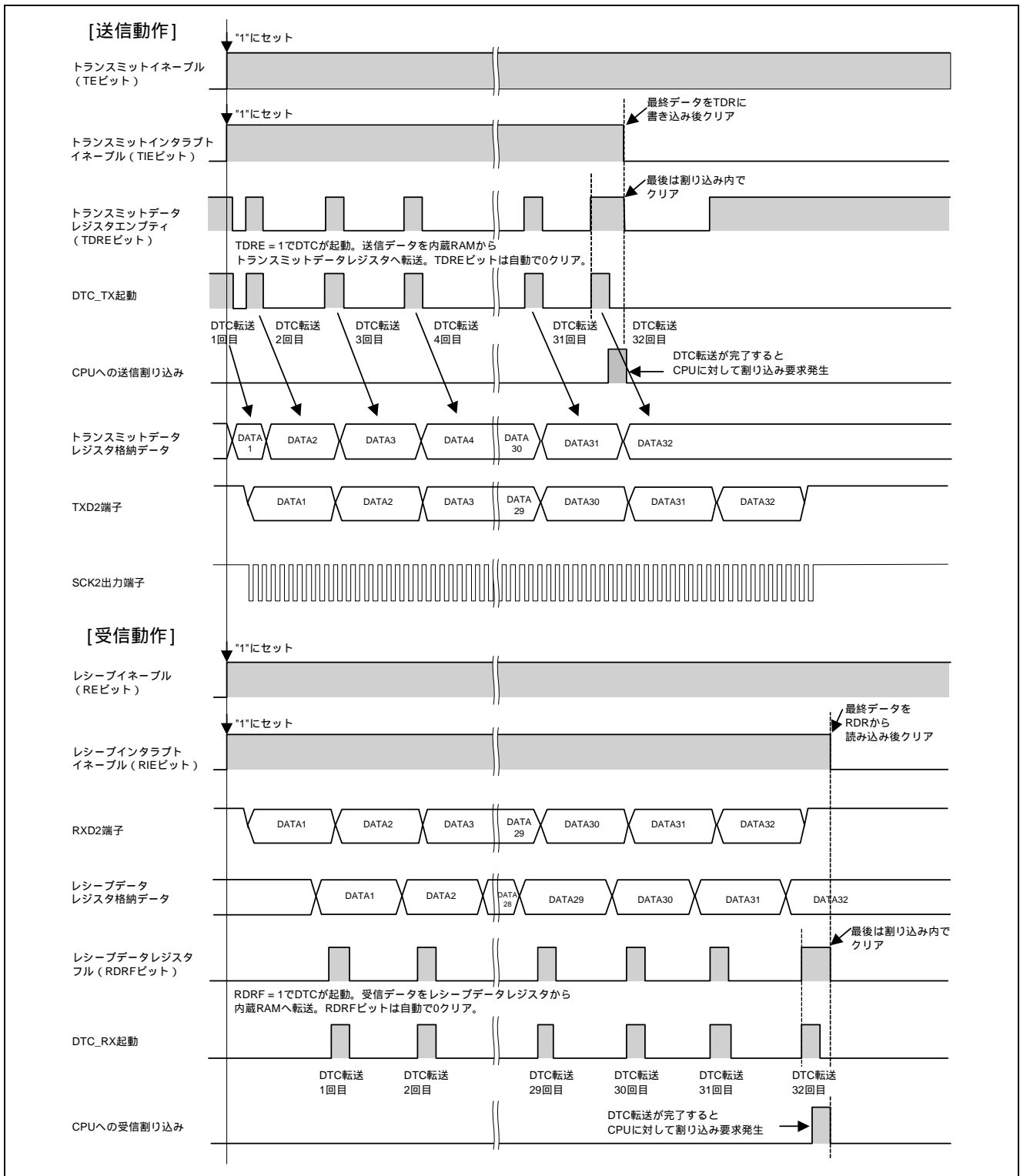
図 6 動作説明
