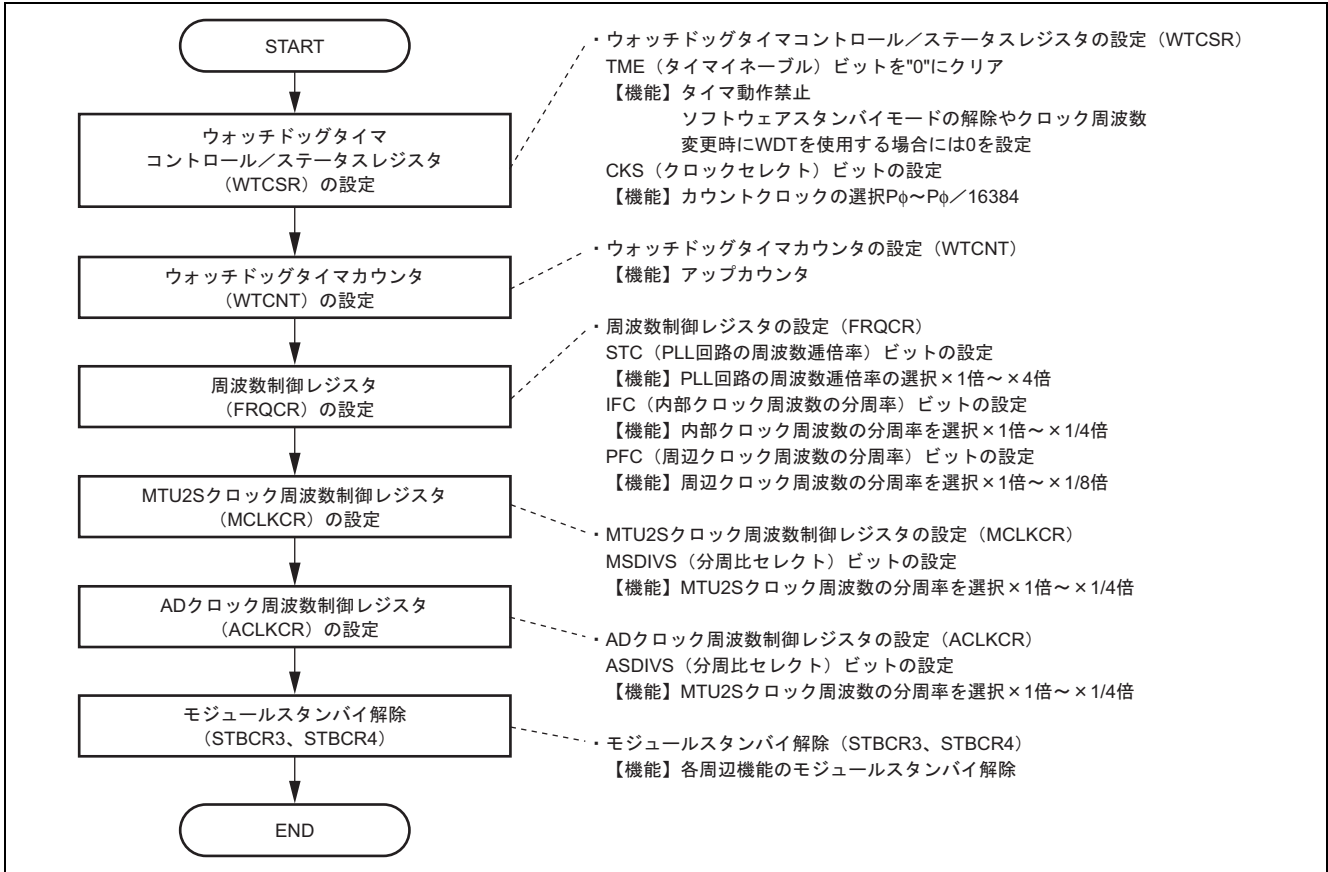
図3 動作周波数変更時のための設定フロー例
