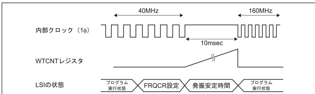
図 4 参考プログラムの動作タイミングイメージ図
