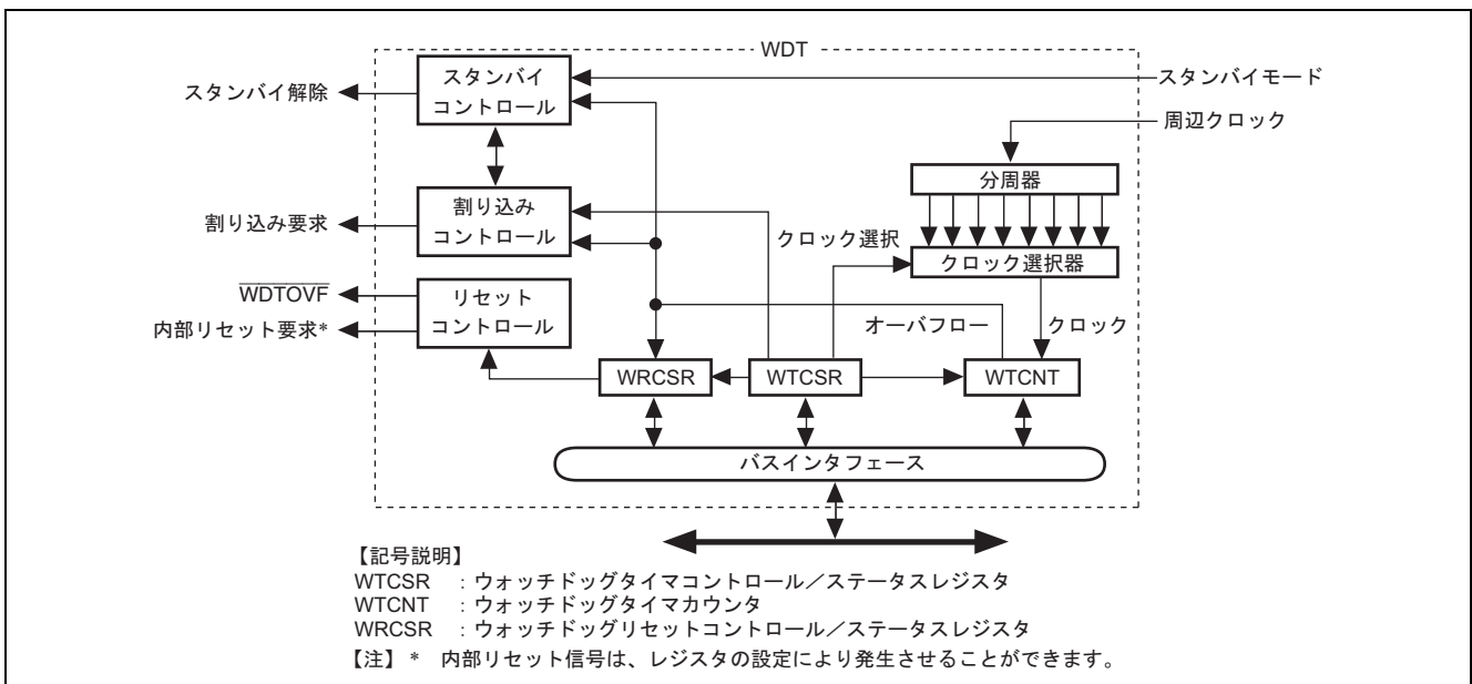
図2 WDTの概念図
