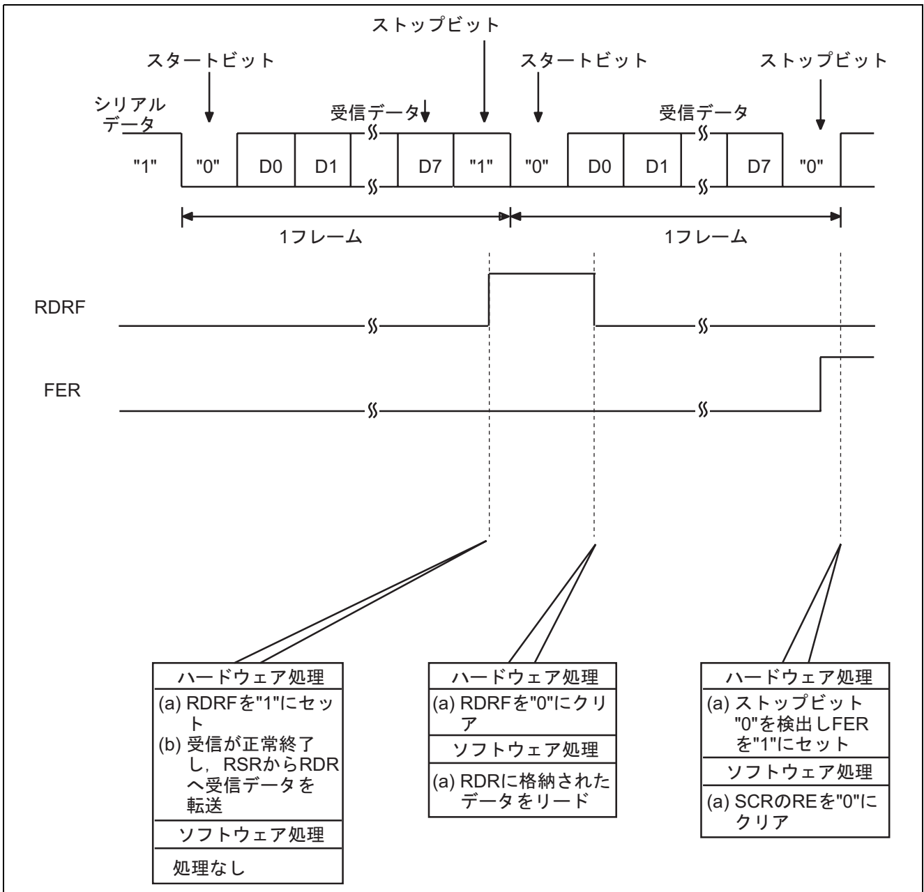
図3 調歩同期式シリアルデータ受信時の動作
