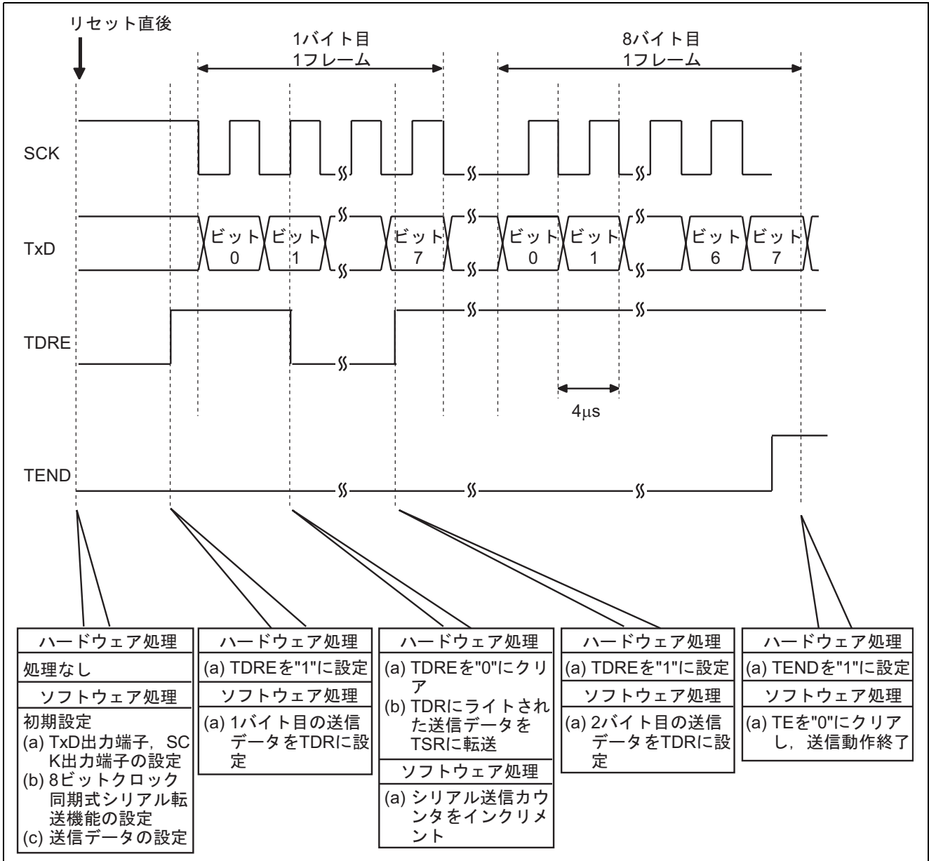
図3 クロック同期式シリアルデータ送信時の動作
