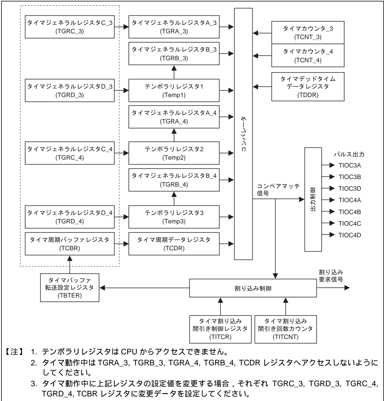
図2 割り込み間引き機能使用時のMTU2 (ch3, ch4) のブロック図
