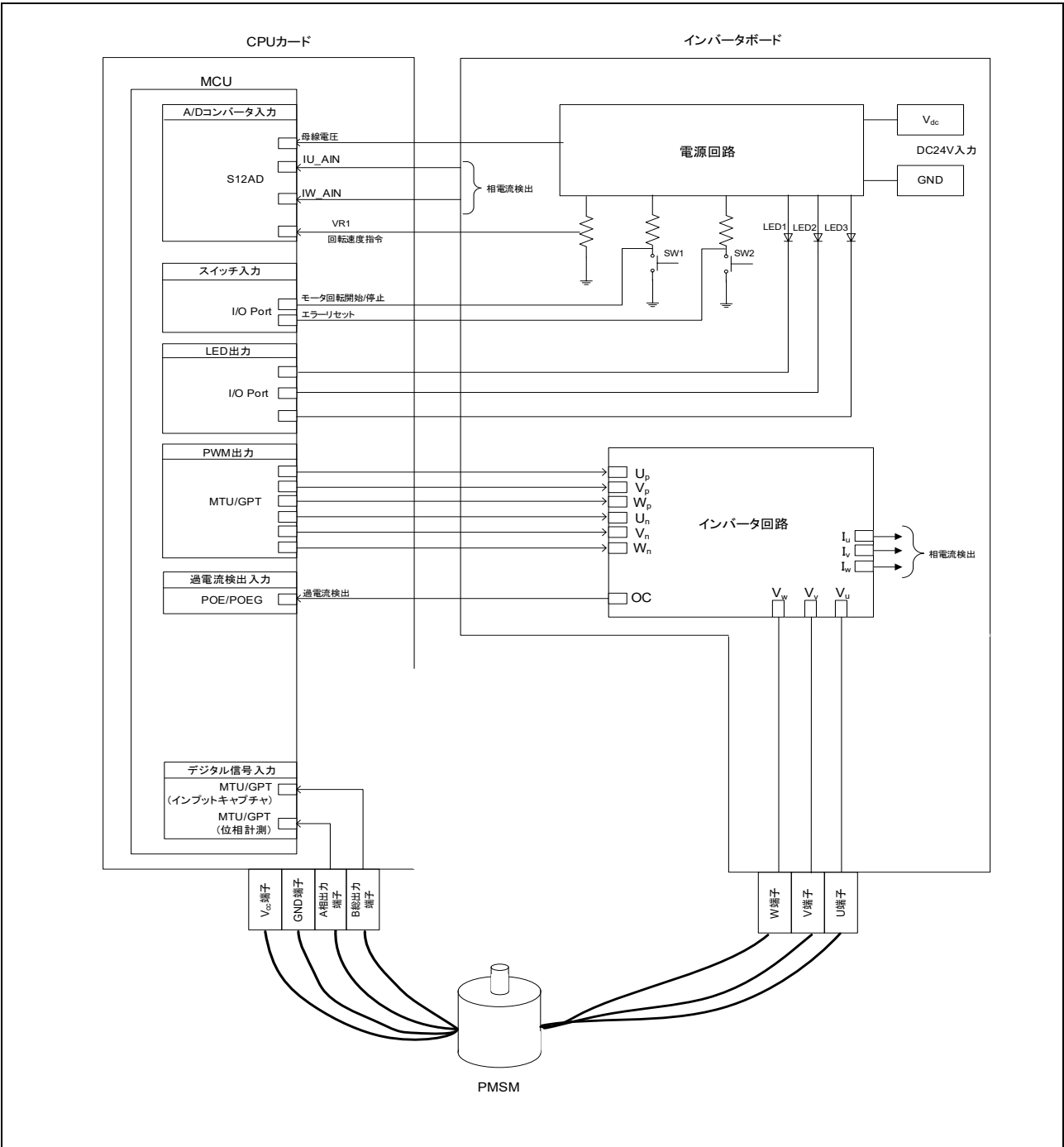
図 2-2 磁気センサ デジタル出力タイプハードウェア構成図
