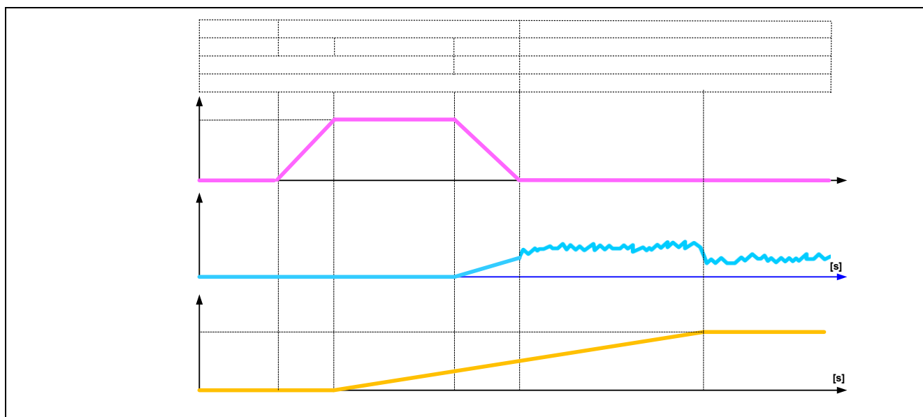
図 5-12 センサレスベクトル制御の始動制御内容
