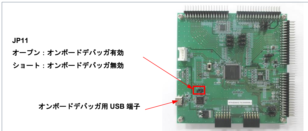
図 2-5 オンボードデバッグ
