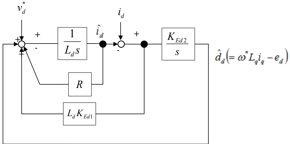
図 5-17 d 軸誘起電圧オブザーバブロック線図
