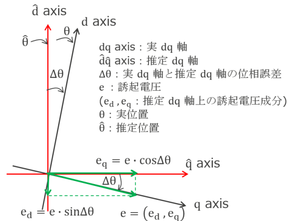
図 5-16 推定 dq 軸上の誘起電圧
