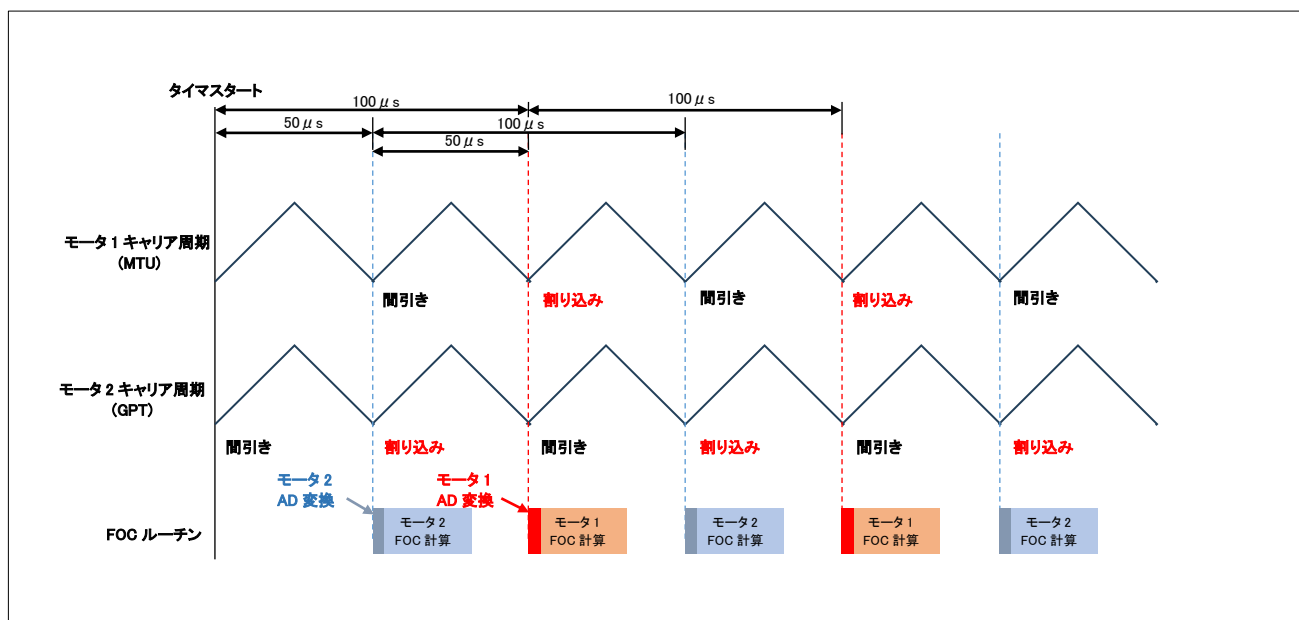
図 5-14 AD 変換完了割り込み周期
