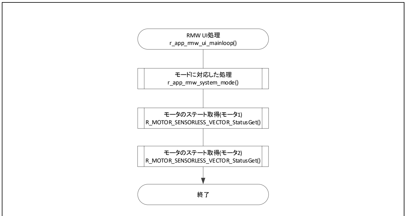
図 5-5 RMW UI 処理フローチャート
