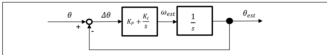
図 5-19 磁極位置推定系のブロック線図
