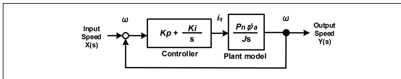
図 6-5 速度制御系のモデル
