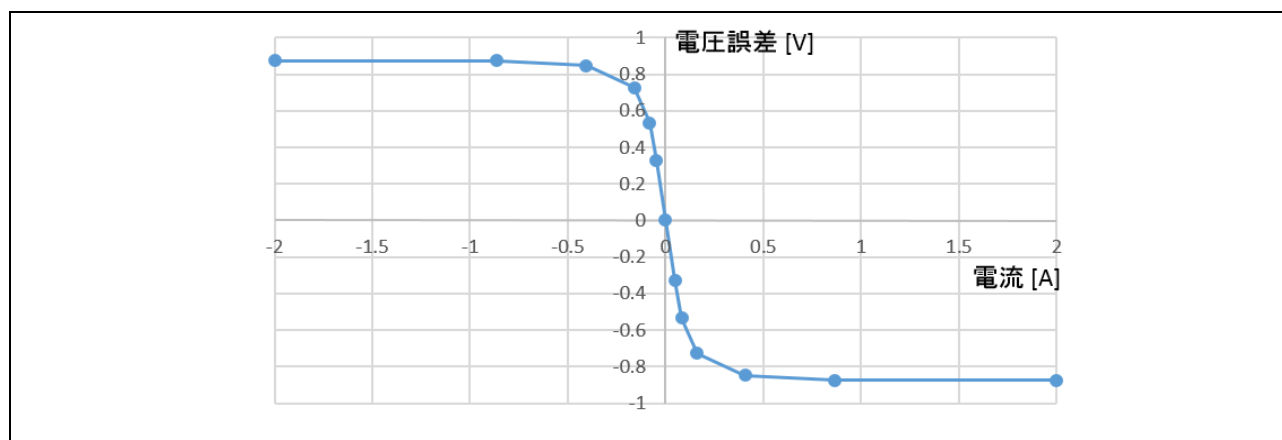
図 5-15 電圧誤差の電流依存性(一例)
