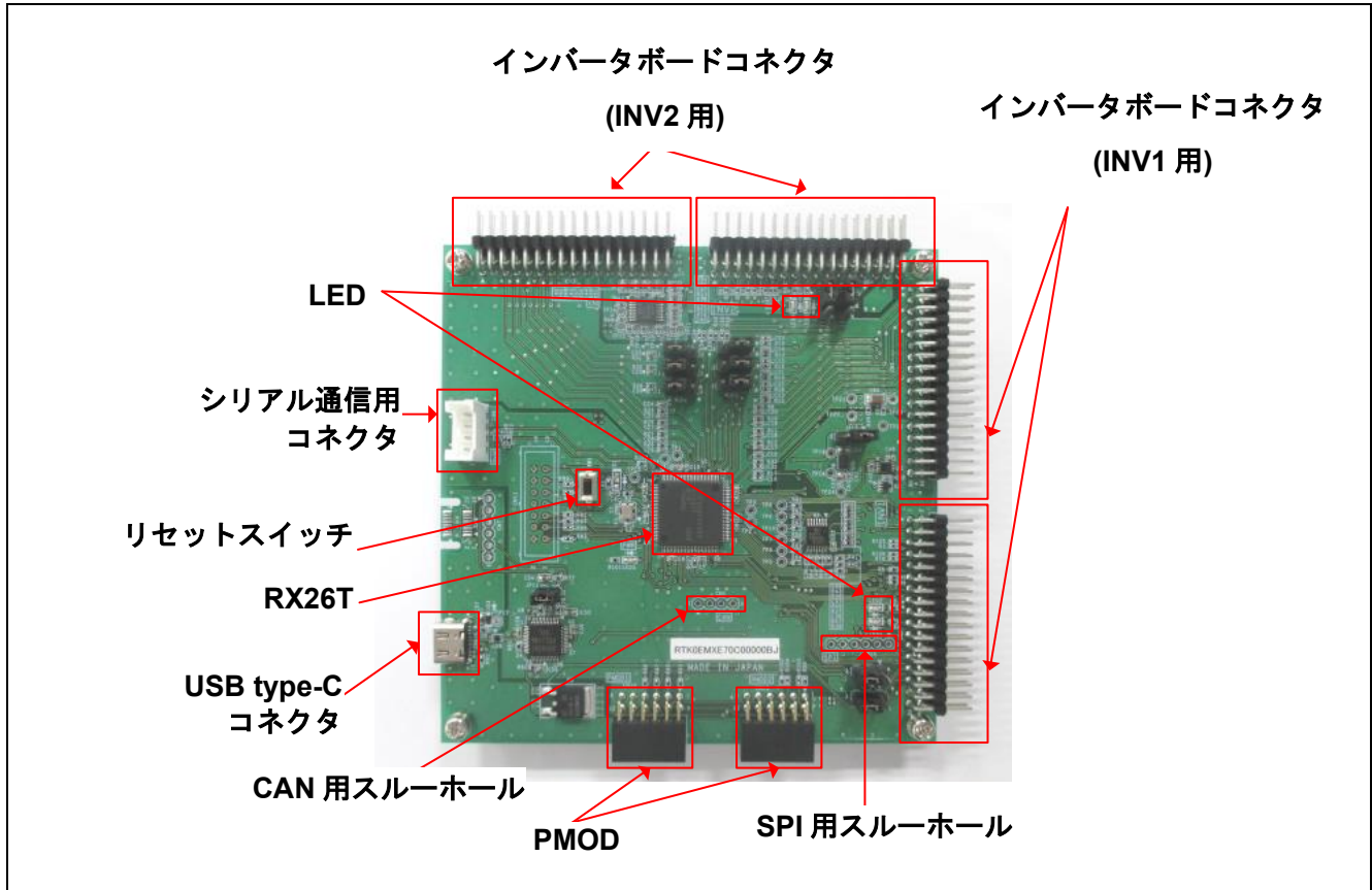
図 2-4 RX26T CPU ボードとインタフェース
