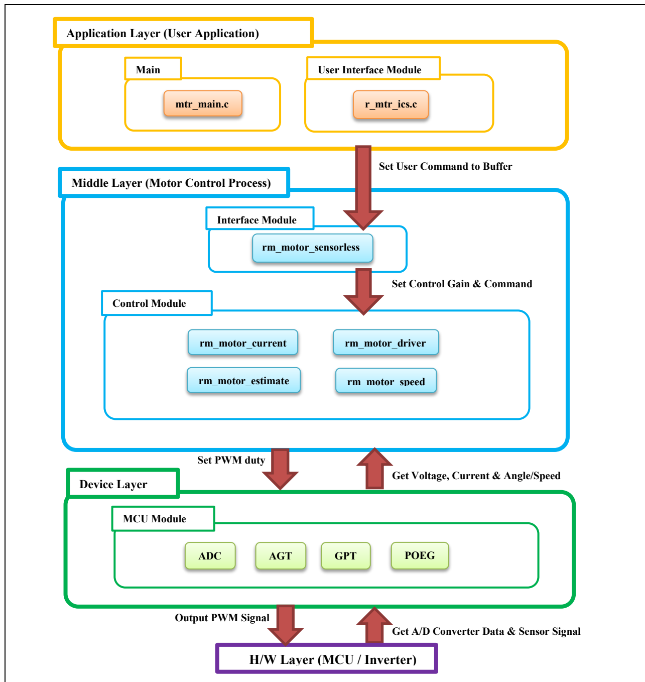
図 2-34 モジュール構成
