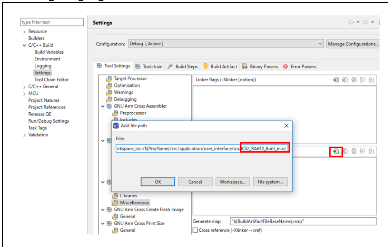
図 4-15 ICS2_RA6T2_Built_in.o を登録
