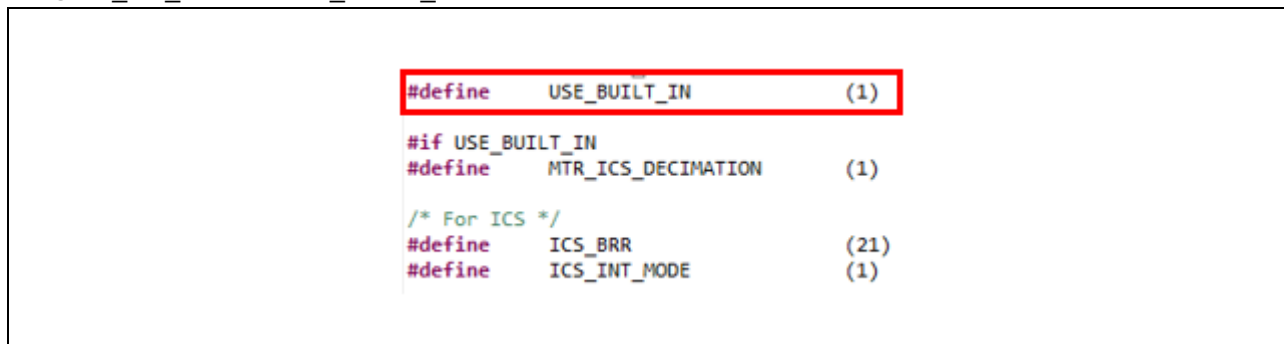
図 4-16 r_mtr_ics.h の修正
