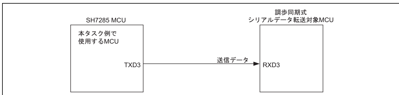
図 1 SCIF 調歩同期式シリアルデータ送信
