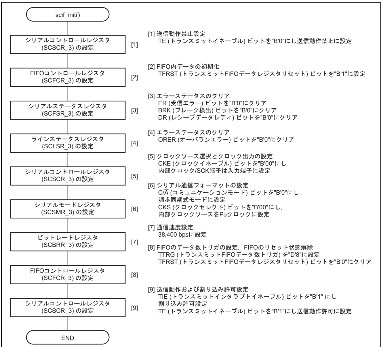
図6 調歩同期式モード送信初期設定フロー
