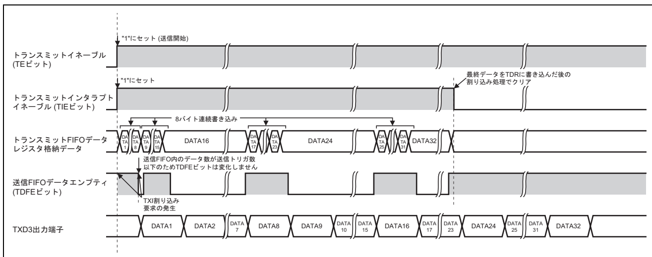
図 3 送信動作説明図
