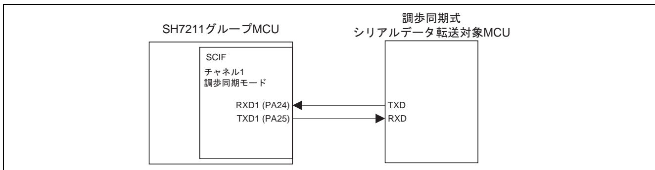
図 1 FIFO 付き調歩同期式シリアルデータ送受信動作
