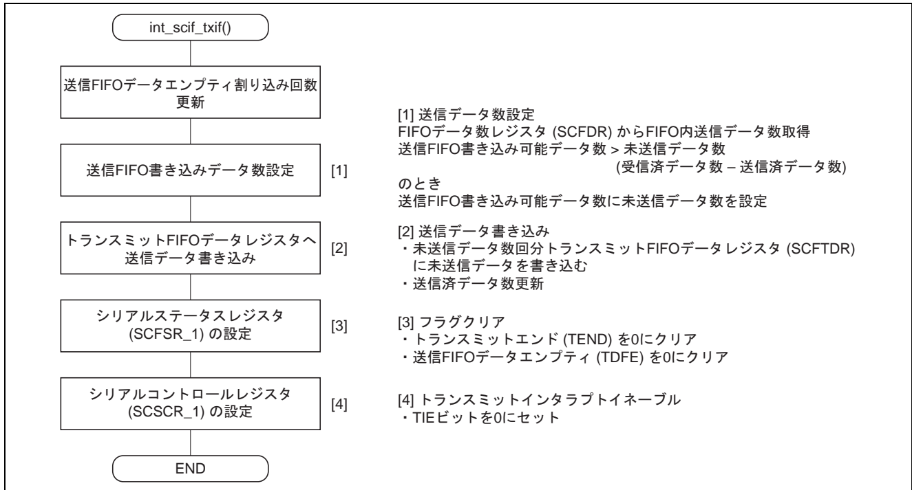
図 11 SCIF 送信 FIFO データエンプティ割り込み関数の処理フロー
