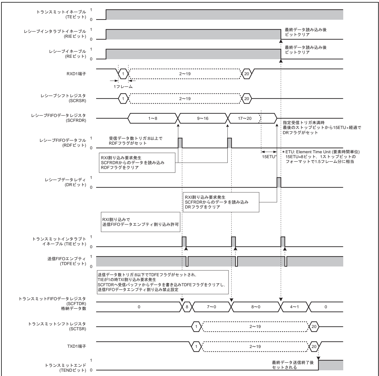
図3 送受信動作
