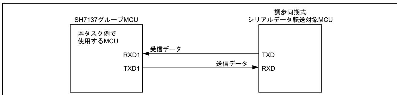
図 1 SCI 調歩同期式シリアルデータ送受信例
