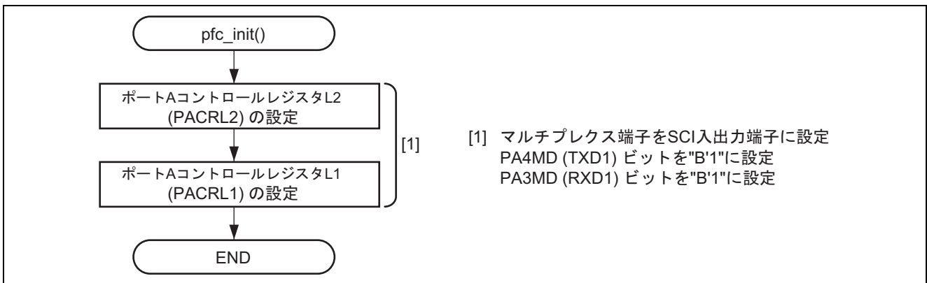
図6 ピンファンクションコントローラの設定フロー
