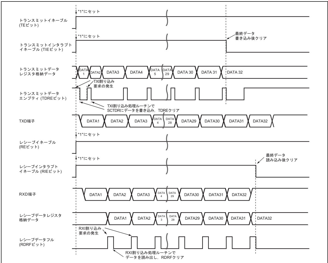
図 3 送受信動作説明
