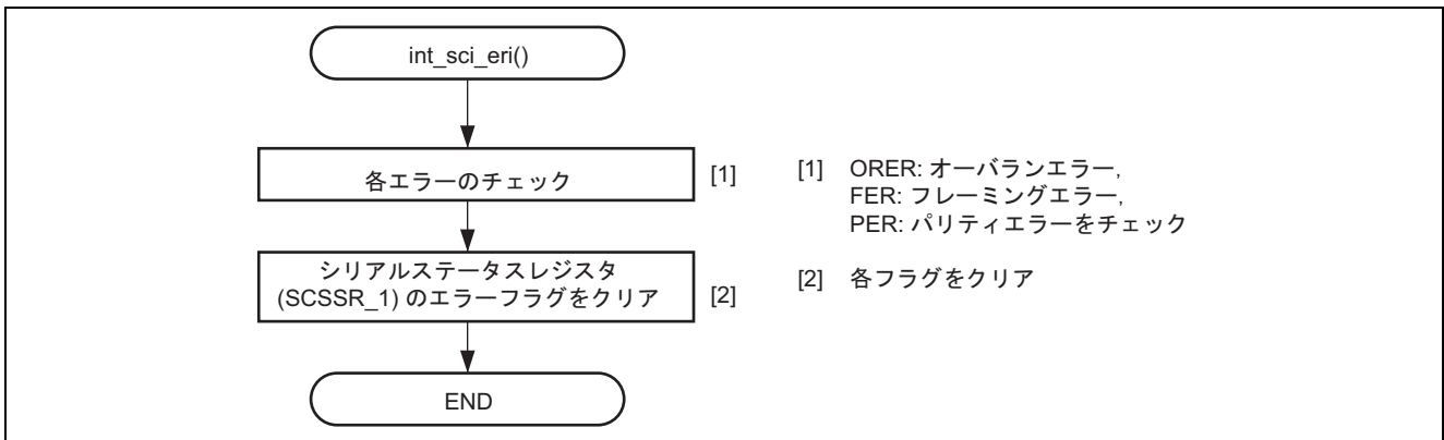
図 9 受信エラー割り込み処理フロー
