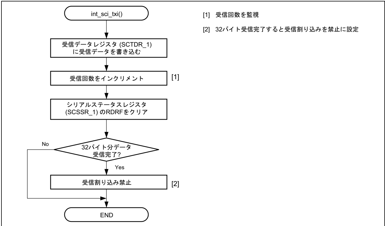
図 8 調歩同期式モード受信割り込み処理フロー
