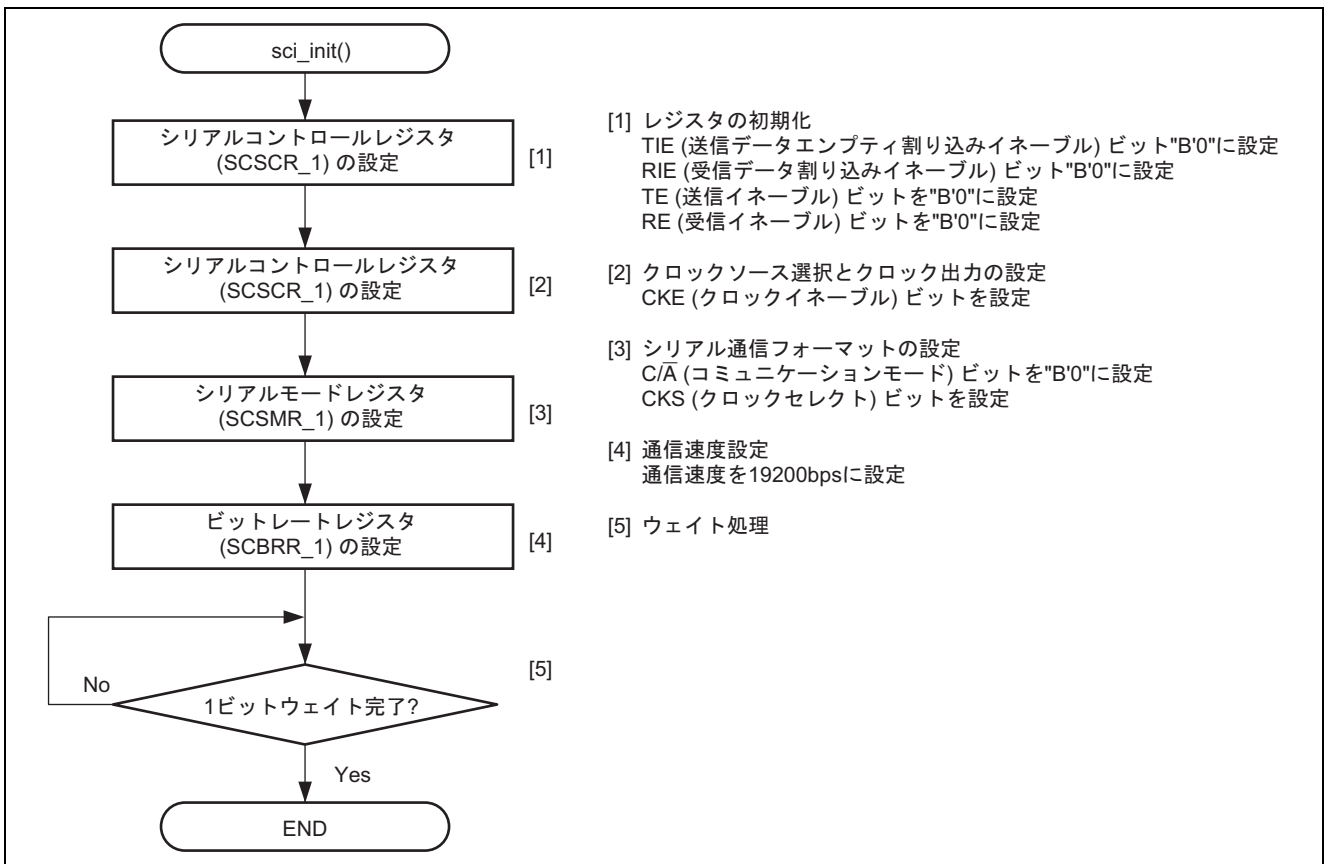
図7 調歩同期式モード受信初期設定フロー
