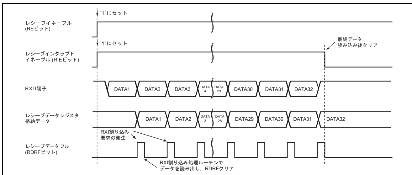
図 3 受信動作説明
