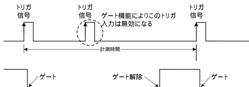
入力パルス波形
