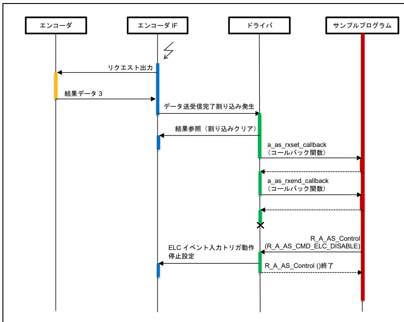
図 4-14 ELC イベントトリガ動作のシーケンス図 (2/2)
