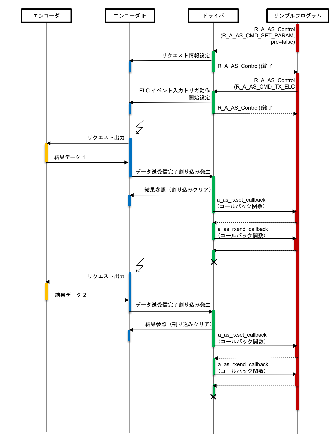
図 4-13 ELC イベントトリガ動作のシーケンス図 (1/2)
