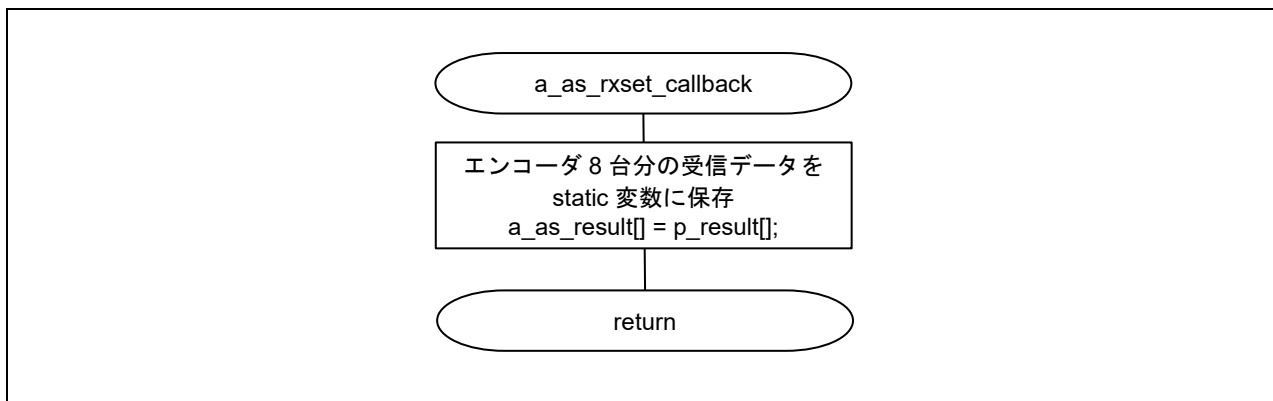
図 4-8 a_as_rxset_callback 関数のフローチャート
