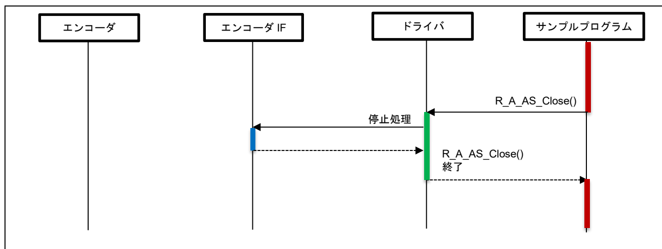
図 4-15 停止シーケンス図
