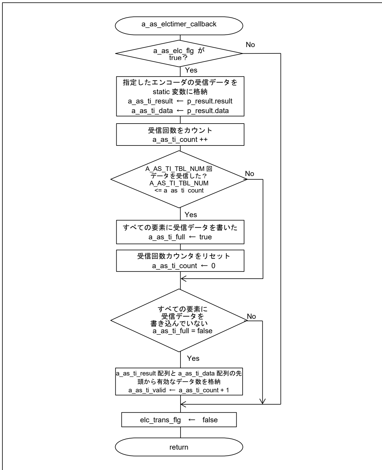
図 4-10 a_as_elctimer_callback 関数のフローチャート
