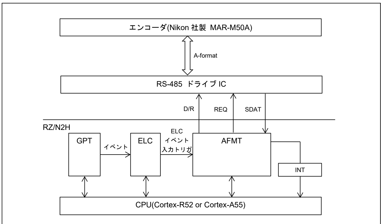
図 4-1 システムブロック図
