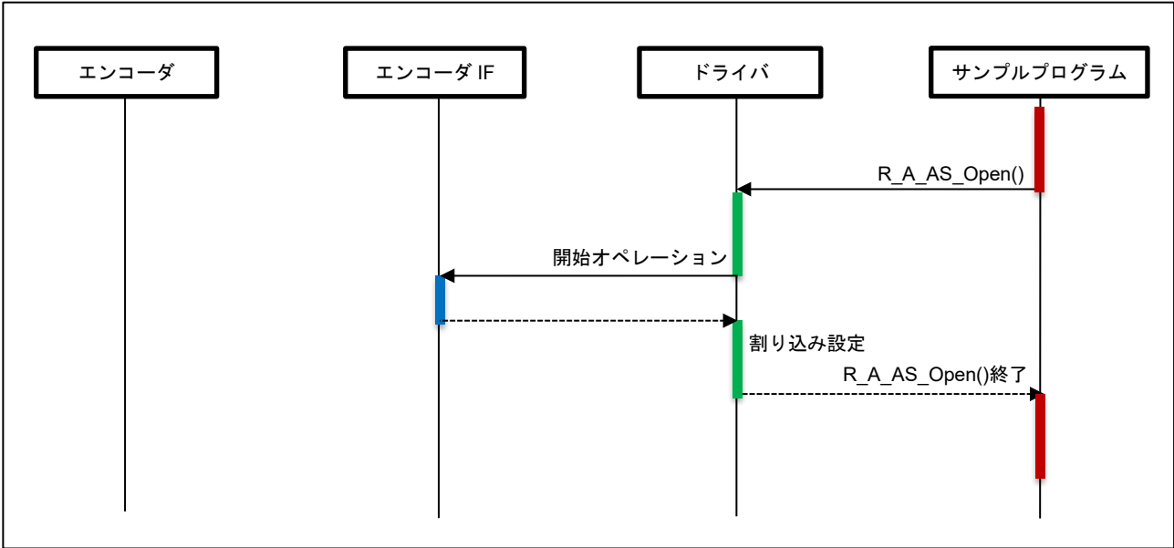
図 4-11 開始シーケンス図
