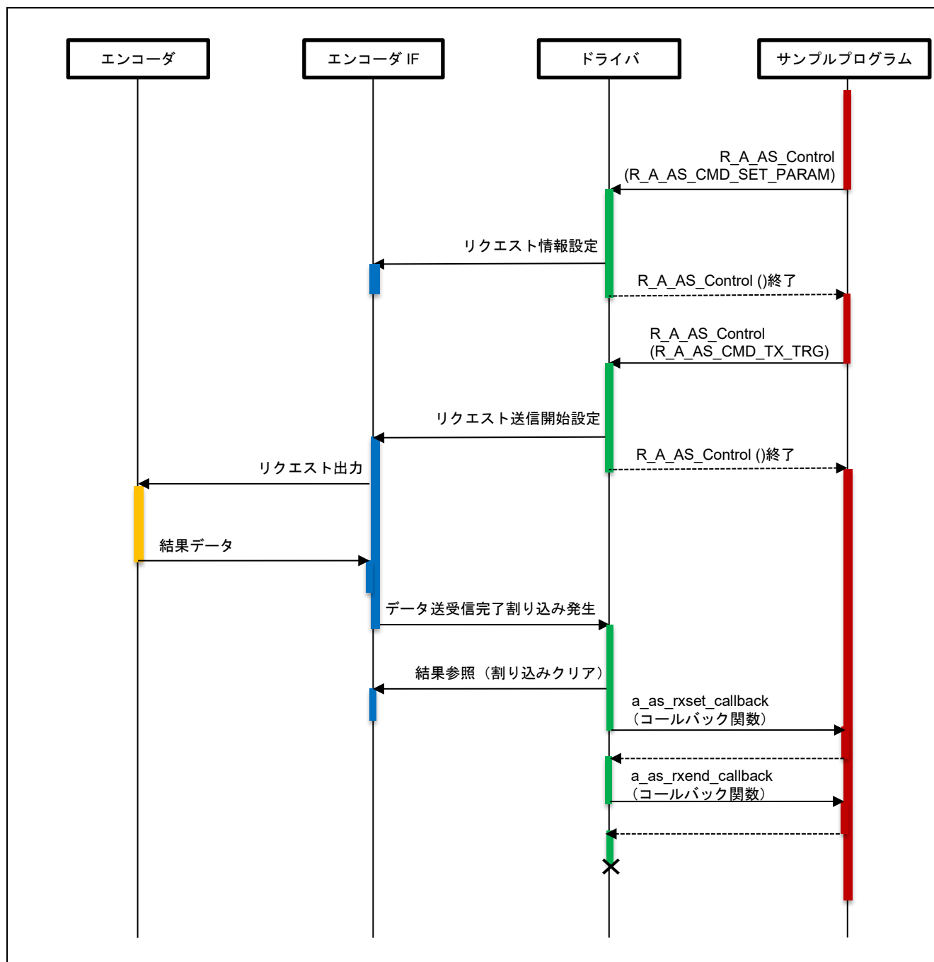
図 4-12 リクエスト送信とデータ受信のシーケンス図
