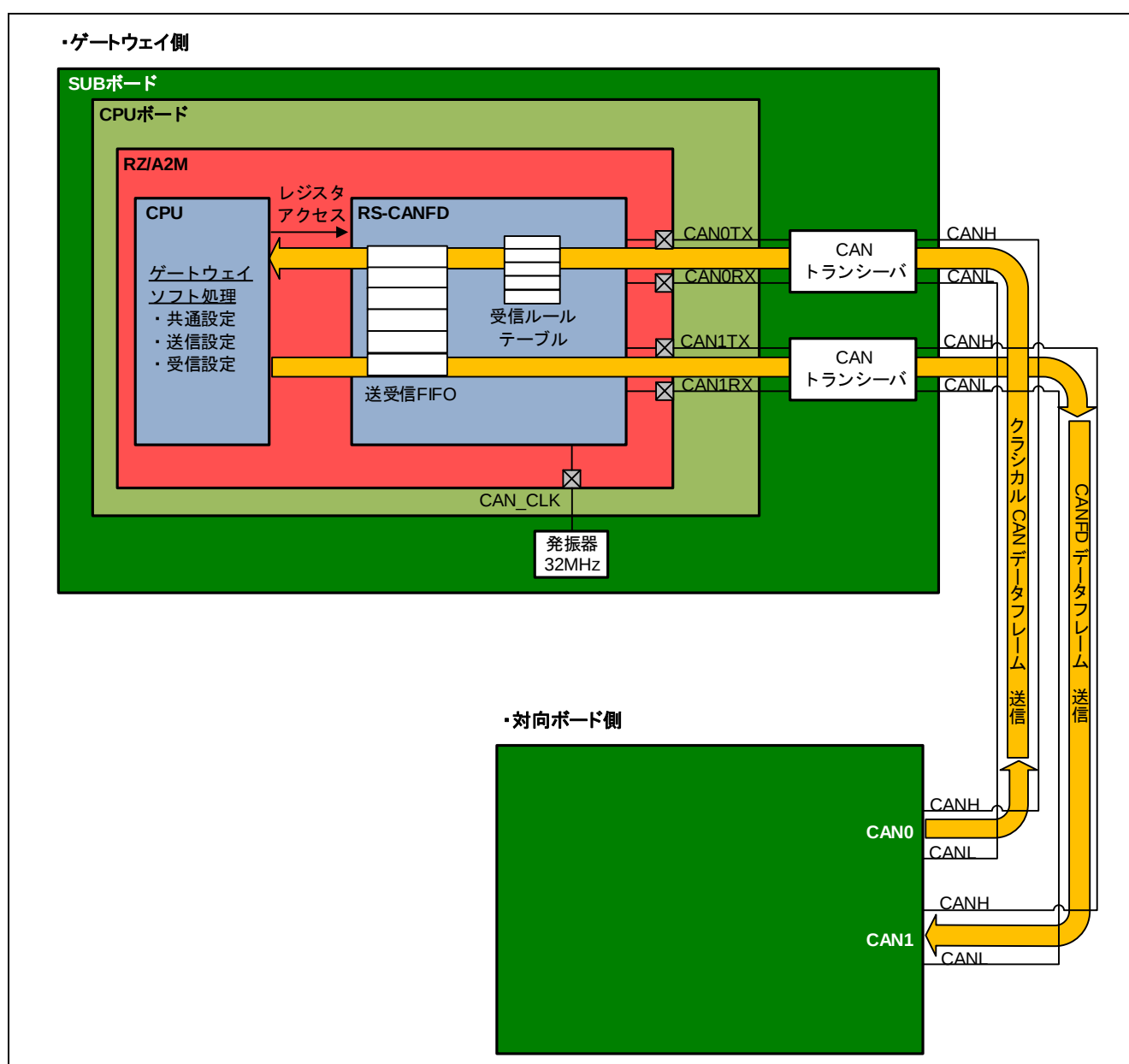
図 3-7 システム構成
