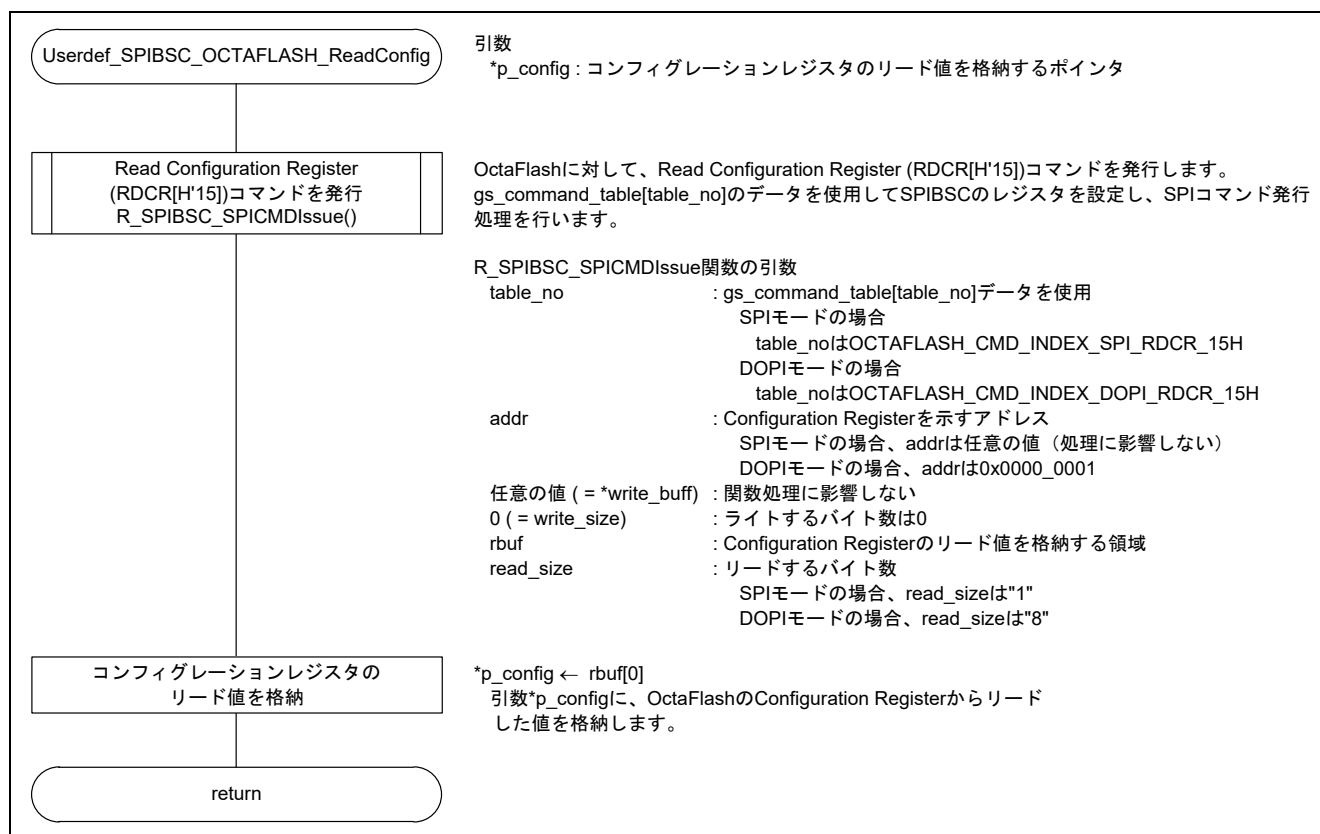
図6.11 Userdef_SPIBSC_OCTAFLASH_ReadConfig 関数のフロー
