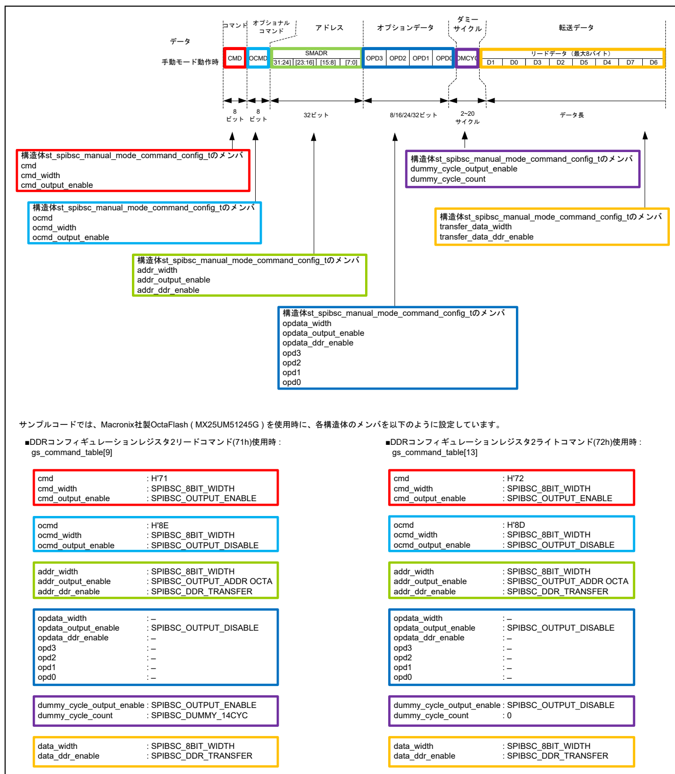
図6.5 SPIBSC レジスタと手動モード時に OctaFlash に出力される波形の関係
