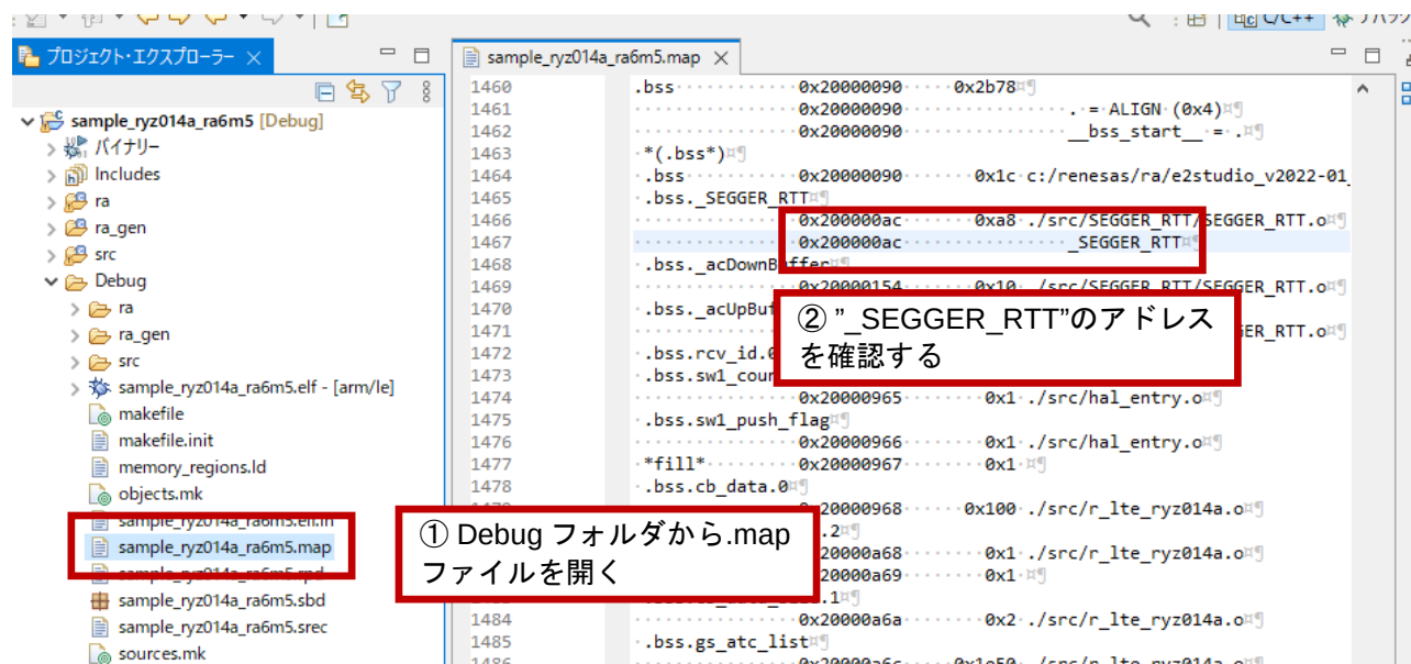
図 2.5 .map ファイルの確認
