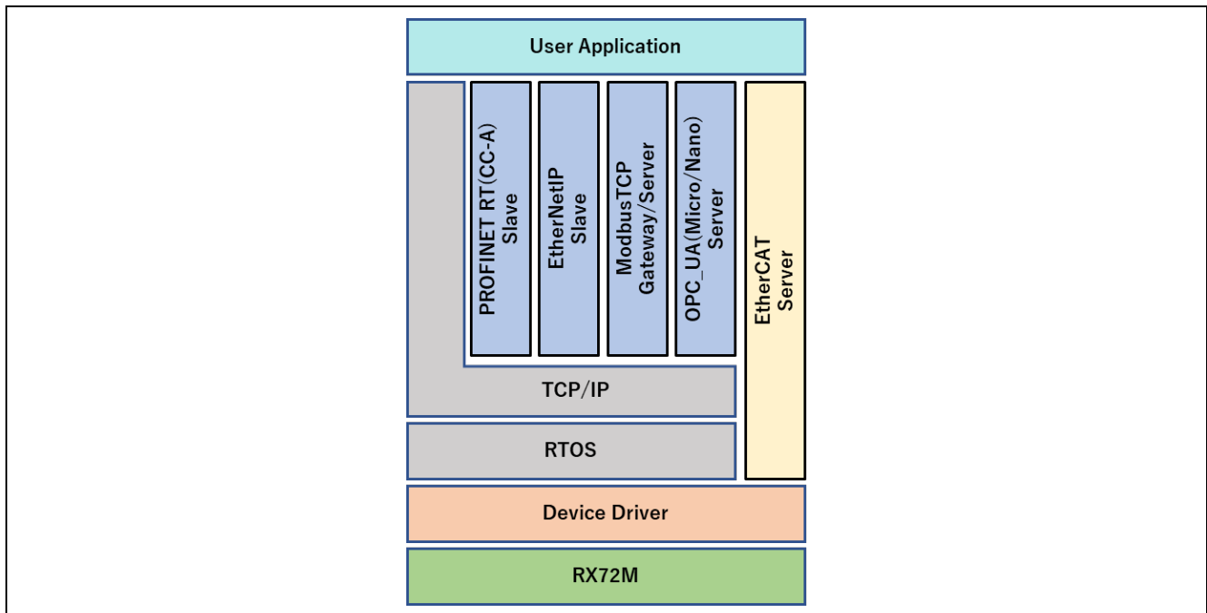
図 2.1 RX72M プロトコルスタックソフトウェア全体構成
