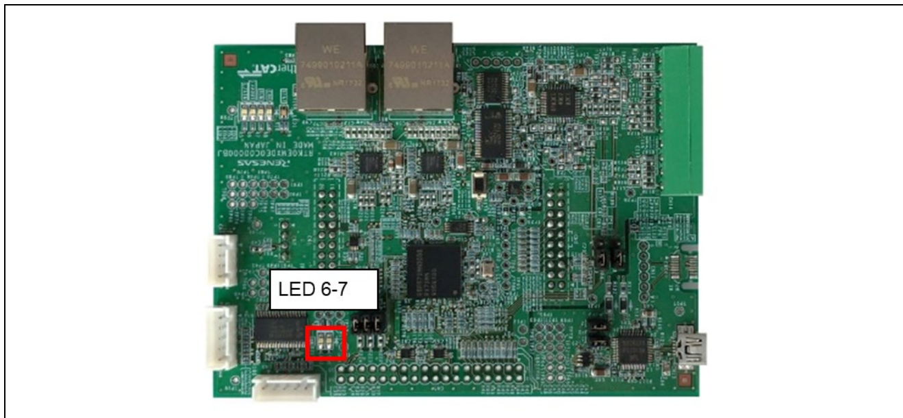
図 6.9 サイクリック伝送受信確認用 LED
