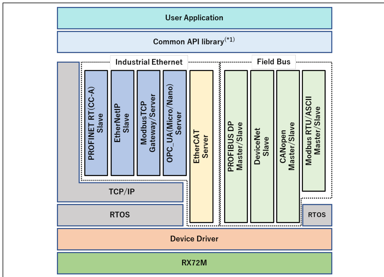
図 2.1 RX72M プロトコルスタックソフトウェア全体構成
