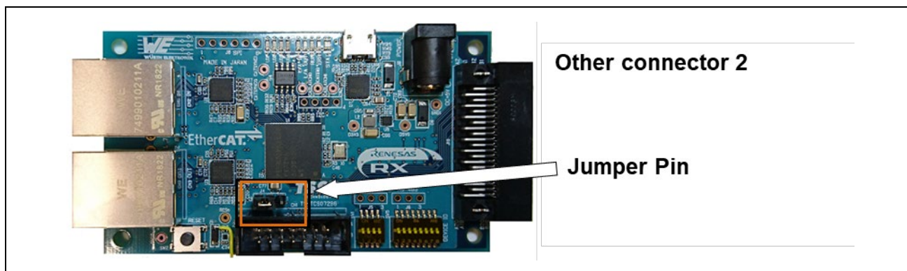
図 1-2 ジャンパーピン設定
