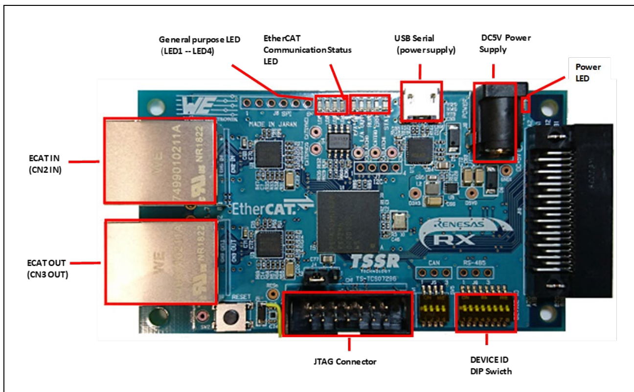
図 1-1 RX72M 通信ボード構成
