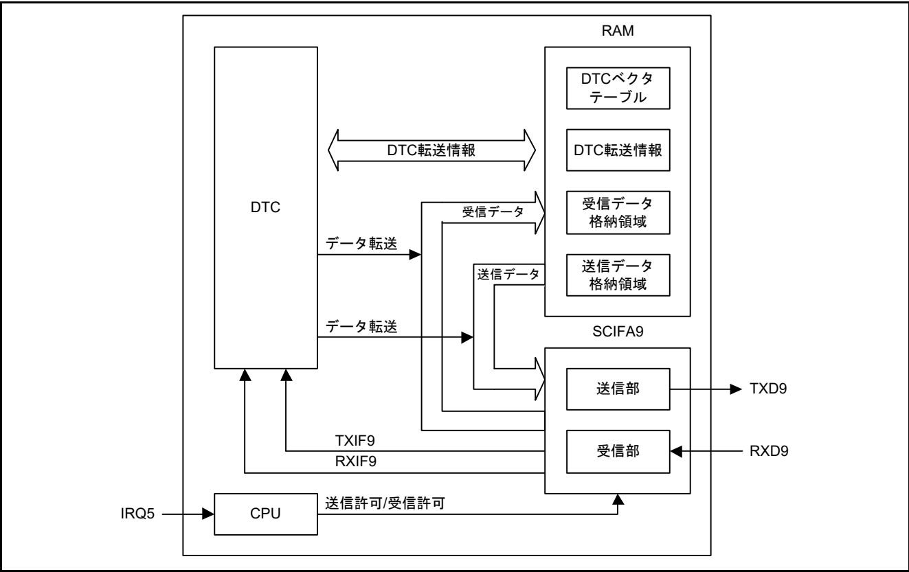
図 1.1 ブロック図
