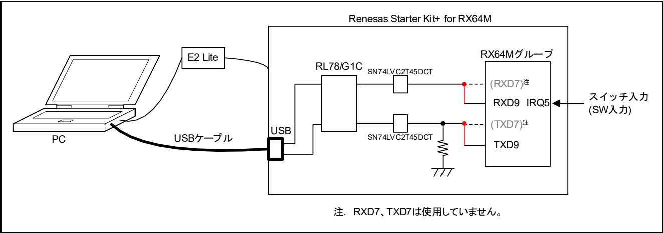
図 4.1 接続例
