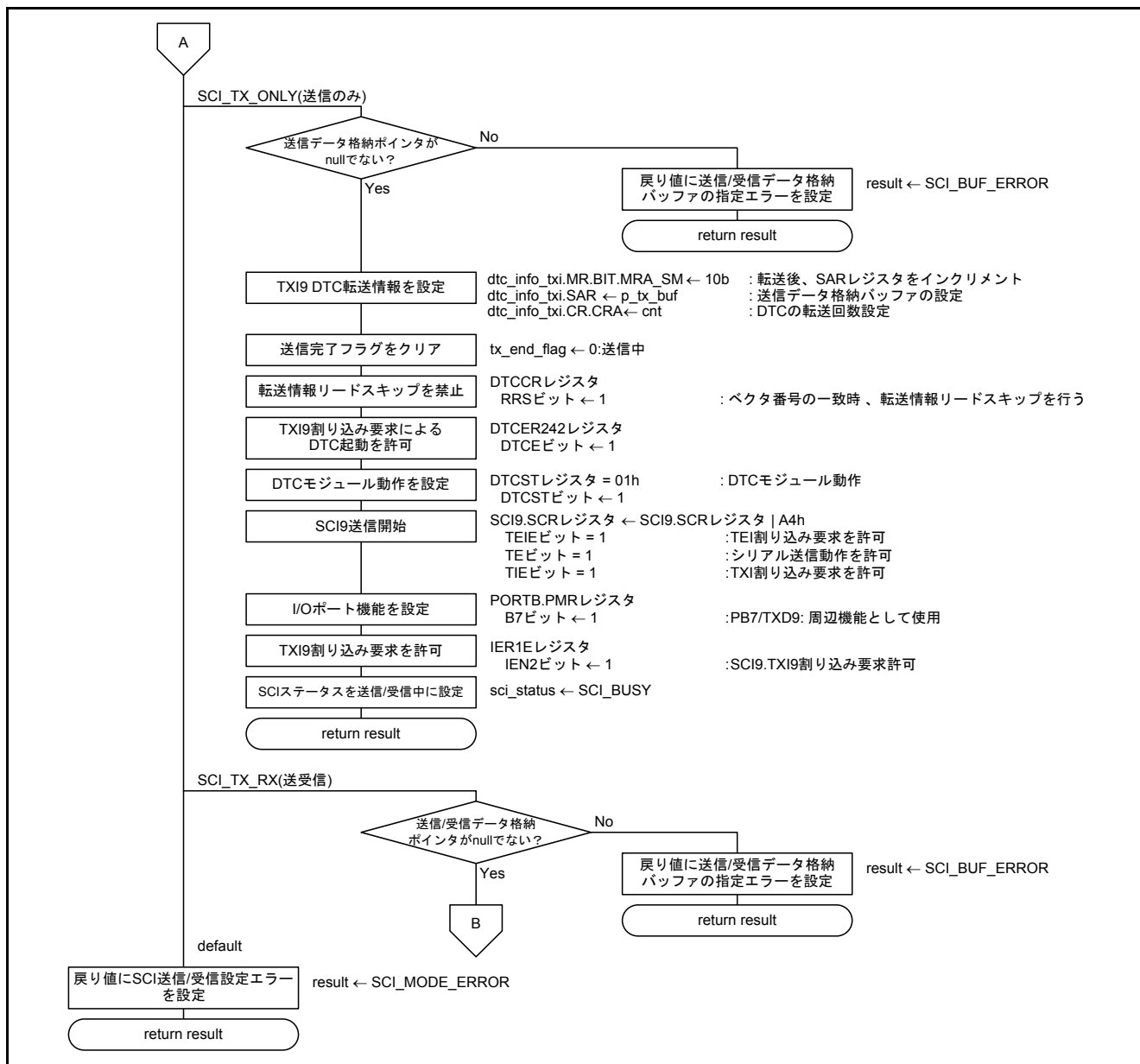
図5.13 SCI 送受信開始処理(2/3)
