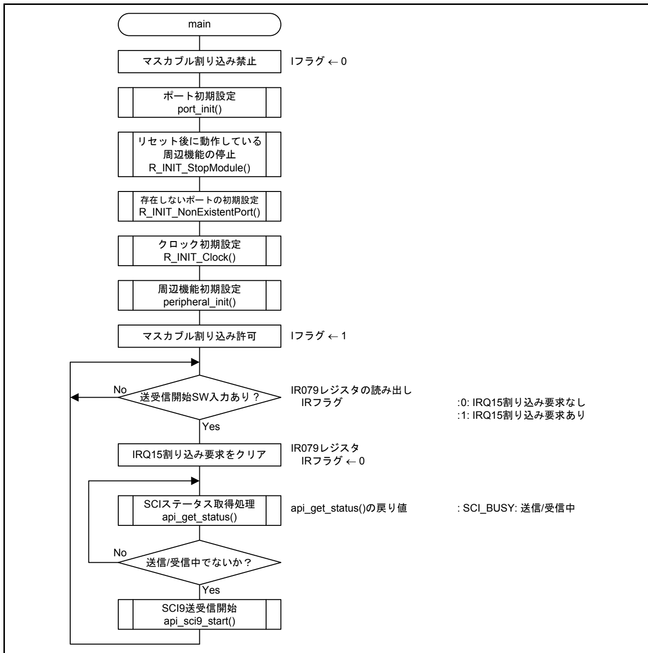
図5.4 メイン処理
