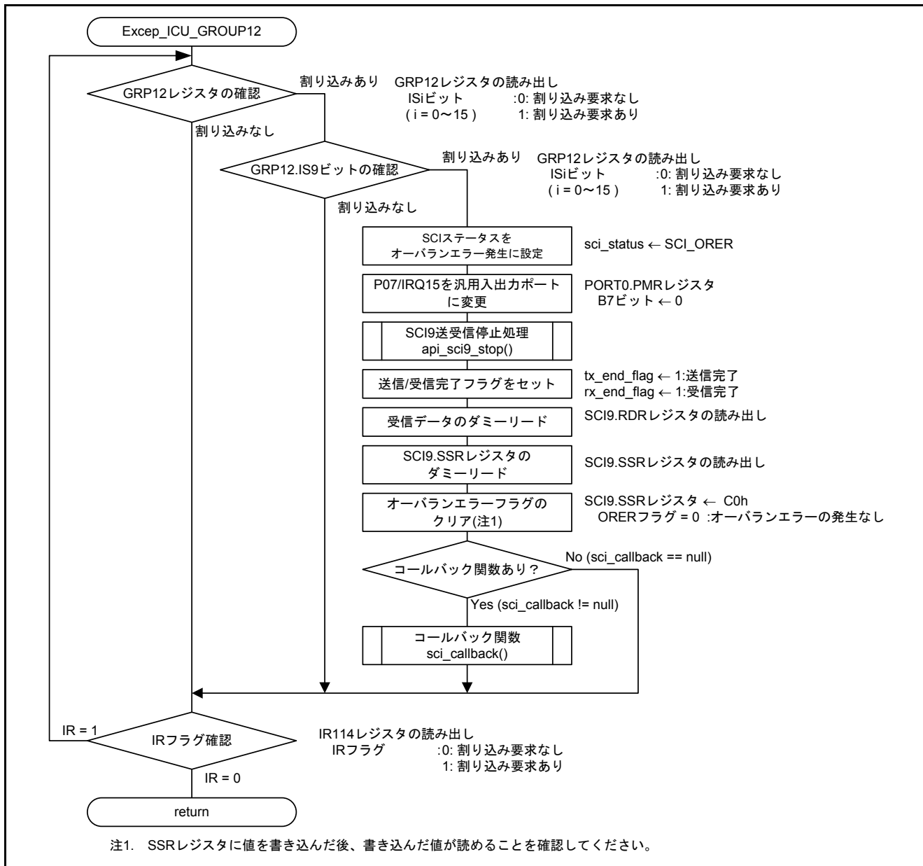
図5.20 GROUP12 割り込み(ERI9 割り込み)処理
