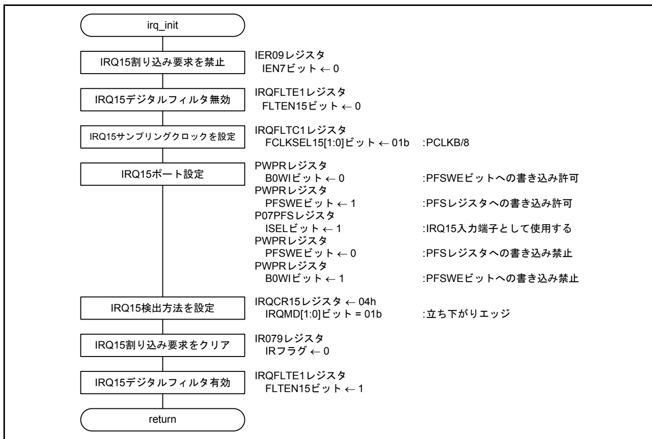
図5.7 IRQ 初期設定
