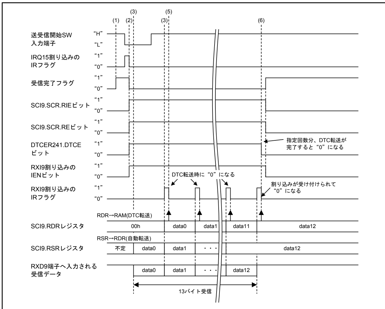
図5.2 受信動作のタイミング図
