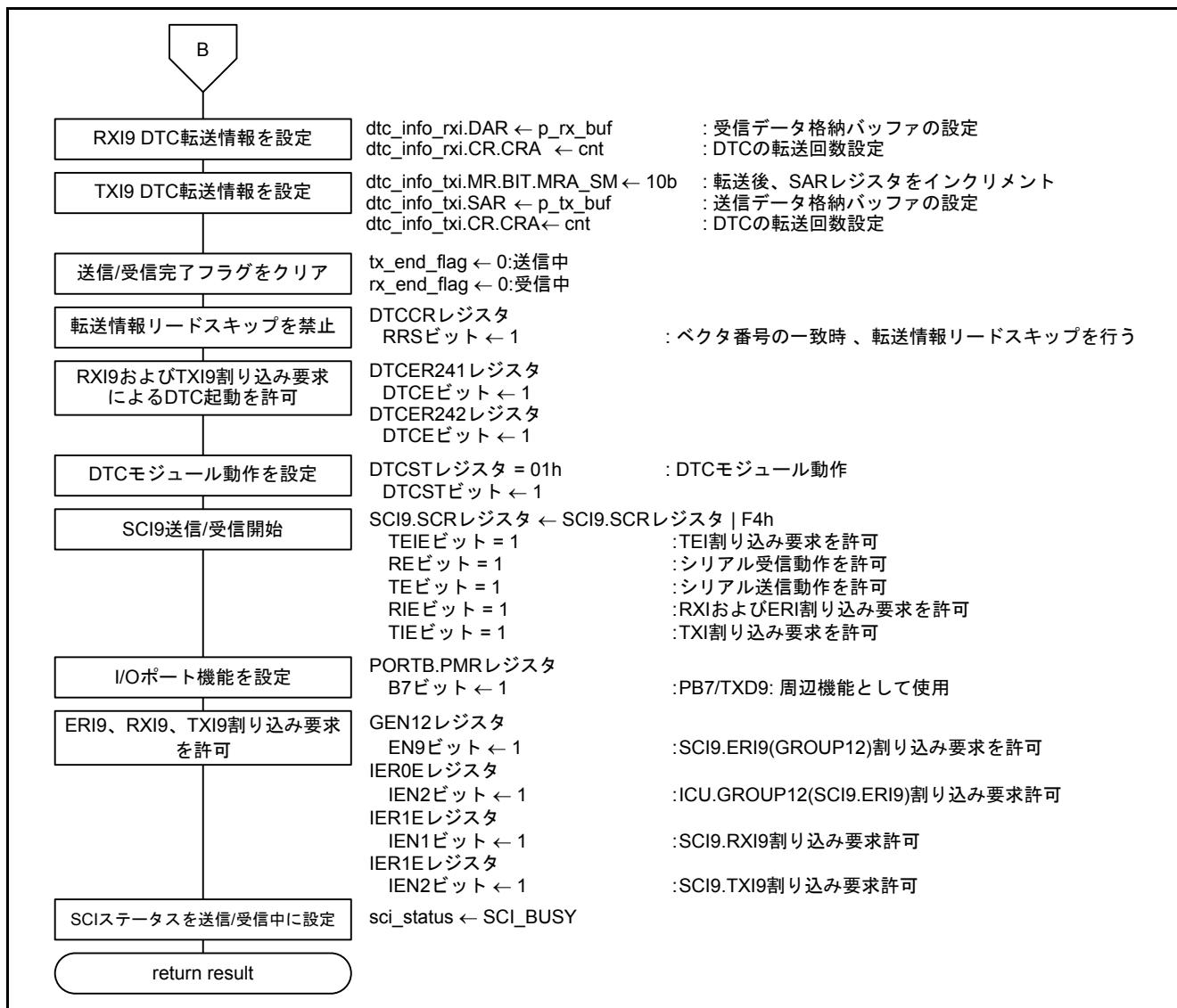
図5.14 SCI 送受信開始処理(3/3)
