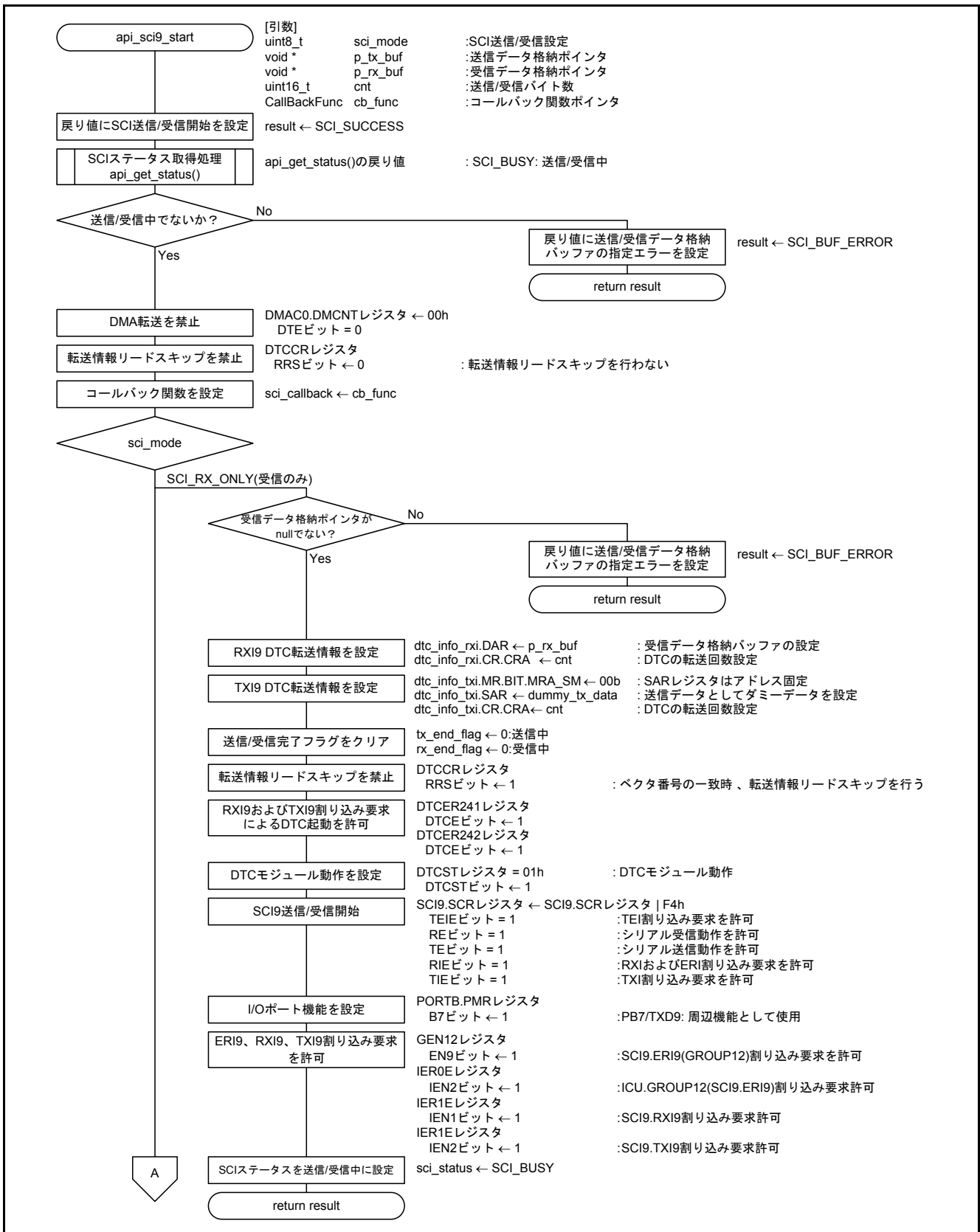
図5.12 SCI9 送受信開始処理(1/3)
