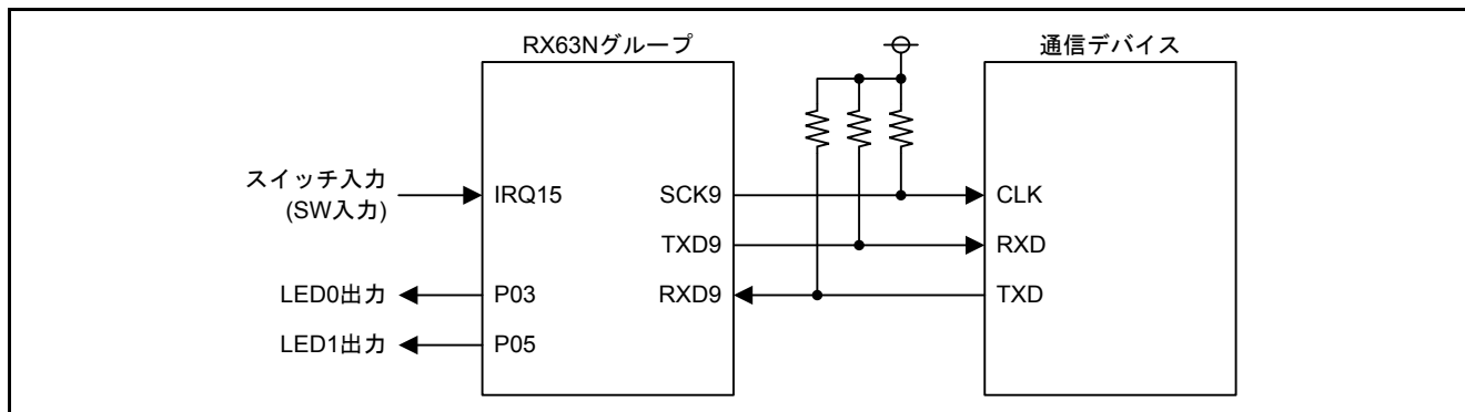
図4.1 接続例
