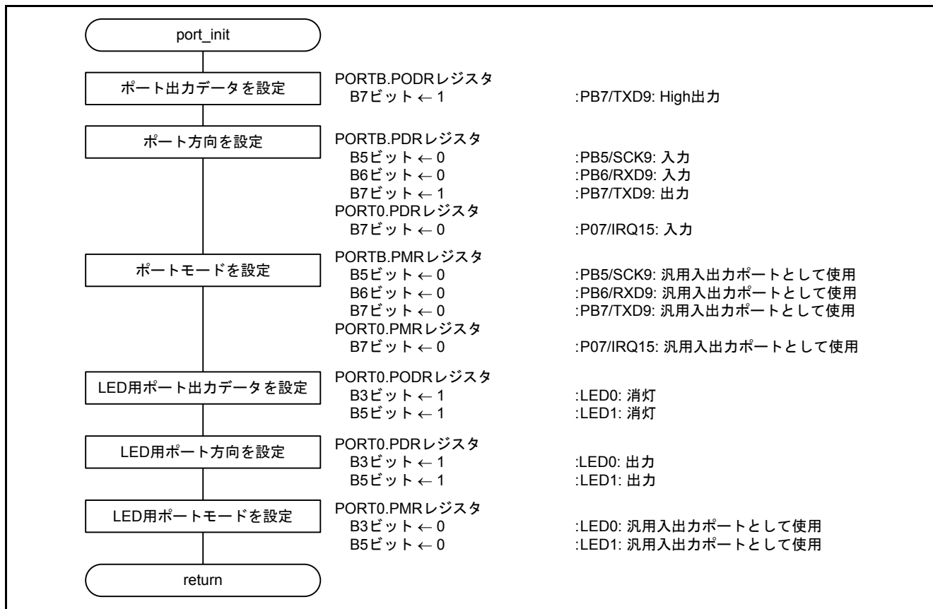
図5.5 ポート初期化処理
