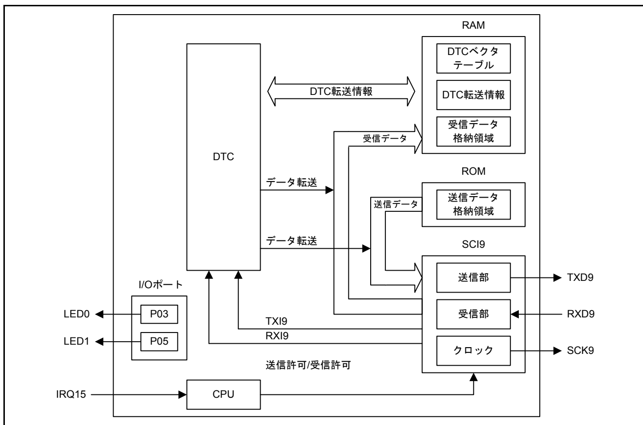
図1.1 ブロック図
