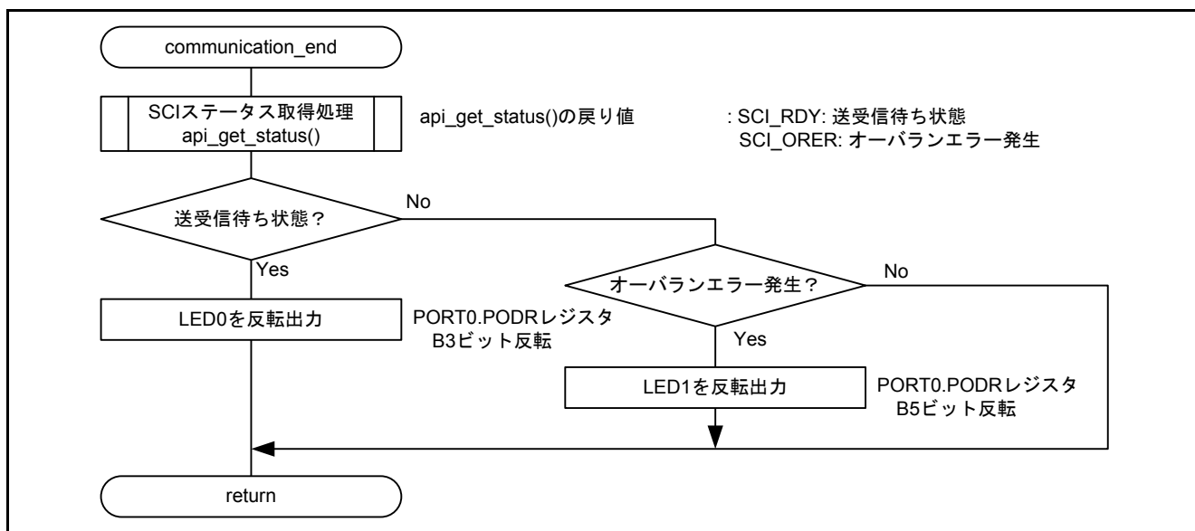
図5.8 送受信完了処理(コールバック関数)
