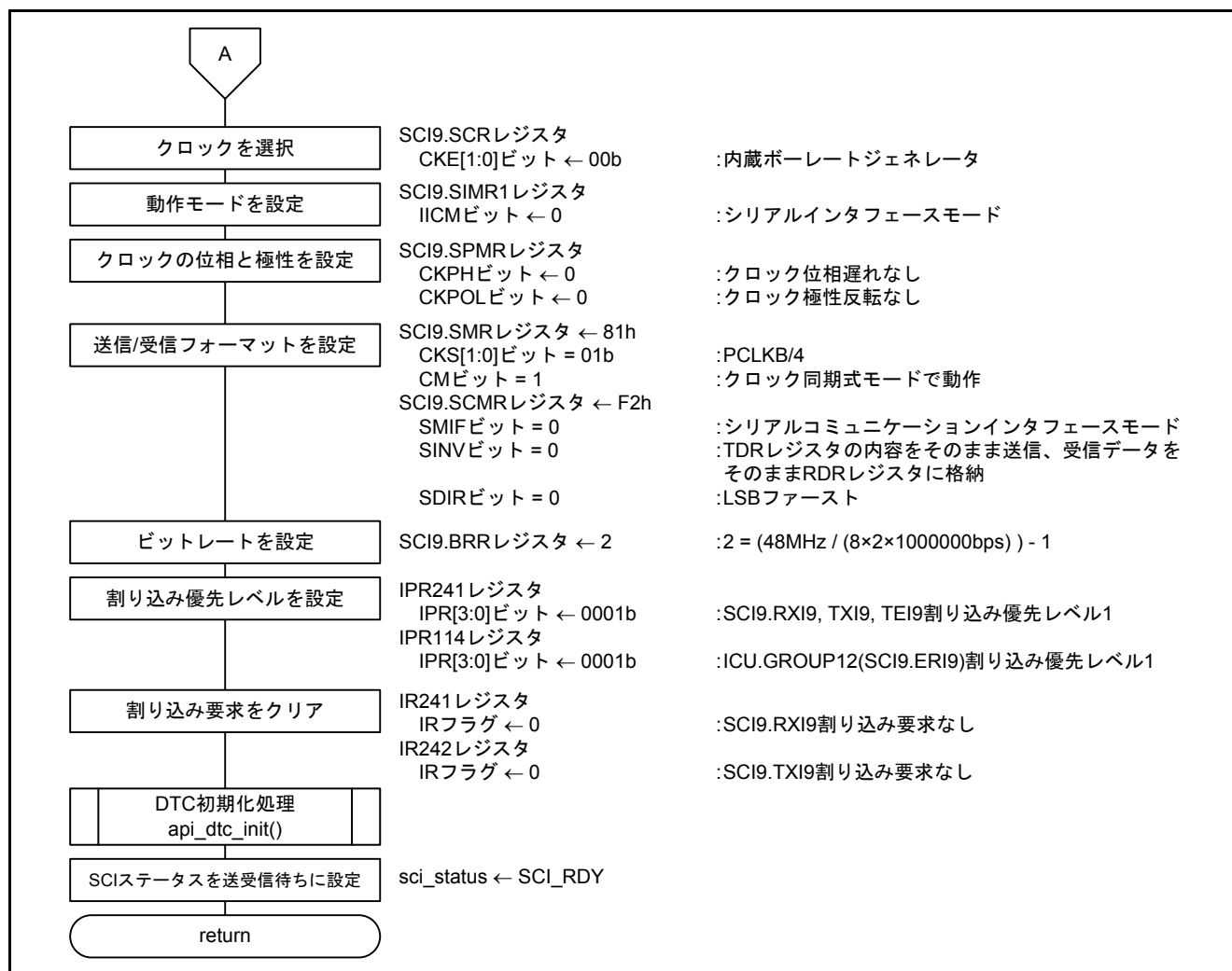
図5.10 SCI 初期設定(2/2)
