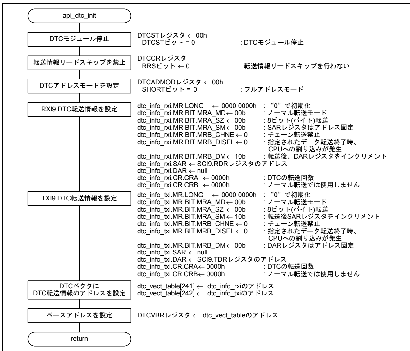
図5.11 DTC 初期設定
