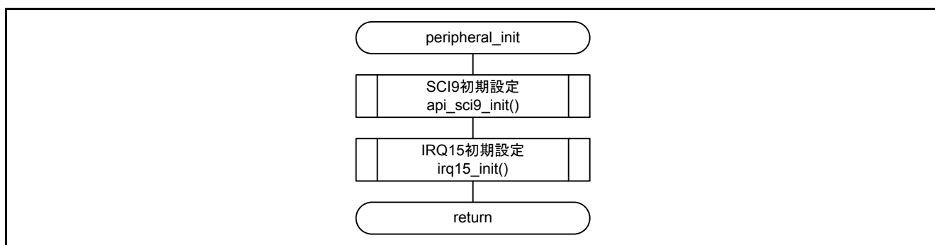
図5.6 周辺機能初期設定
