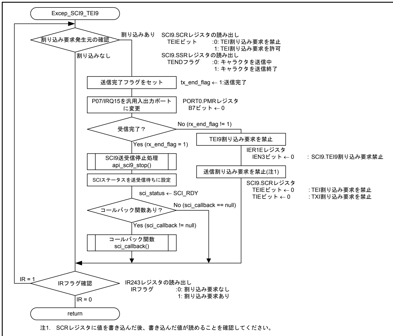
図5.19 TEI9 割り込み処理
