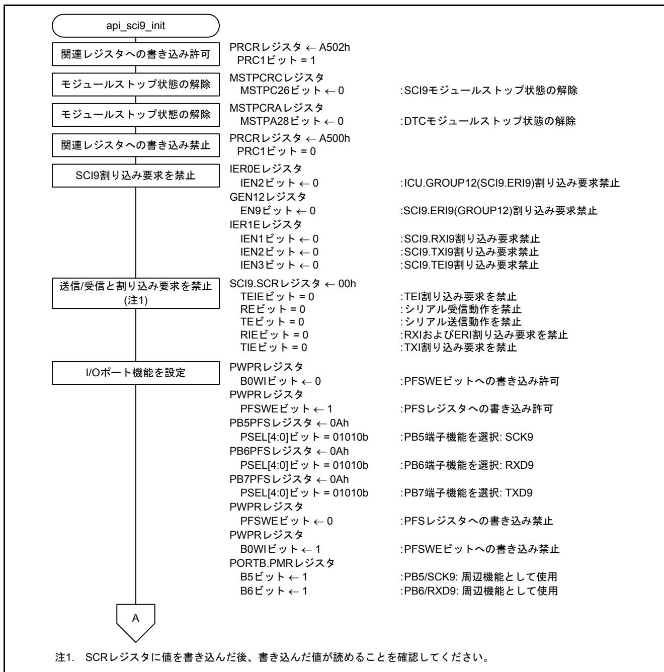
図5.9 SCI9 初期設定(1/2)
