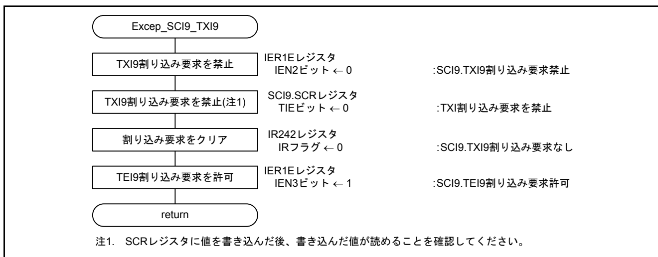
図5.18 TXI9 割り込み処理
