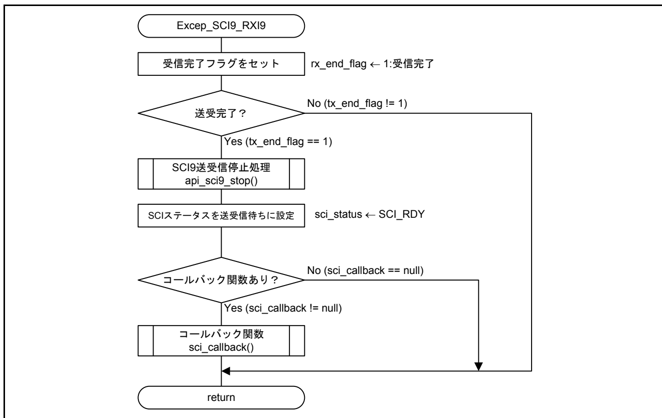
図5.17 RXI9 割り込み処理
