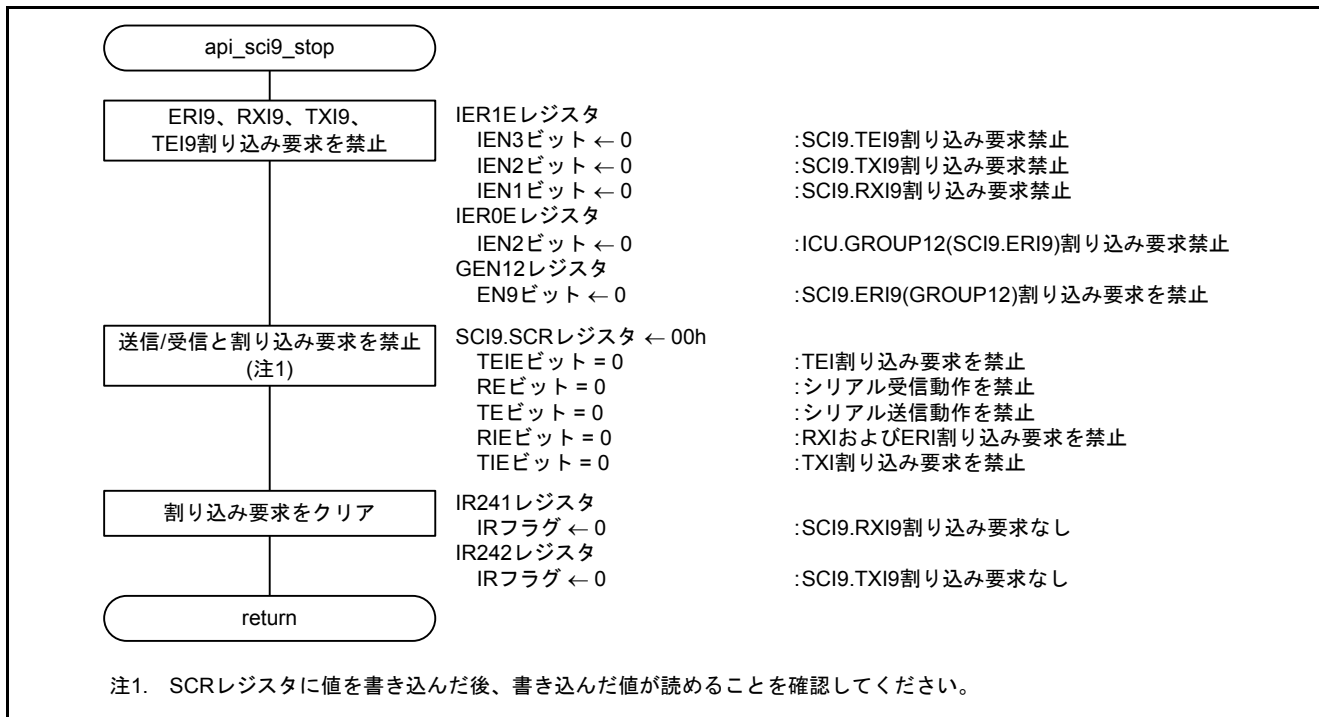
図5.15 SCI 送受信停止処理
