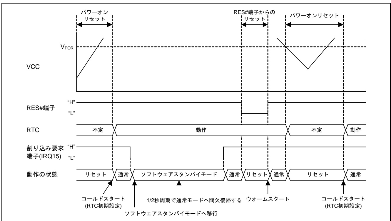
図1.1 動作概要
