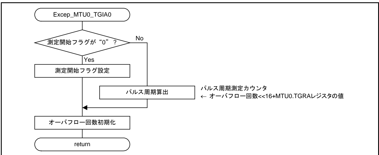
図5.8 MTU0 インพุットキャプチャ A 割り込み処理
