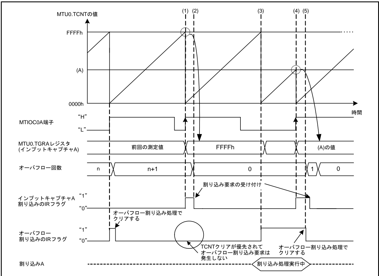
図5.2 インพุットキャプチャとオーバーフローが同時に発生したときのタイミング図
