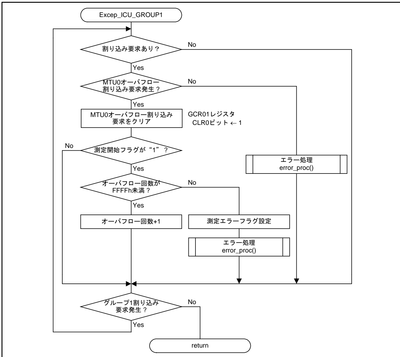
図5.9 MTU0 オーバフロー割り込み処理
