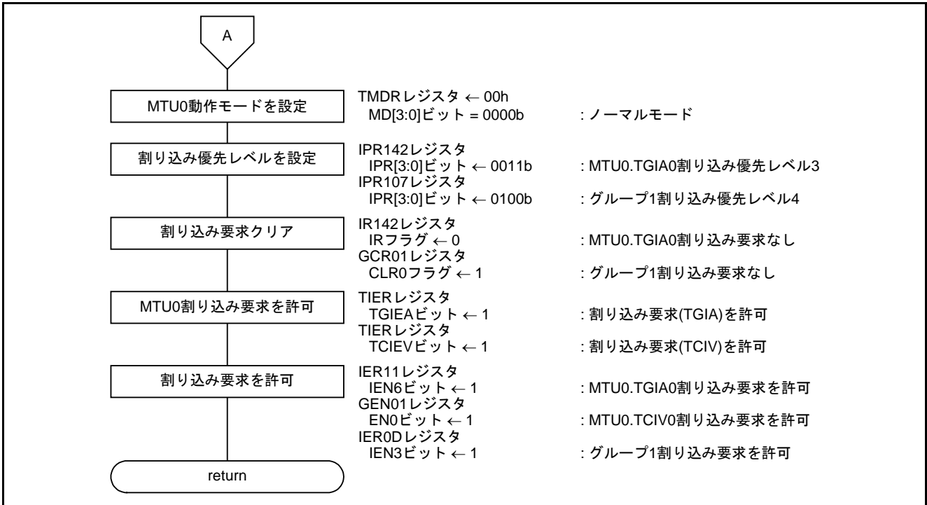
図5.6 周辺機能初期設定(2/2)
