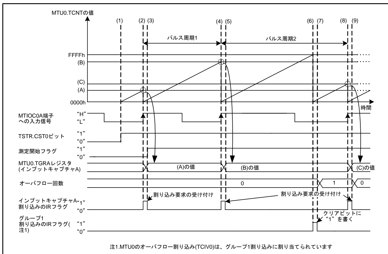
図5.1 パルス周期測定のタイミング図
