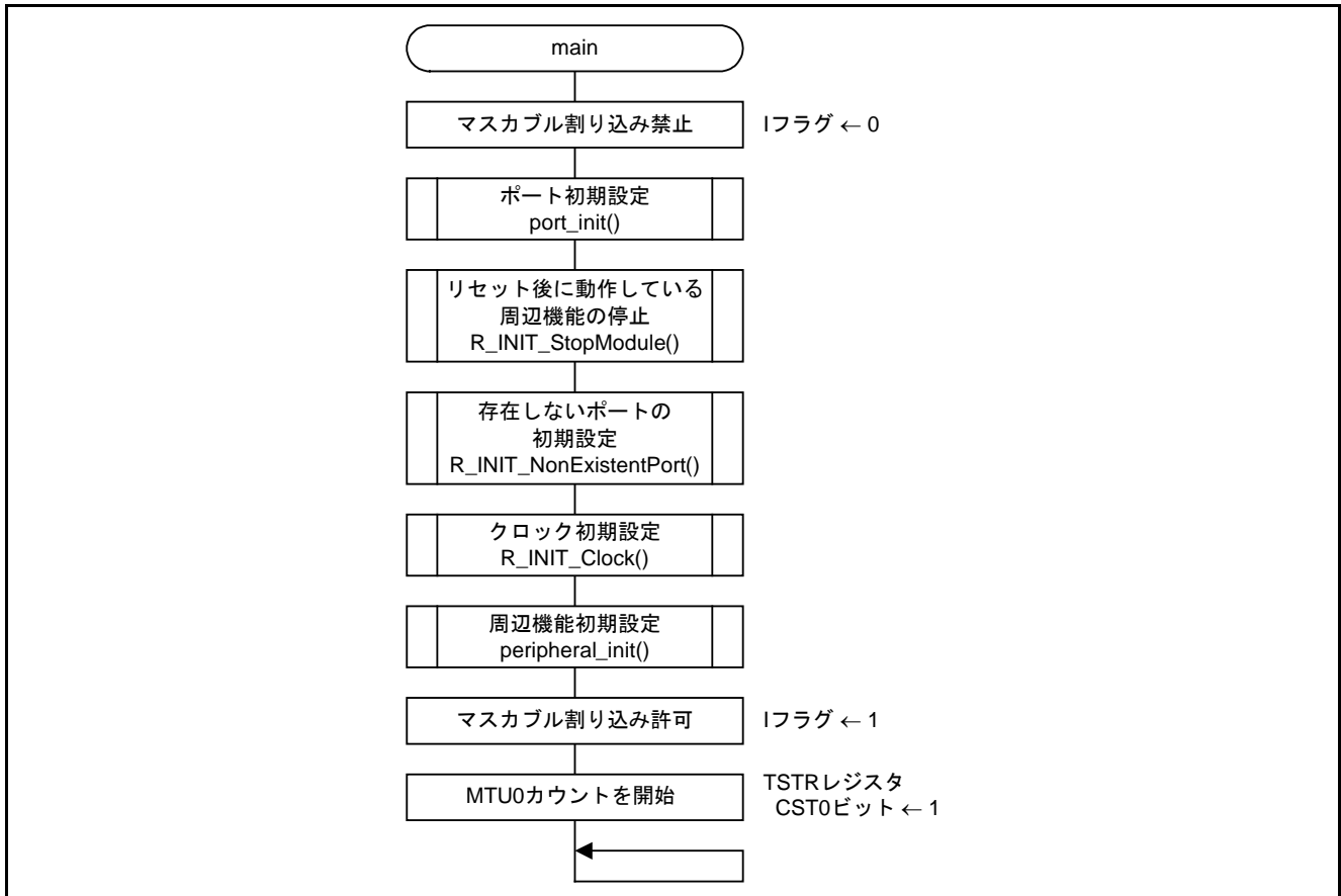
図5.3 メイン処理
