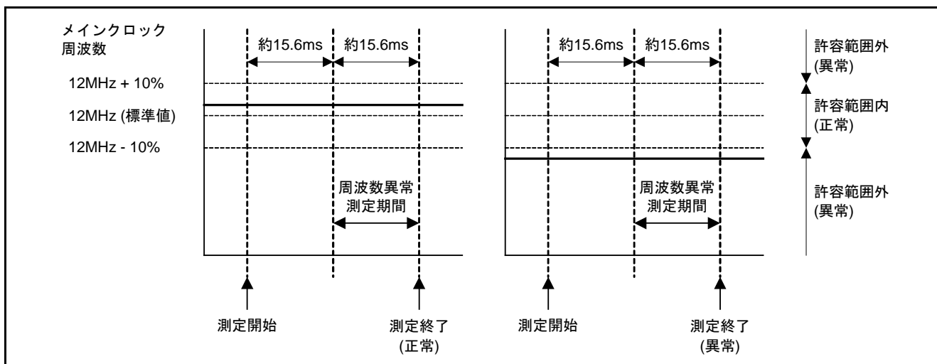
図 1.2 動作概要
