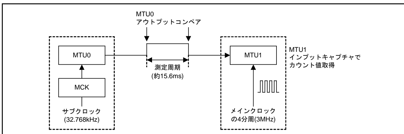
図 1.1 ブロック図
