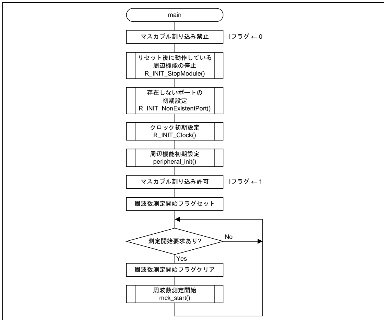
図4.2 メイン処理
