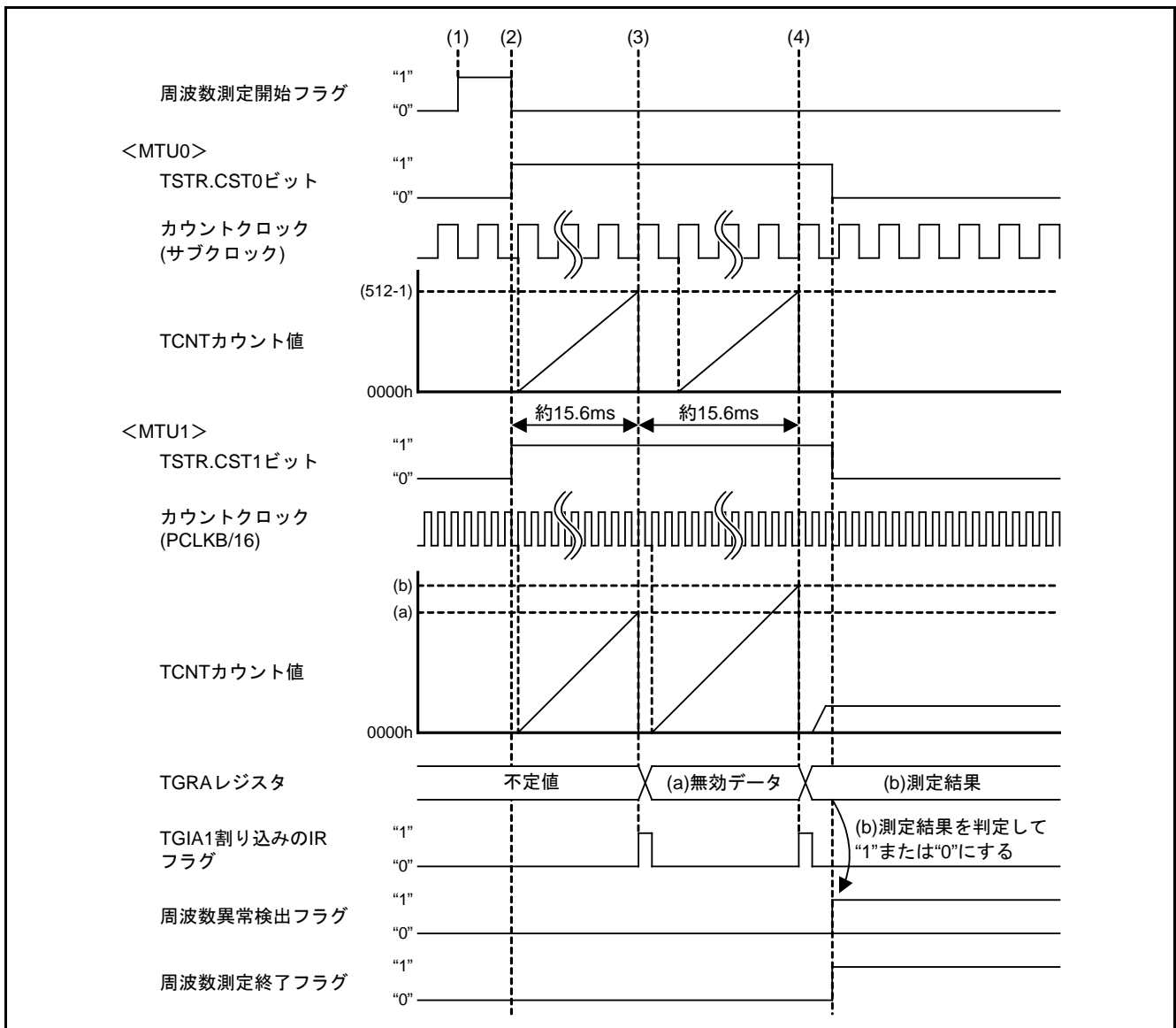
図4.1 タイミング図
