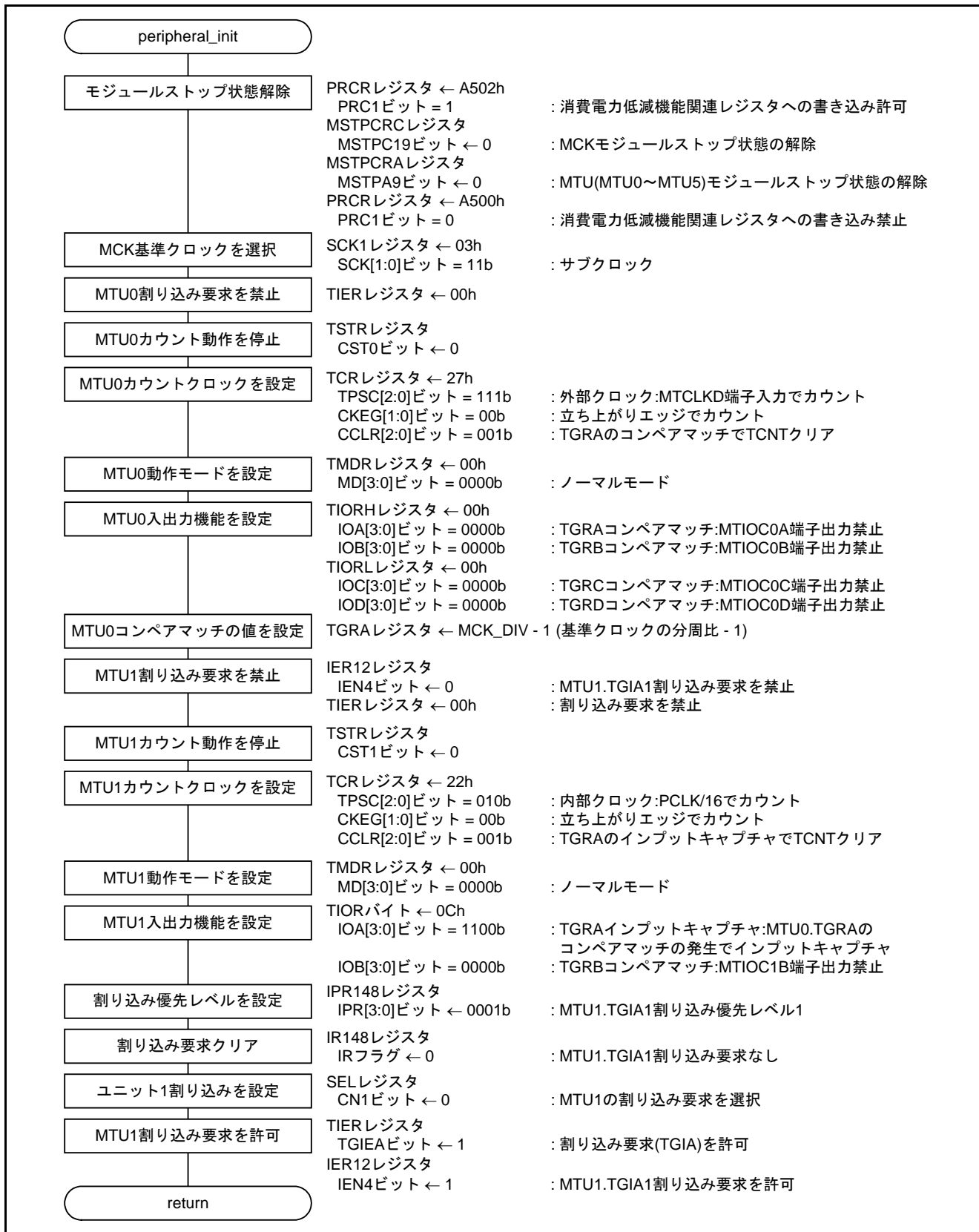
図4.3 周辺機能初期設定
