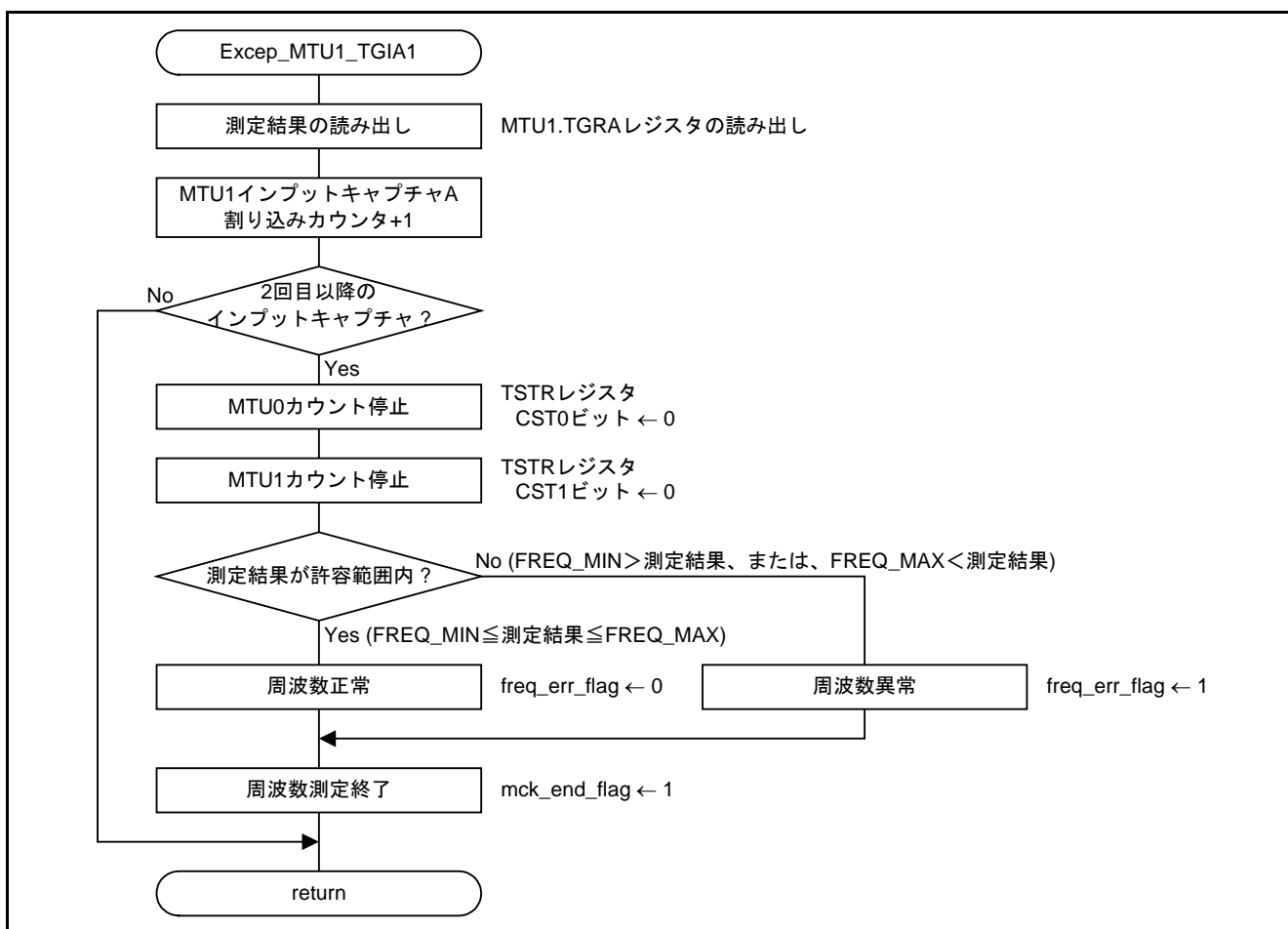
図4.5 MTU1 インプットキャプチャ A 割り込み処理
