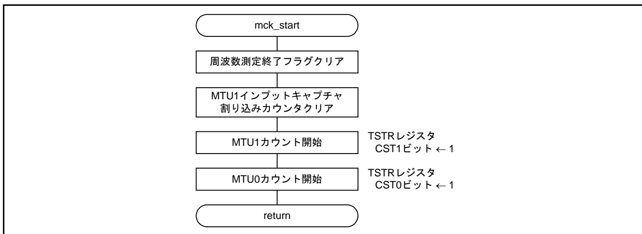
図4.4 周波数測定開始
