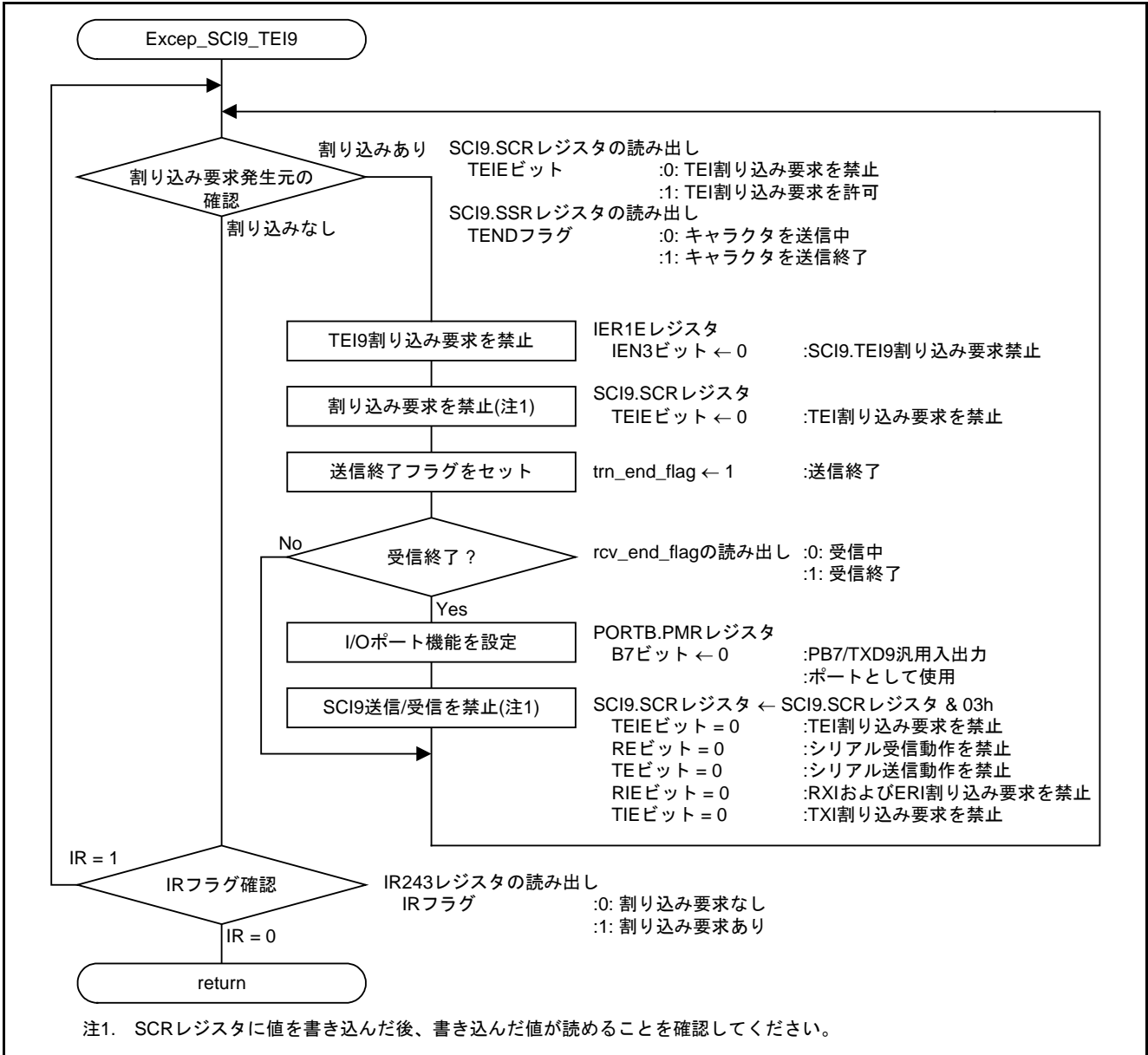
図5.12 SCI9 送信終了割り込み処理
