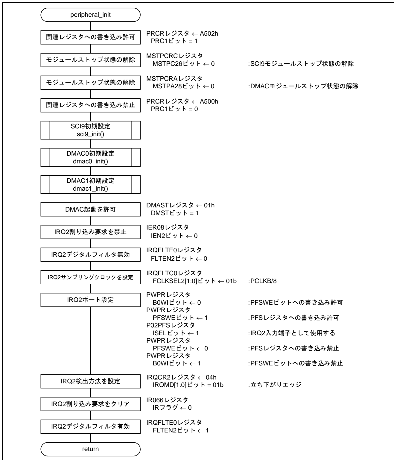
図5.5 周辺機能初期設定
