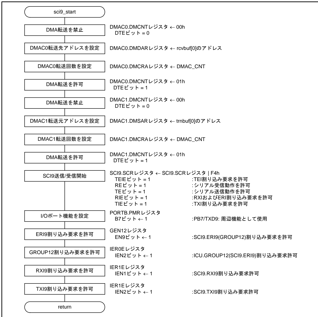
図5.9 SCI9 送受信開始
