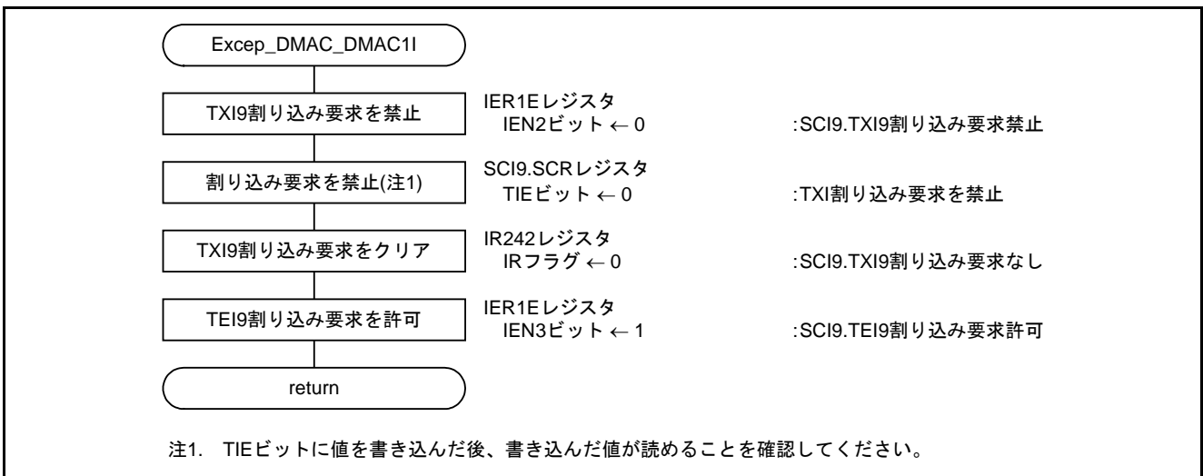
図5.11 DMAC1 転送終了割り込み処理
