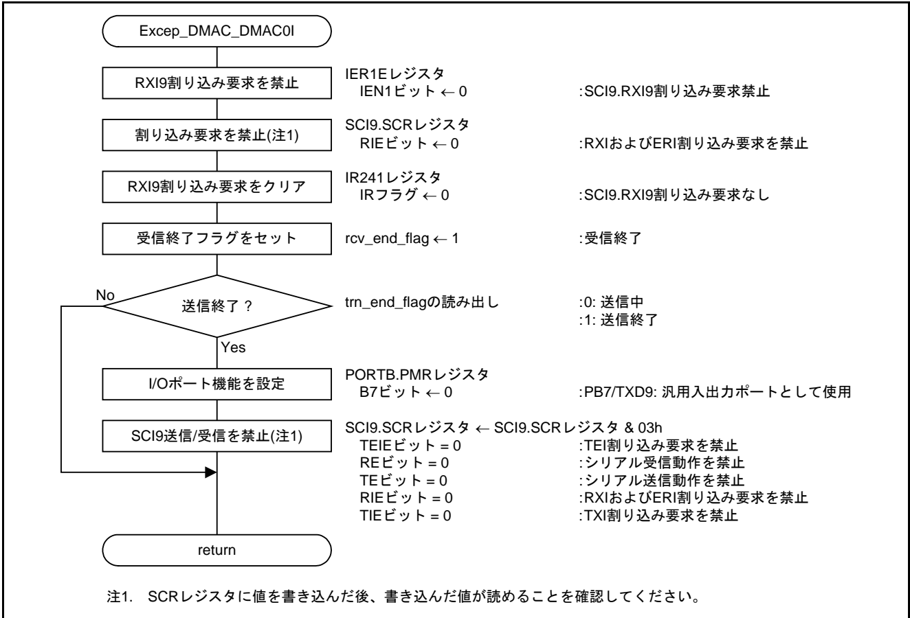
図5.10 DMAC0 転送終了割り込み処理
